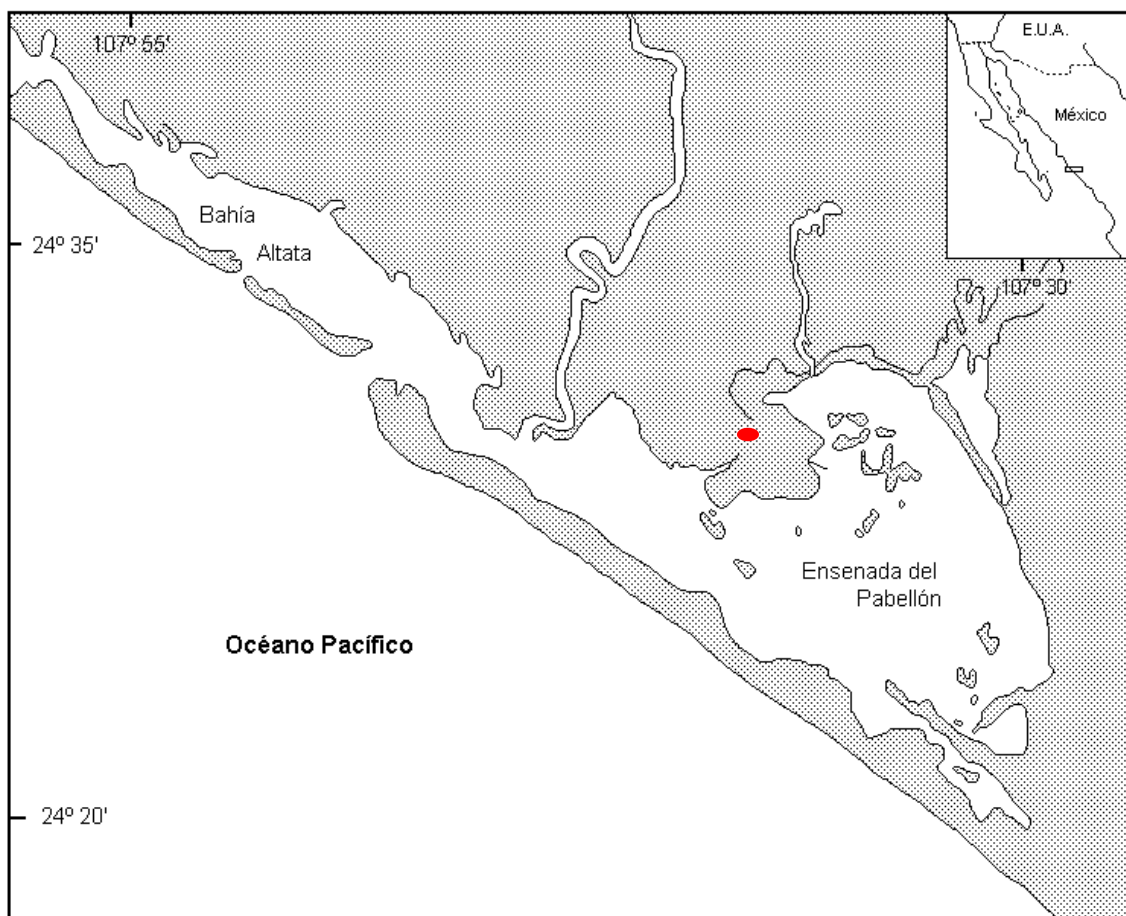
Imagen IV.11. Sistema ambiental del sitio del proyecto. Google earth.
