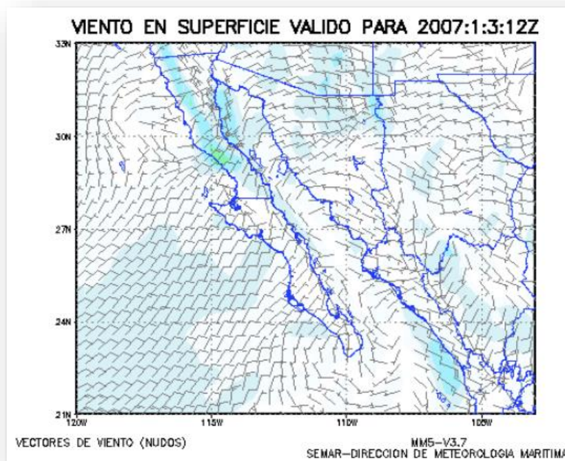
Figura 25. Vientos dominantes.
