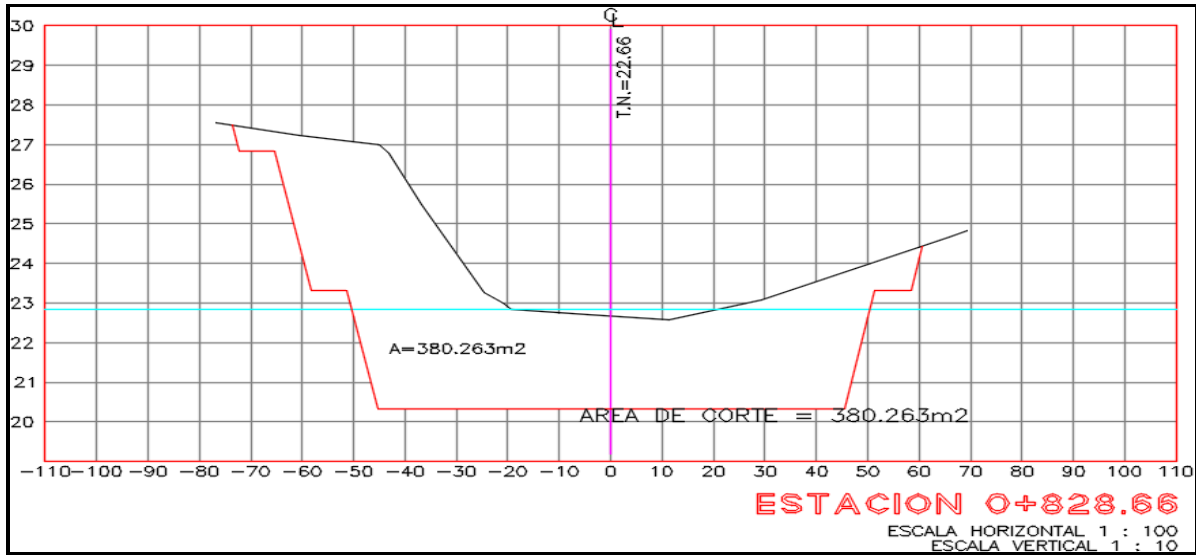
Figura 4.- ESTACION 0+828.66 (Parte final del proyecto):
