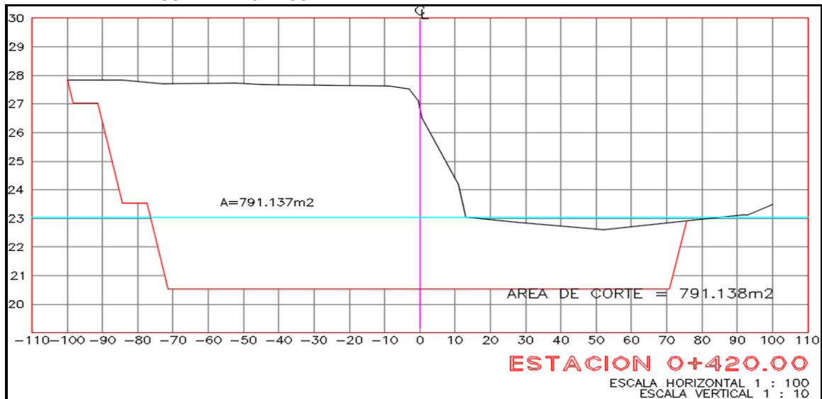
Figura 3.- ESTACION 0+420.000 (Parte central del proyecto):
