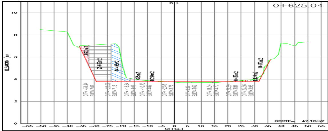
Figura 8.- ESTACION 0+625.04 (Aguas más arriba del proyecto): AREA DE TERRAPLEN = 0.000 m 2 AREA DE CORTE = 47.18 m 2
