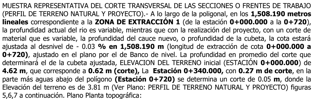
ESTACION ELEVACION TERR. NAT. ELEVACION PROYECTO NIVEL DE AGUA ESPESES TERRAPLEN ESPESES CORTE 0+000 4.62 4.00 5.40 0.62 0+100 4.39 3.98 5.49 0.59 0+140 4.08 3.98 5.49 0.59 0+160 3.98 3.98 5.48 0.00 0.00 0+180 3.96 3.97 5.47 0.02 0+195.54 3.97 3.97 5.47 0.00 0.00 0+100 3.97 3.97 5.47 0.00 0.00 0+120 3.97 3.96 5.46 0.01 0+140 3.97 3.95 5.45 0.01 0+160 4.21 3.95 5.45 0.26 0+180 4.86 3.94 5.44 0.94 0+200 4.80 3.93 5.43 0.87 0+220 4.66 3.93 5.43 0.73
