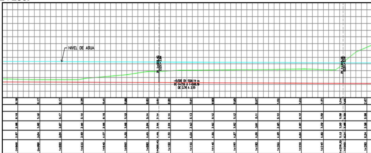
Figura 12.- Muestra representativa de corte transversal, de la estación 0+960 a la estación 1+280 .
