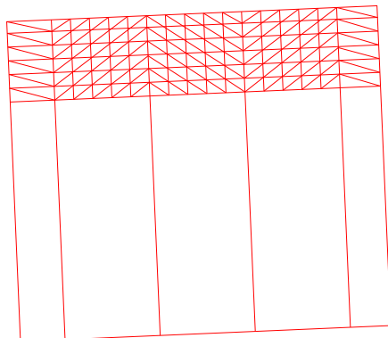
Ilustración 11.- Diseño de excluidor de fauna acuática en cárcamo de bombeo 1.
