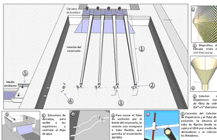
Ilustración 73.- Sistemas de exclusión de fauna acuática (SEFA).
