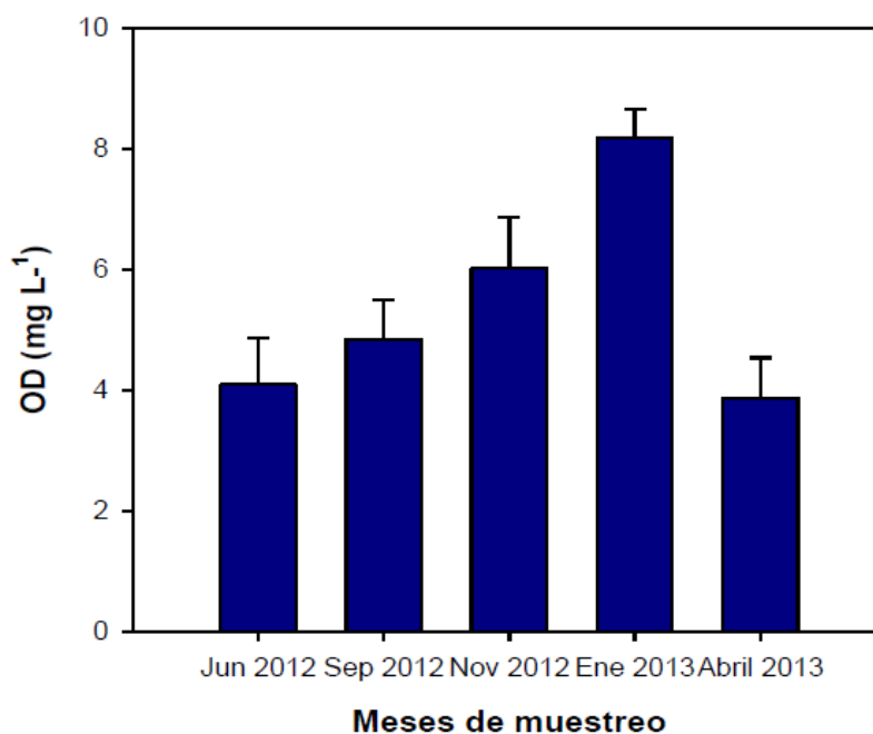
Ilustración 34.- Oxígeno disuelto (mg L -1 ) promedio en el Sistema Lagunar Navachiste registrado en los diferentes meses de muestreo.
