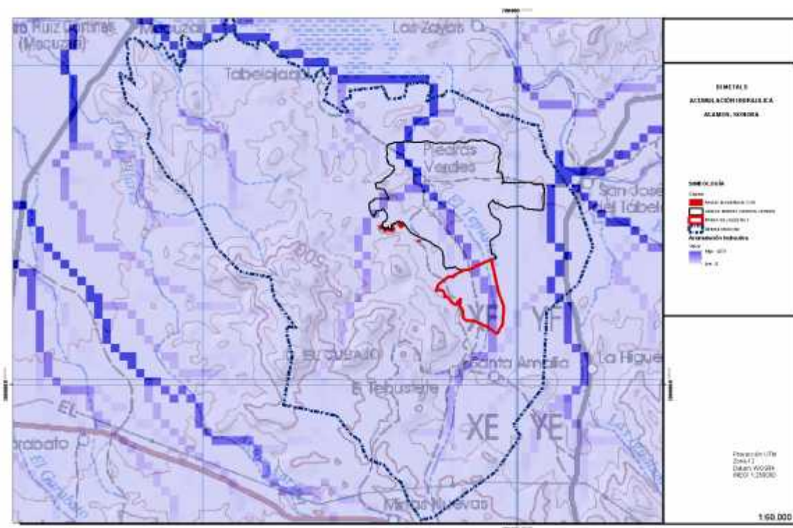
Figura IV.11. Hidrología del área del Proyecto Cerro Chato.
