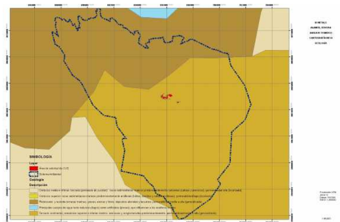
Figura IV.6. Geología del sistema ambiental definido para el Proyecto.
