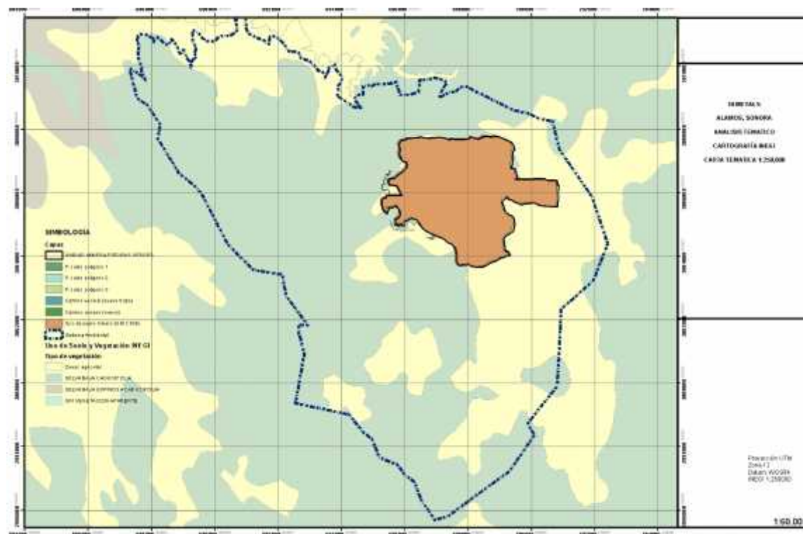
Figura IV.12. Tipo de vegetación presente en el Sistema Ambiental definido para el proyecto Cerro Chato.
