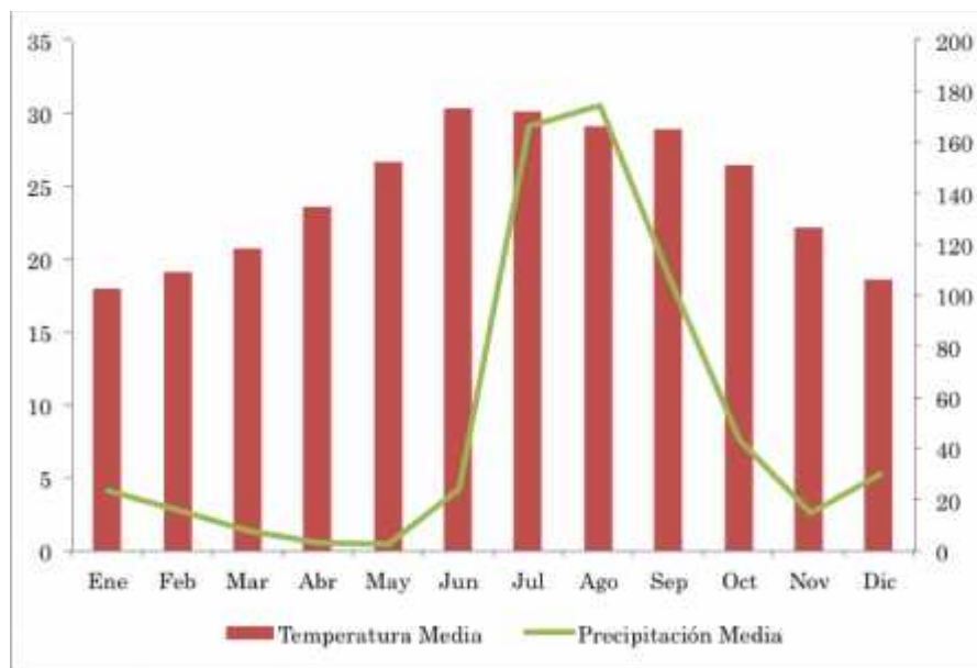
Figura IV.4. Climograma del sistema ambiental definido para el proyecto Operación de tajo y tepetatera 2 Segunda Etapa.
