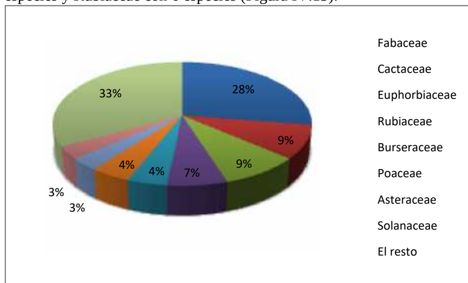
Figura IV.13. Porcentaje de especies de flora por familia en el sistema ambiental definido para el Proyecto.
