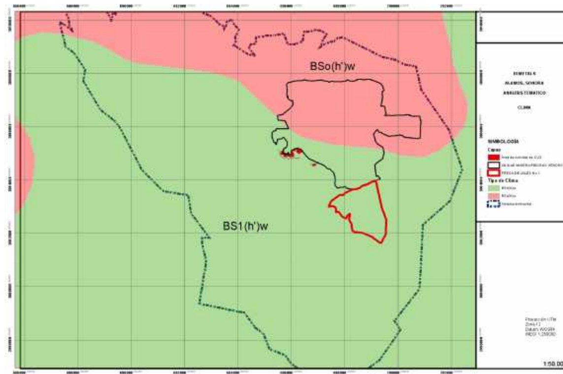
Figura IV.3. Tipos climáticos presentes en el Sistema Ambiental y en el área de Proyecto
