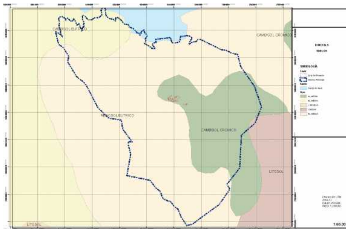
Figura IV.10. Suelos del Sistema Ambiental definido para el Proyecto.
