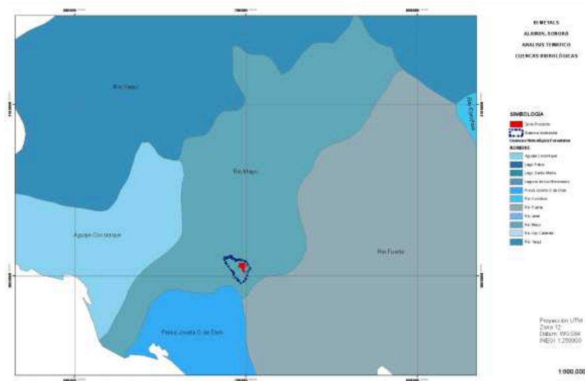
Figura IV.1 Ubicación de la cuenca hidrológica donde se ubica el proyecto (CONAGUA, 2009).
