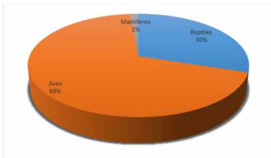
Figura IV.19. Porcentaje de abundancia por grupo registrada en el sistema ambiental definido para el Proyecto.
