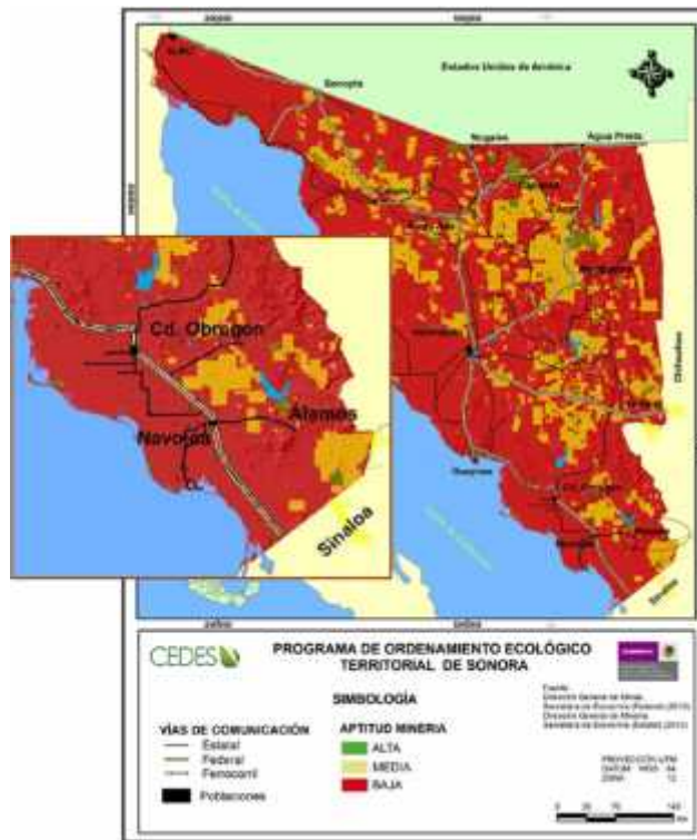
Figura III.2. Aptitud minera del estado de Sonora y de la Región de Álamos.
