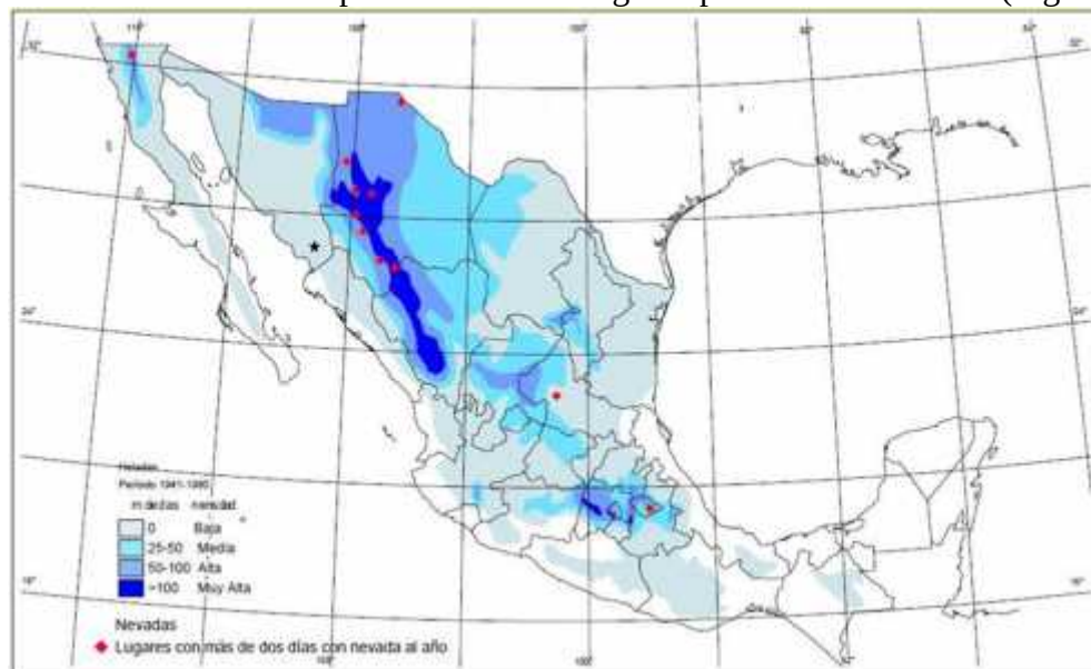
Figura IV.5. Registro de heladas en la república mexicana.
