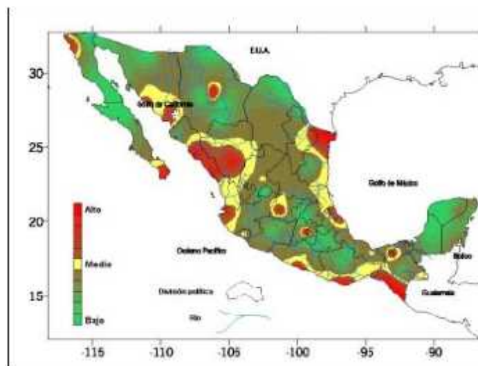
Figura IV.29. Ubicación del área de Proyecto respecto a Zonas con Peligro de inundaciones.
