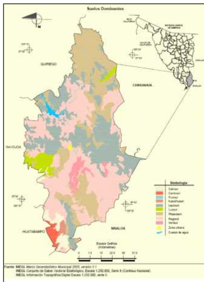
Figura IV.9. Tipos de suelo en el municipio de Álamos, Sonora.
