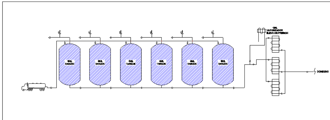
Figura II- 20. Arreglo tipo general de la estación de suministro de GNL.
