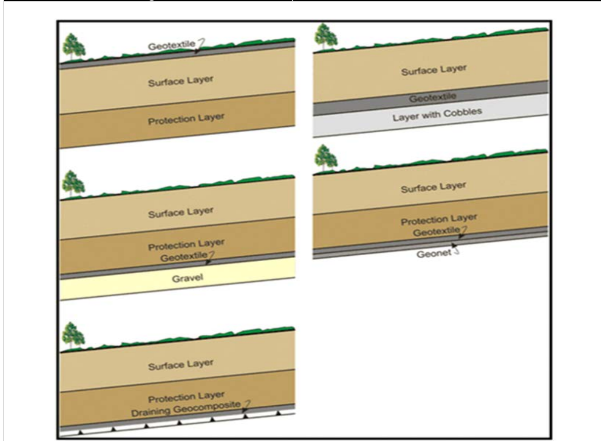
Figura II- 3. Diferentes esquemas de cubiertas sintéticas.
