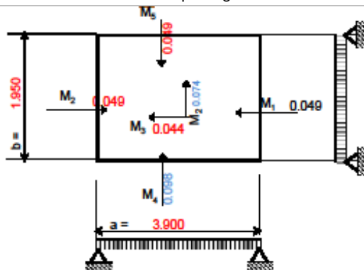
Diagrama de la losa tapa Tablero I Croquis M5
