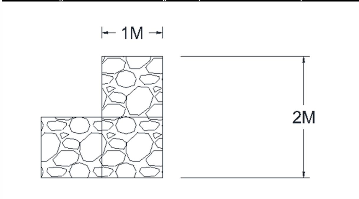
Figura II- 13. Detalle del muro de gaviones tepetatera 1 del socavón 3 de mayo.
