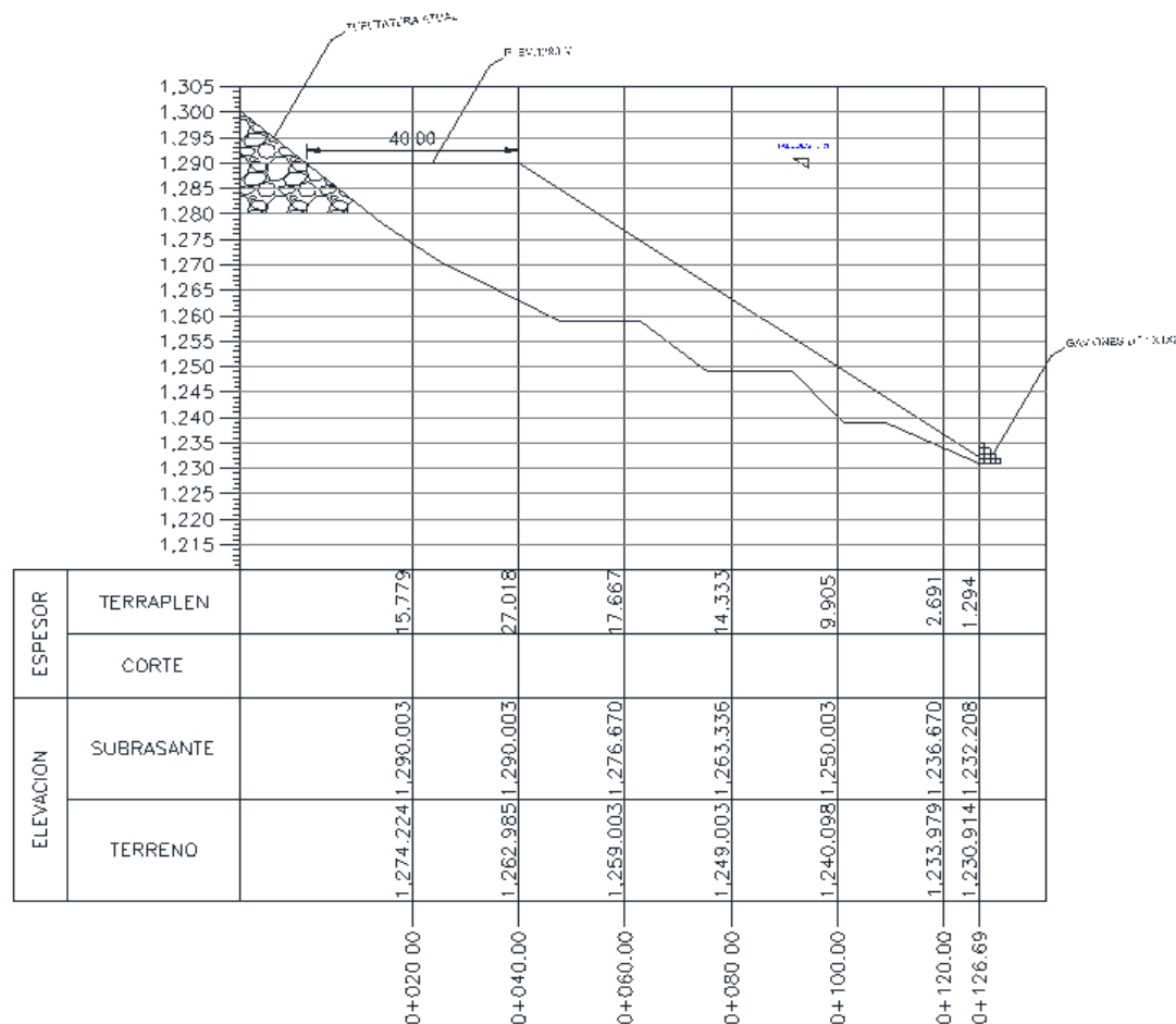
Figura II- 10. Perfil geométrico del depósito superficial de tepetate Nivel 23.
