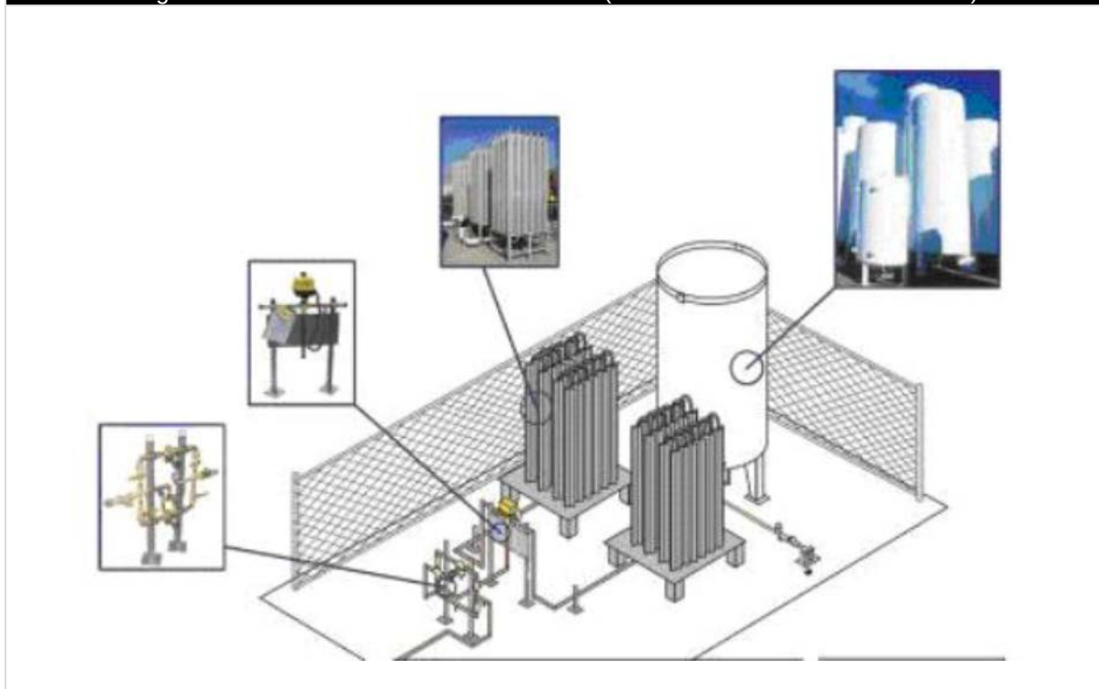
Figura II- 21. Estación de abastecimiento GNL (Fuente NOM-013-SECRE-2012 Secc 119)
