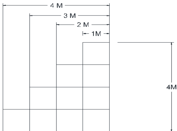
Figura II- 11. Detalle del muro de gaviones nivel 23.
