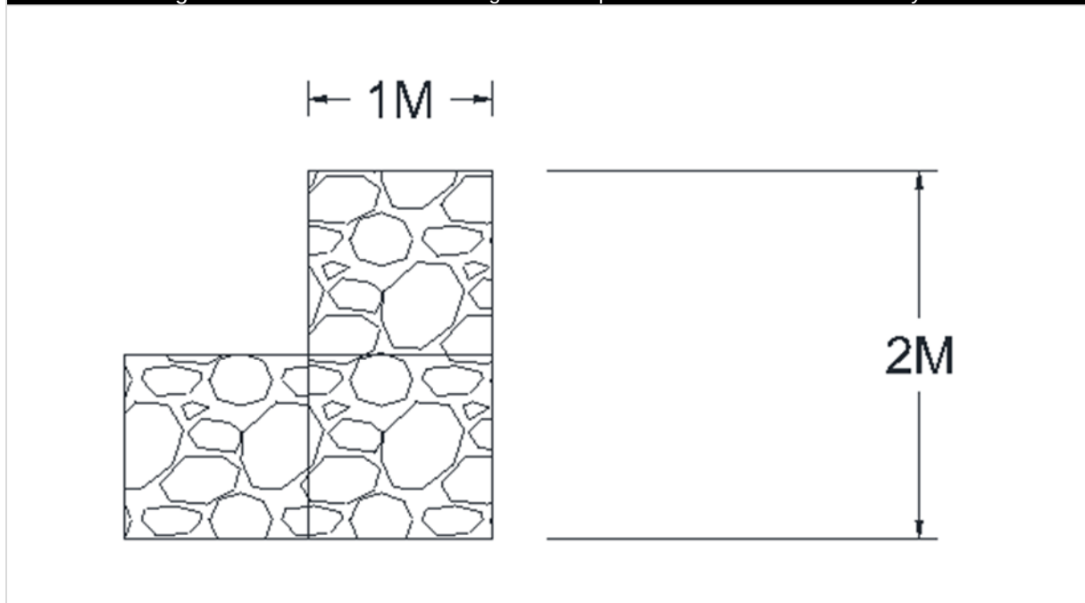
Figura II- 15. Detalle del muro de gaviones tepetatera 2 del socavón 3 de mayo.
