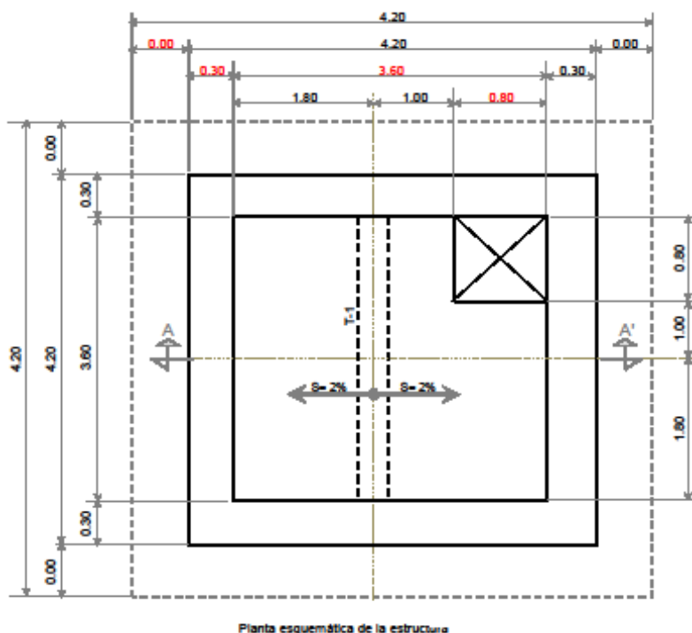
Figura II- 16. Croquis esquemático de la estructura TCR.
