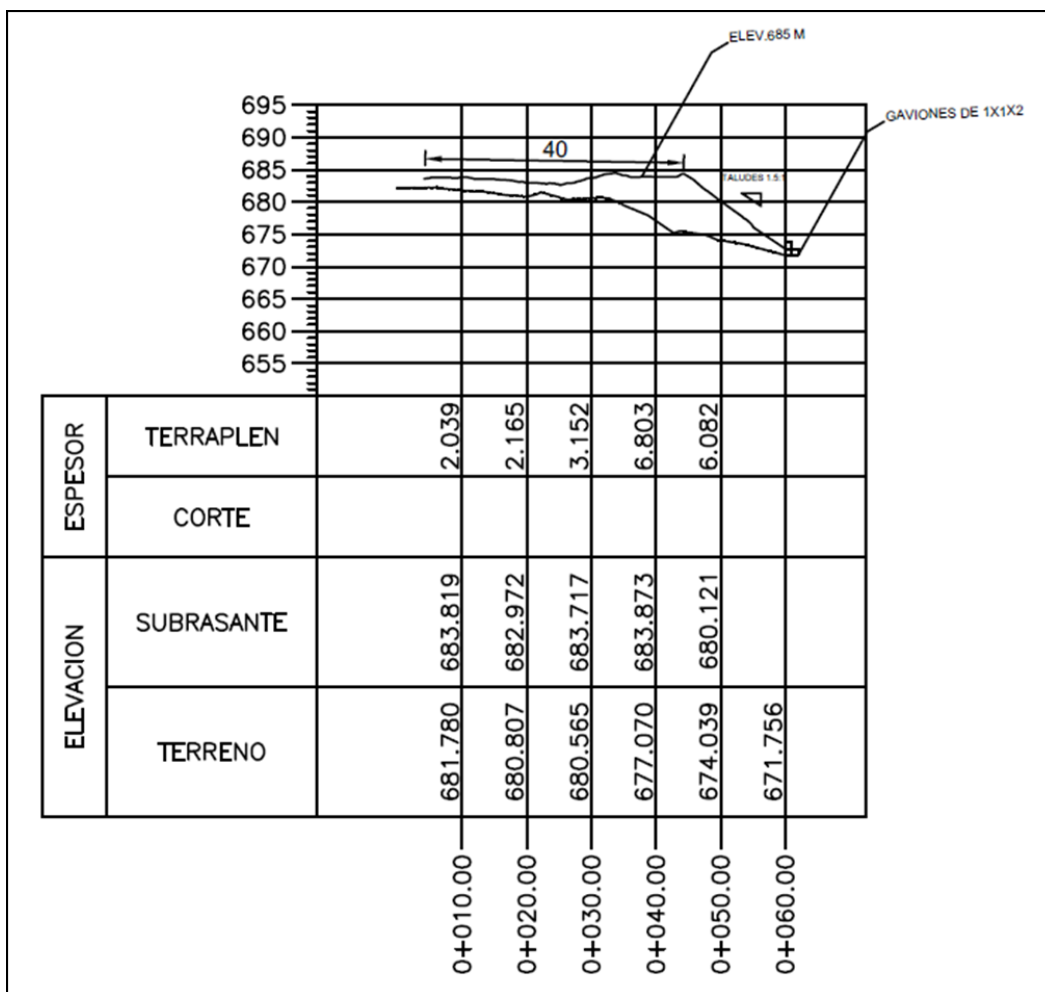
Figura II- 12. Perfil geométrico del depósito superficial de tepetate 1 del socavón 3 de mayo.
