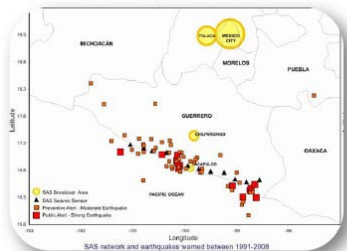
Imagen 25 Estaciones permanentes del Sistema de alerta sísmica
