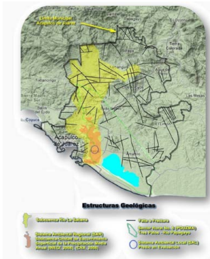
Imagen 22 Fallas y fracturamiento
