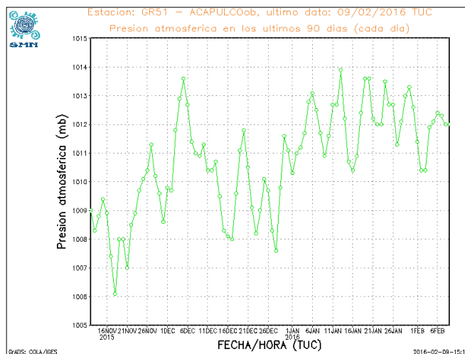
Imagen 17 Presión atmosférica en 90 días
