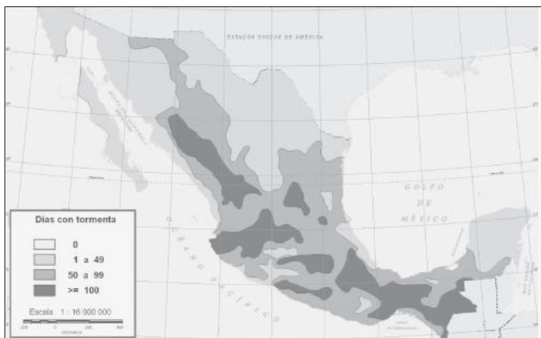
Imagen 18 Máximo anual de días con tormenta eléctrica en México. FUENTE: CENAPREV, SEGOB. 2010
