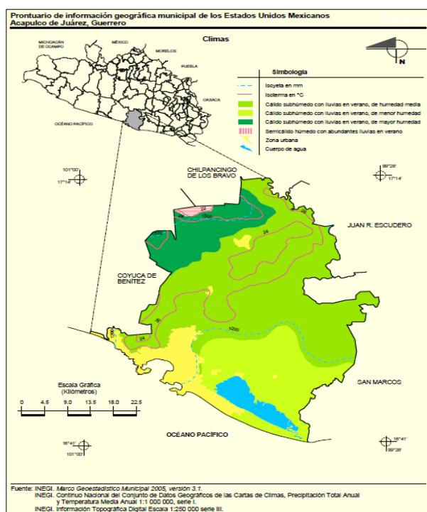
Imagen 13 Clima del municipio de Acapulco. FUENTE INEGI
