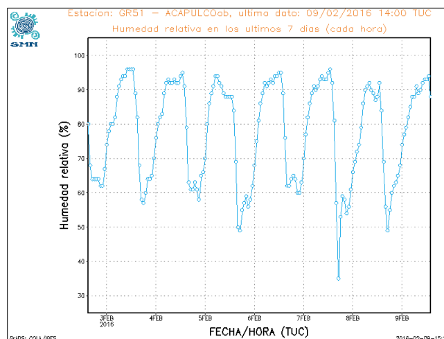
Imagen 16 Humedad relativa en 7 días.
