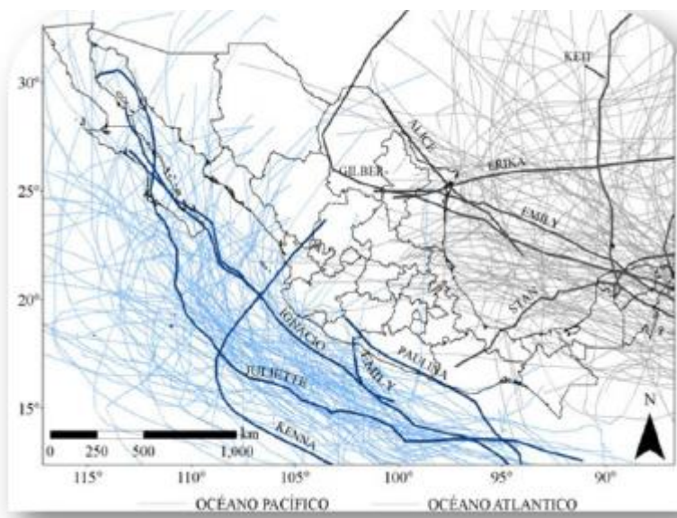
Imagen 20 Ruta de huracanes
