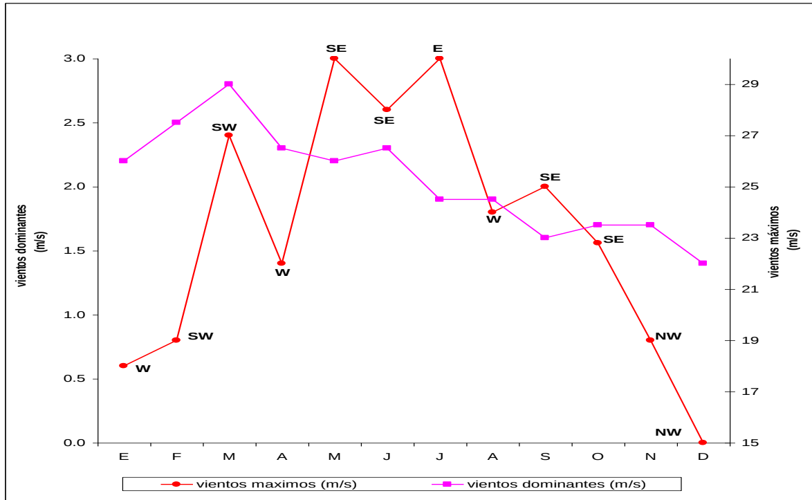
Imagen IV.4. Vientos dominantes.
