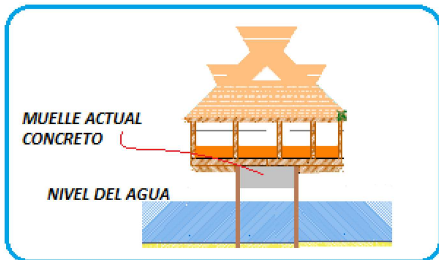
Diagrama de Corte del muelle y el Gazebo de forma volada sin pilotes extras.
