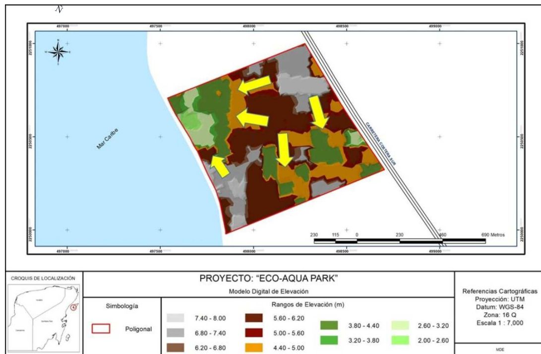
Plano No. 12 Modelo digital de elevación del predio elaborado a partir de curvas de nivel levantadas en el predio.
