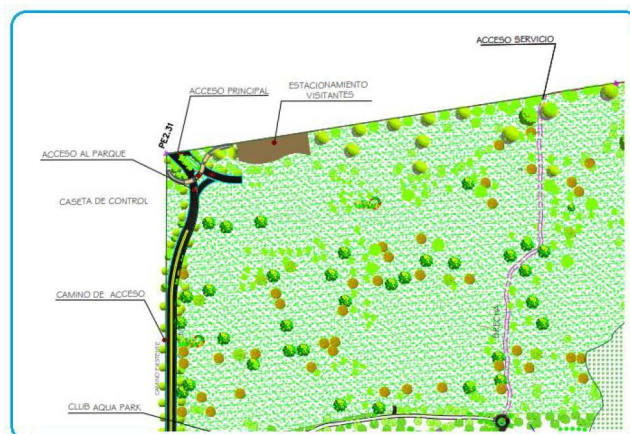
Diagrama extracto del plan maestro(plano 009), indicando el acceso al proyecto
