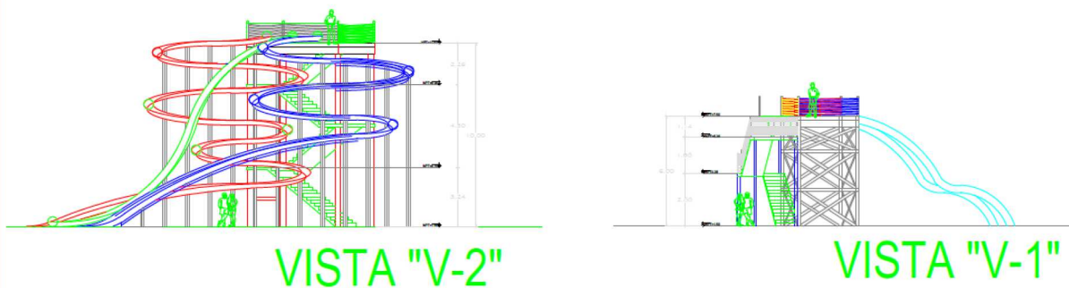
Diagramas de los alzados de los toboganes
