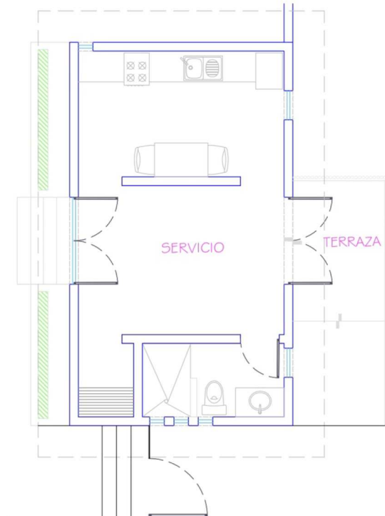
Figura 3. Desplante del área de servicio.
