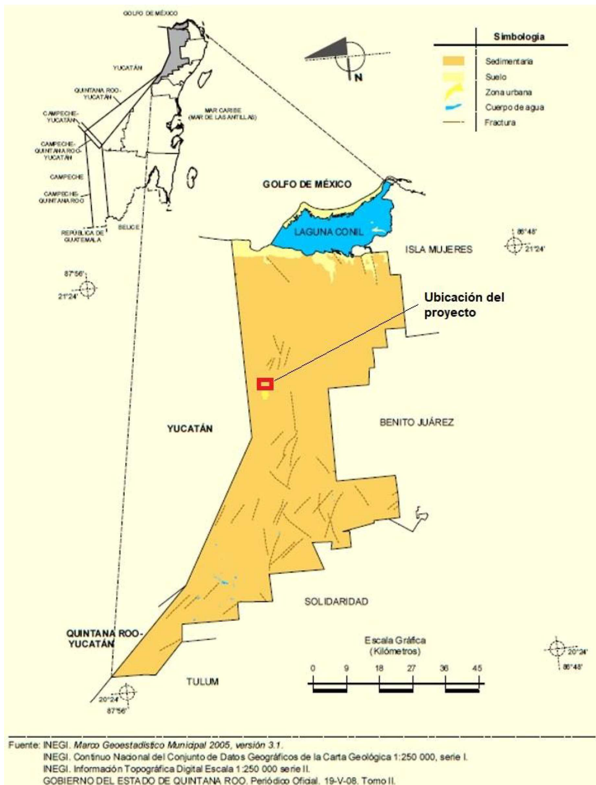
Figura IV.5. Geología establecida en el Prontuario del INEGI (2009) para el municipio de Lázaro Cárdenas, para el sitio del proyecto corresponde a sedimentaria.
