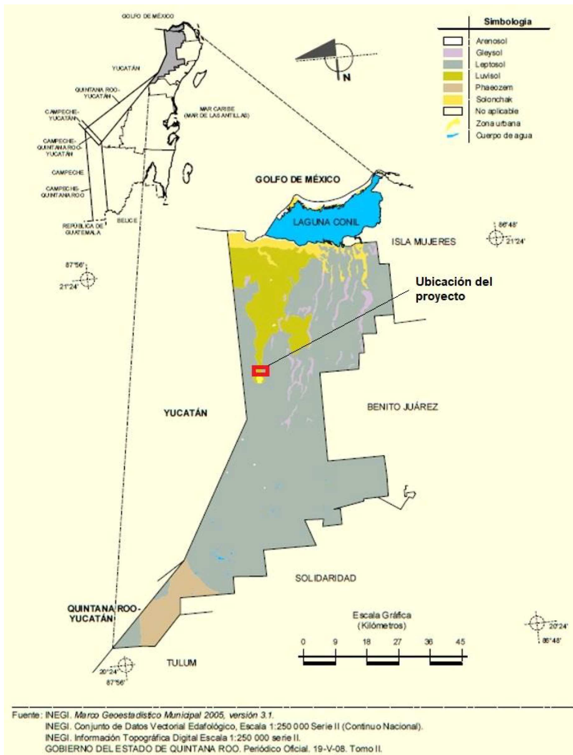
Figura IV.6. Suelos dominantes establecidos en el Prontuario del INEGI (2009) para el municipio de Lázaro Cárdenas.
