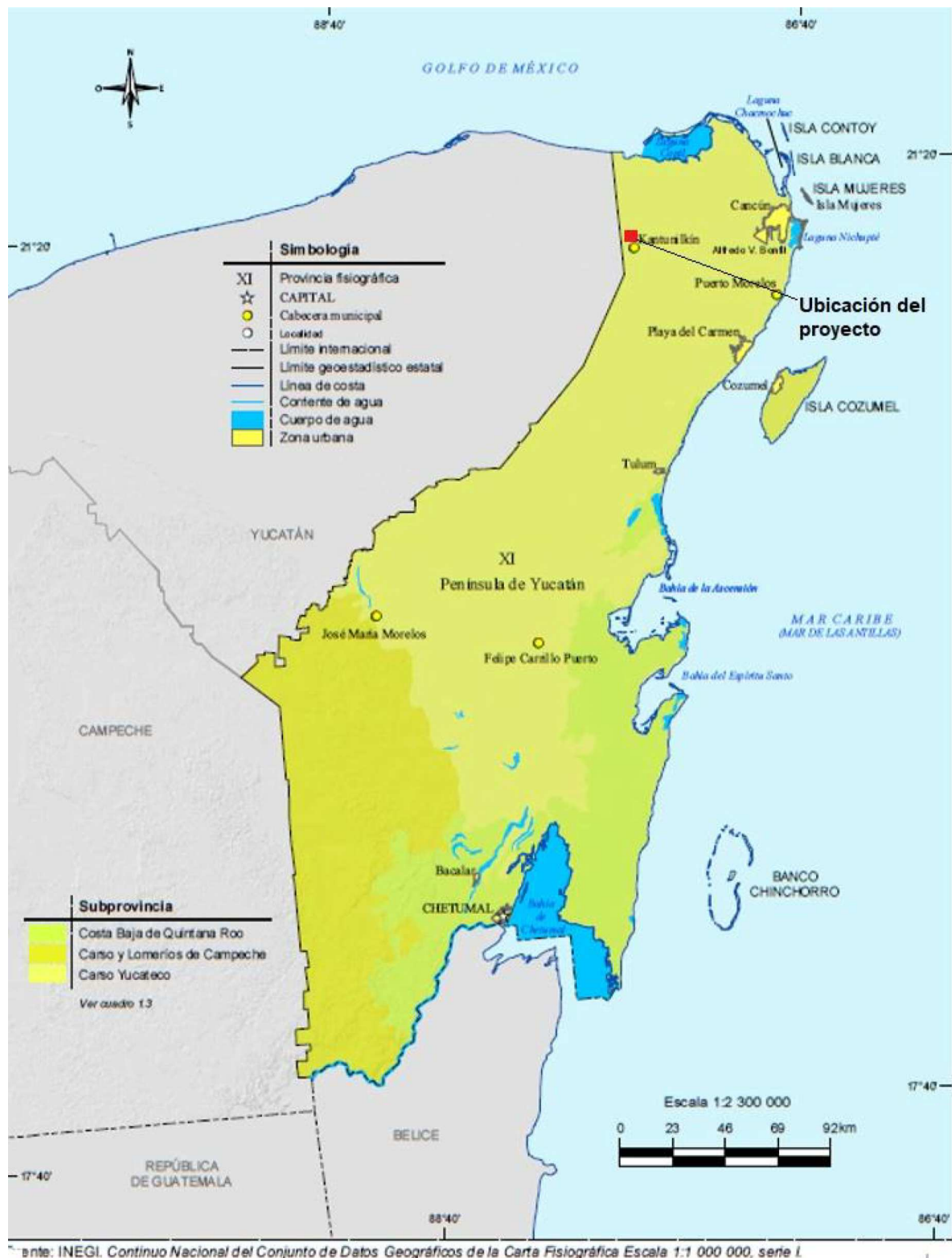
Figura IV.8. Fisiografía establecida en el anuario de Quintana Roo por el INEGI (2017), el sitio del proyecto se encuentra ubicado en el Carso Yucateco.
