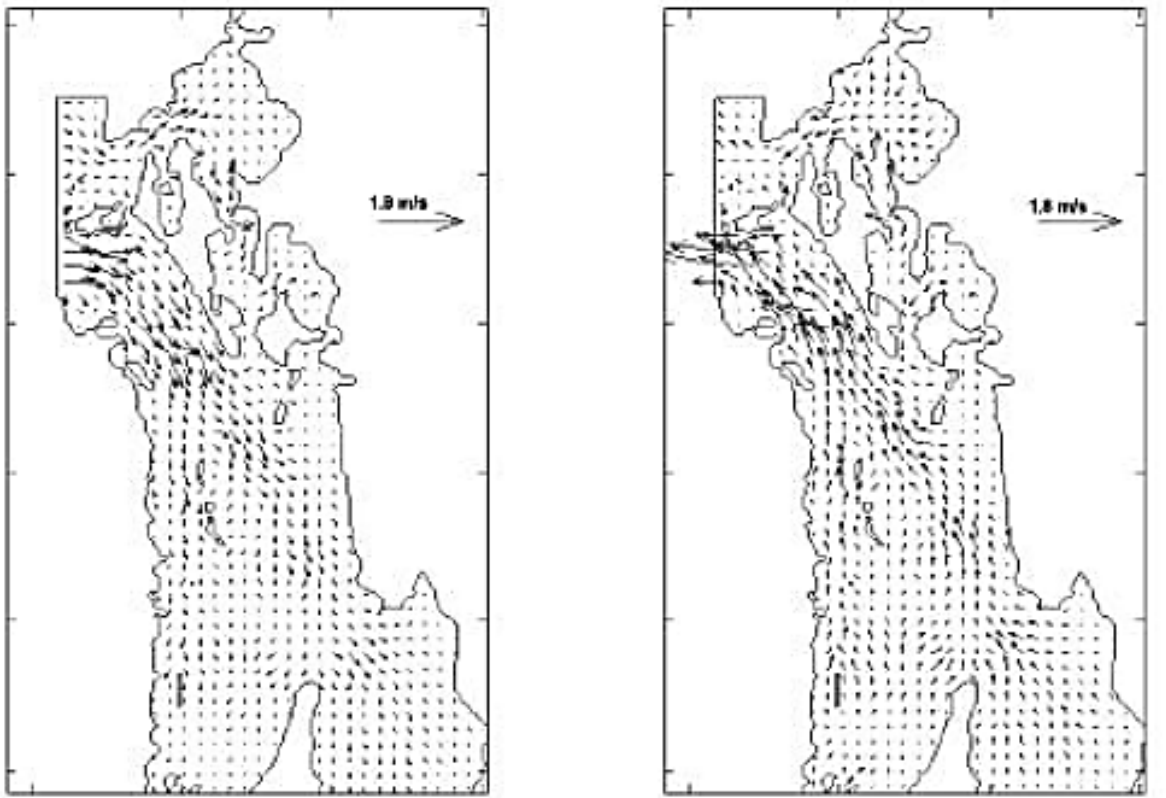
Campo de velocidades del flujo y refluo generado por los 7 armónicos de marea en la boca norte de Santa María La Reforma.
