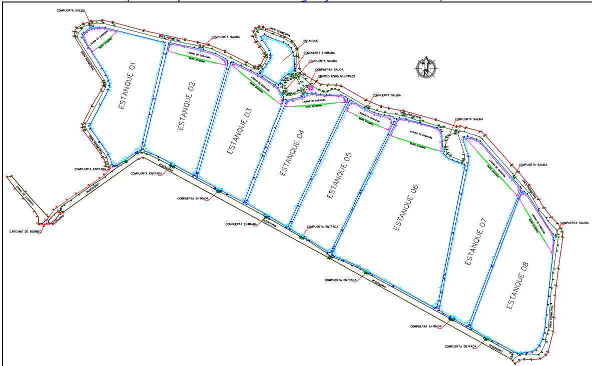
Plano general del proyecto.
