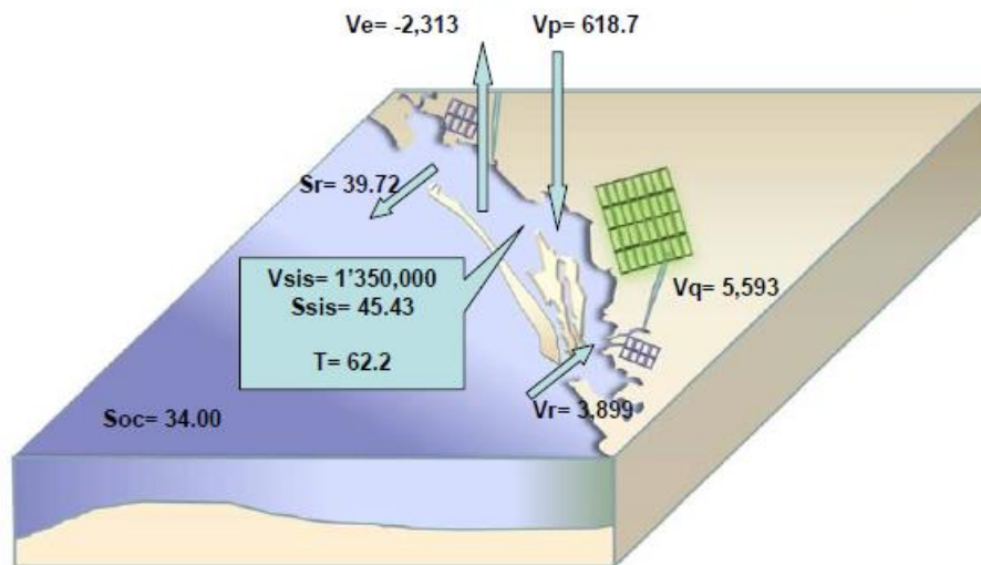
BALANCE DE AGUA Y SAL EN LA LAGUNA SANTA MARÍA-LA REFORMA
