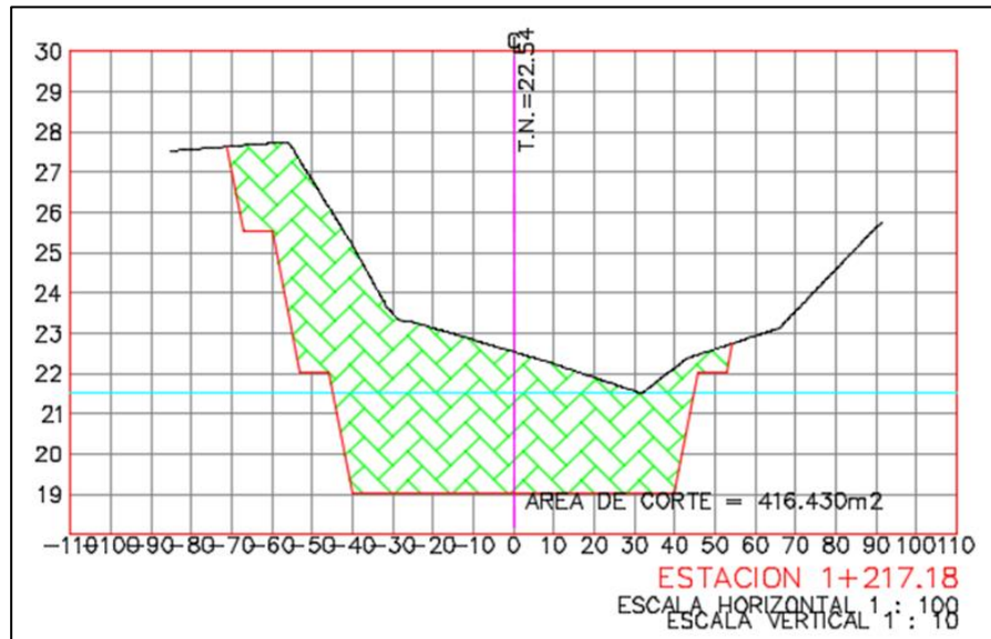
FIGURA 4.- ESTACION 1+217.18 (PARTE FINAL DEL PROYECTO):
