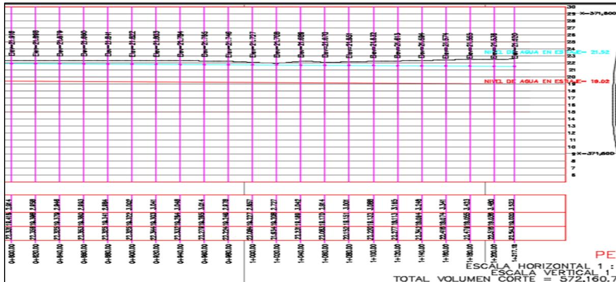
FIGURA 7.- MUESTRA REPRESENTATIVA DE CORTE TRANSVERSAL, DE LA ESTACIÓN 0+800.000 A LA ESTACIÓN 1+217.18
