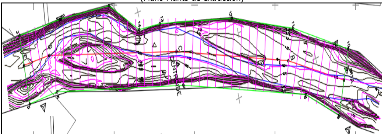
Figura 8.- 5 frentes de extracción divididos en 41 estaciones o secciones. (Plano Planta de extracción)
