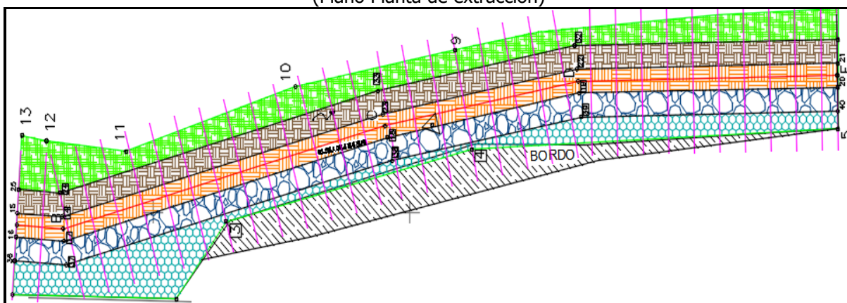
Figura 8.- 5 frentes de extracción divididos en 34 estaciones o secciones. (Plano Planta de extracción)
