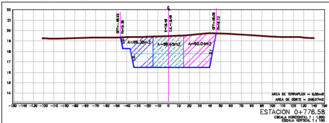
FIGURA 4.- ESTACION 0+776.58 (PARTE FINAL DEL PROYECTO):
