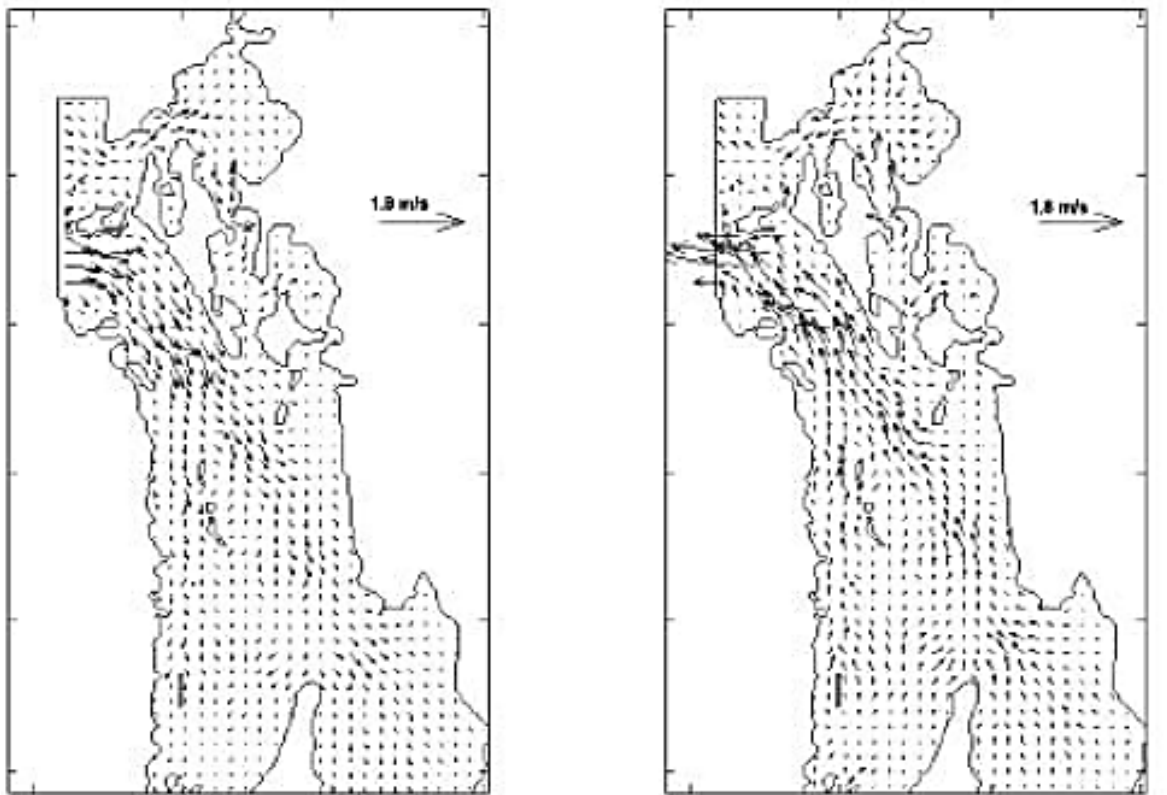
Campo de velocidades del flujo y reflujos generado por los 7 armónicos de marea en la boca norte de Santa María La Reforma.
