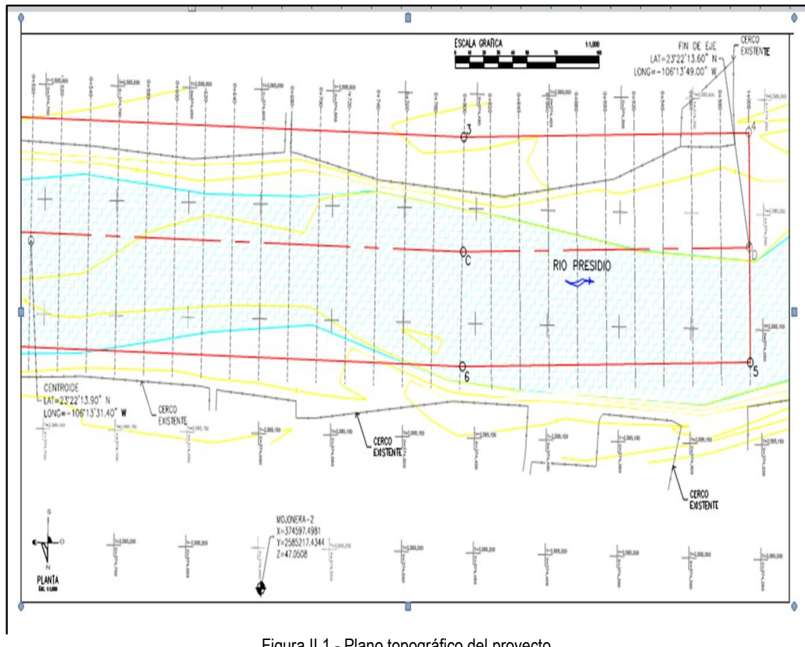
Figura II.1.- Plano topográfico del proyecto
