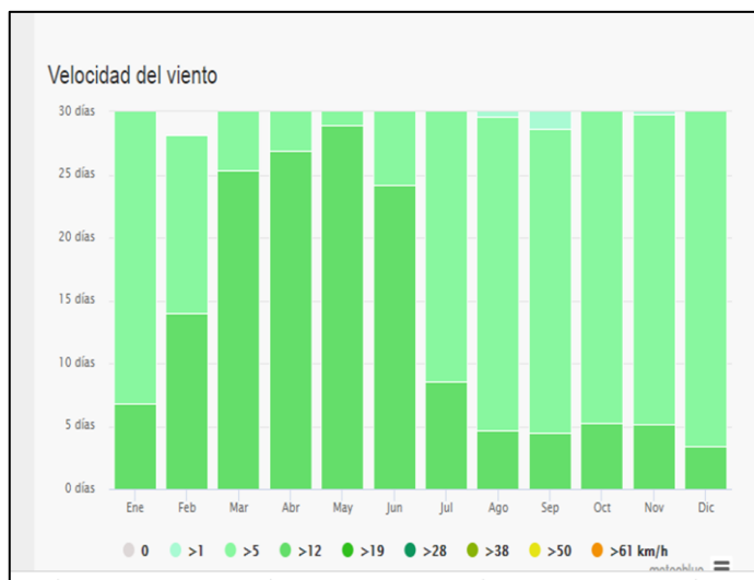
Figura IV.5.- Velocidad del viento.
