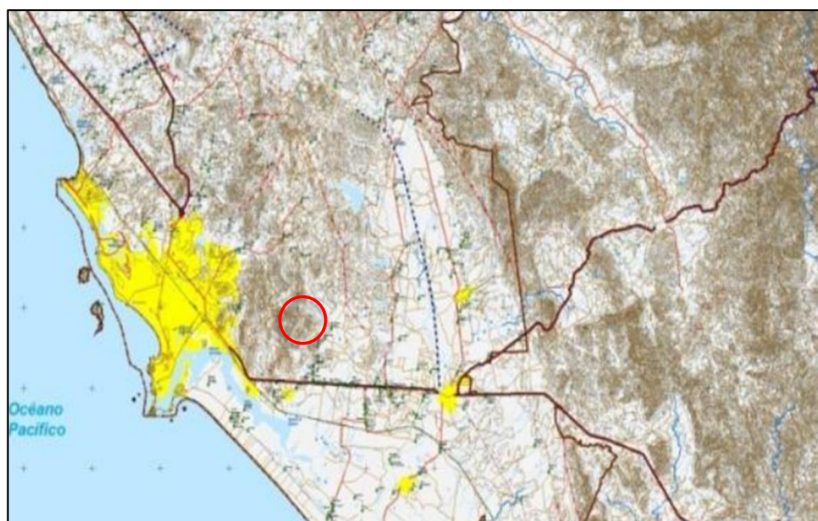
Figura IV.8.- Geomorfología de Sinaloa
