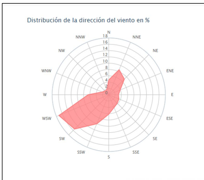
Figura IV.6.- Rosa de los vientos
