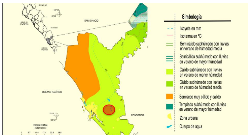
Figura IV.4.- Tipo de clima.
