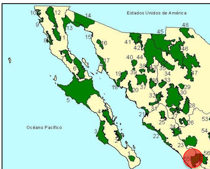
Figura III.5.- Regiones Terrestres.
