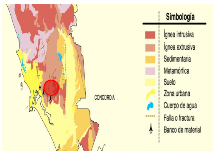
Figura IV.7.- Geología de proyecto.
