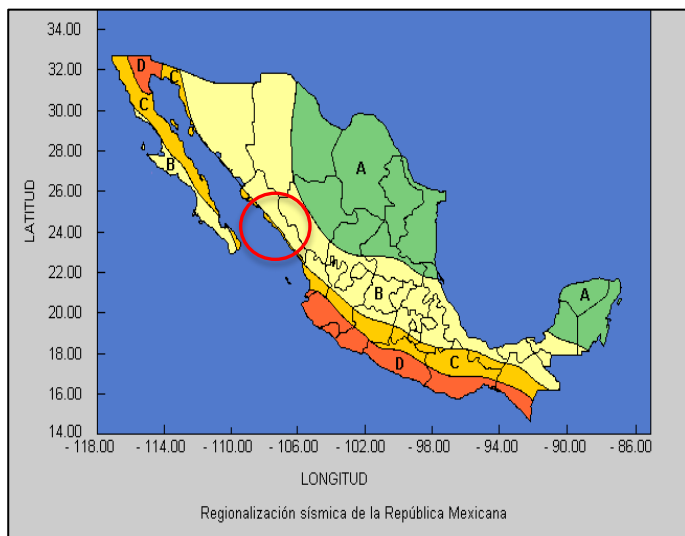
Figura.IV.11.- Zona sísmica.
