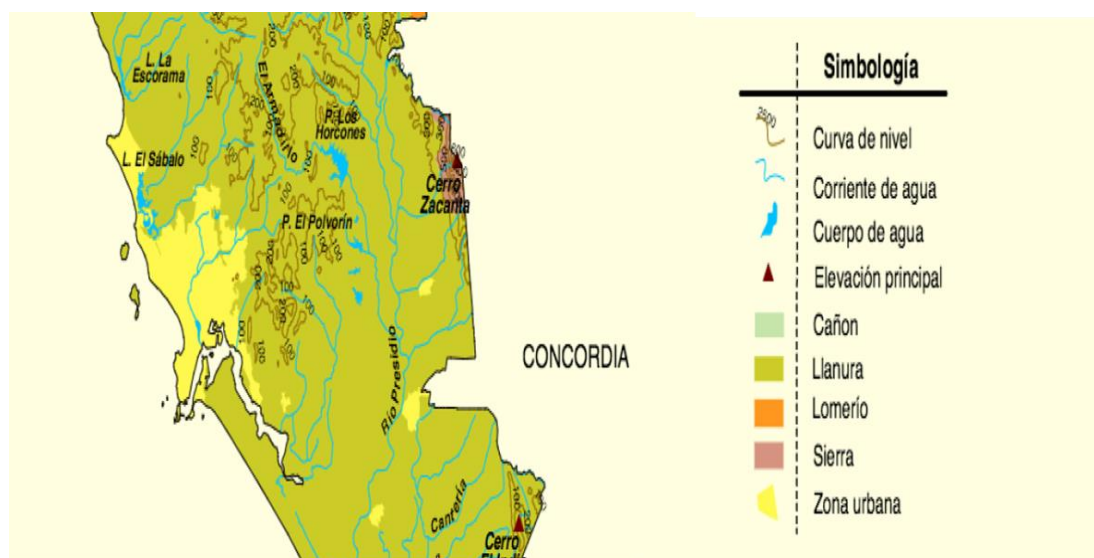
Figura IV.9.- Relieve.
