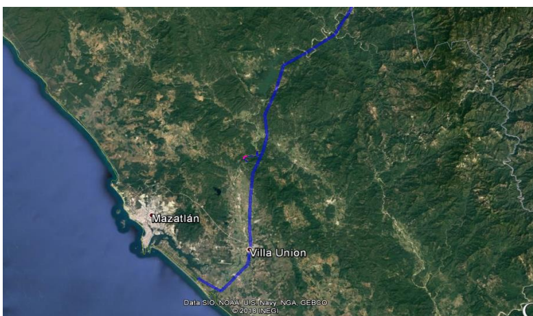
Figura IV.1.- Río Presidio
