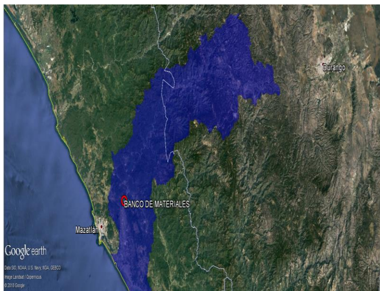
Figura IV.2.- Cuenca hidrológica.
