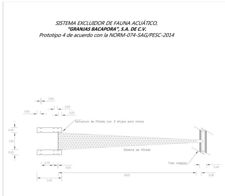
Figura. Sistema excluidor de fauna acuática de prototipo Bolso conectado a registro con tubo excluidor (SEFA-2): a) vista general, b) dispositivo de filtrado y c) especificaciones del colector de organismos.
