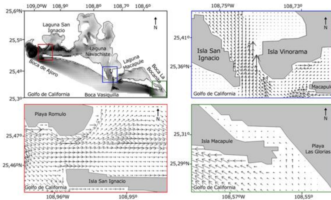
Figura 11. Distribución vectorial de corrientes durante el flujo de la marea, y el forzamiento del viento uniforme de 5 \text{ m s}^{-1} del noroeste
