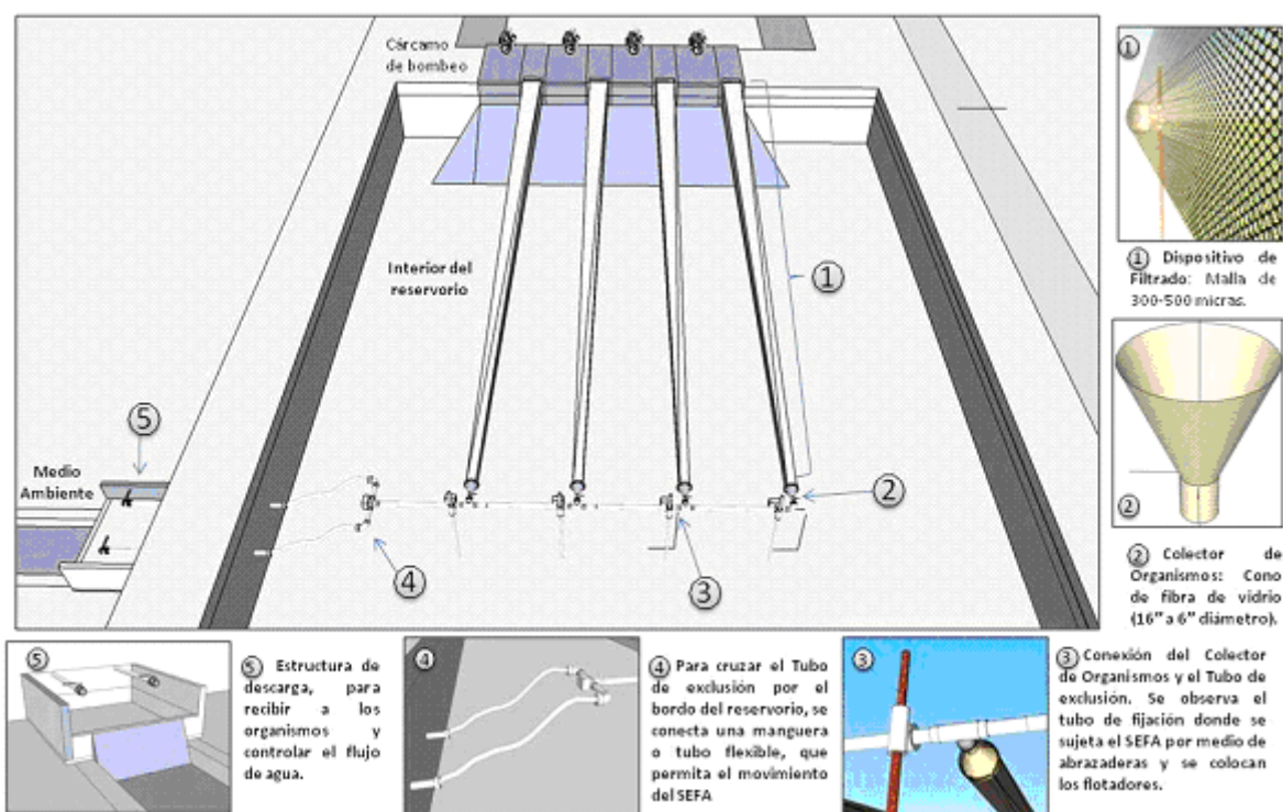
Figura.- Esquema general del SEFA-1 que consiste en unidades de dispositivos excluidores cónicos.
