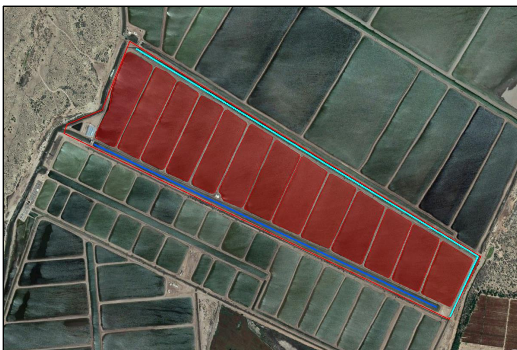
Figura II.1. Distribución de estanques ( ♦ ), reservorio ( — ) y drenes ( — ) en Acuícola Pleamar S.A de C.V.
