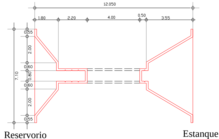
Corte Transversal
