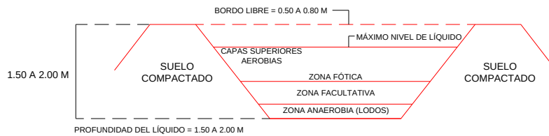
Ilustración 30.- Características de laguna de oxidación.
