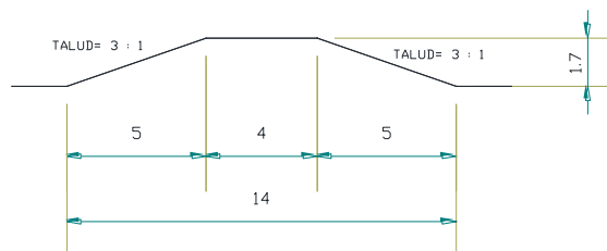
Ilustración 29.- Construcción de estanquería
