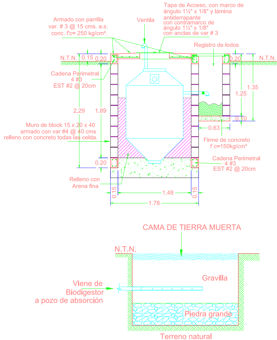
Ilustración 33.- Mecanismo Biodigester
