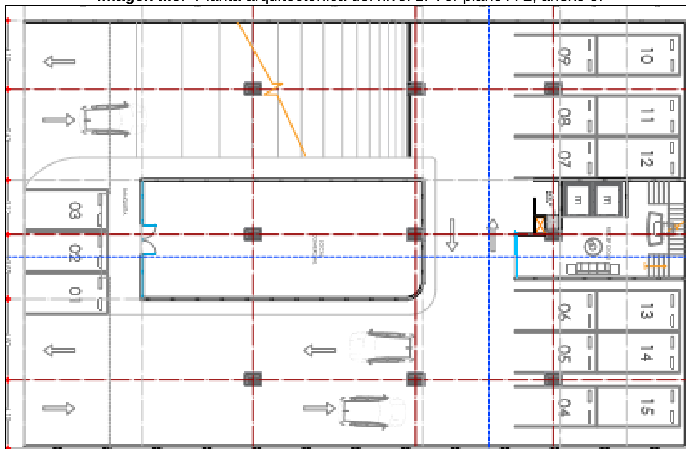
Imagen II.5.- Planta arquitectónica del nivel 1. Ver plano A-2, anexo 5.
