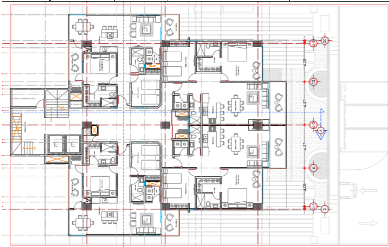
Imagen II.7.- Planta tipo A de los departamentos del nivel 3 al 5. Ver plano A-3, anexo 5.
