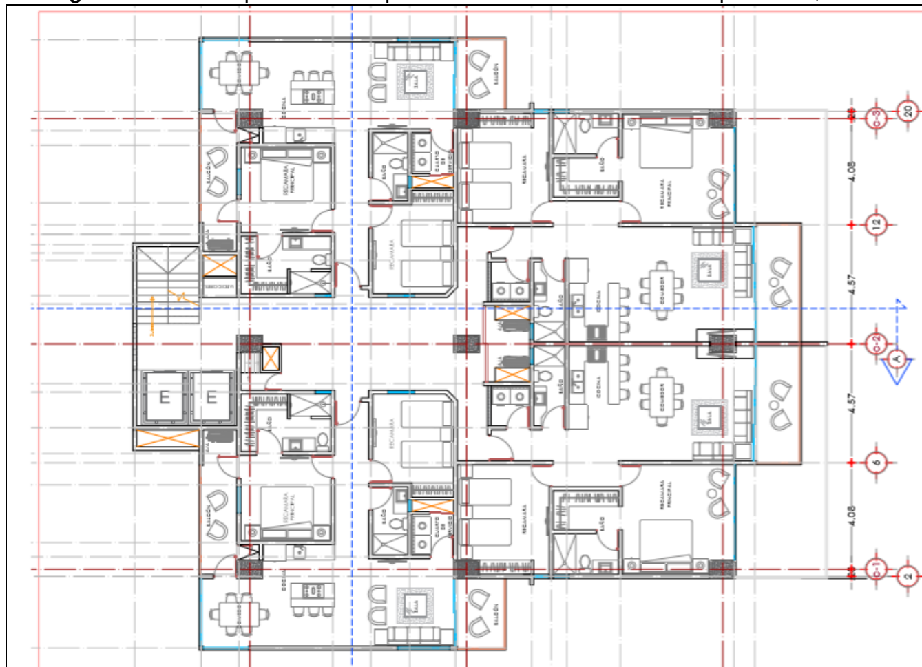
Imagen II.8.- Planta tipo A de los departamentos del nivel 6 al 19. Ver plano A-4, anexo 5.
