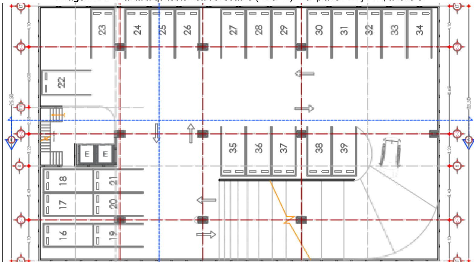
Imagen II.4.- Planta arquitectónica del sótano (nivel -1). Ver plano A-1 y A-2, anexo 5.
