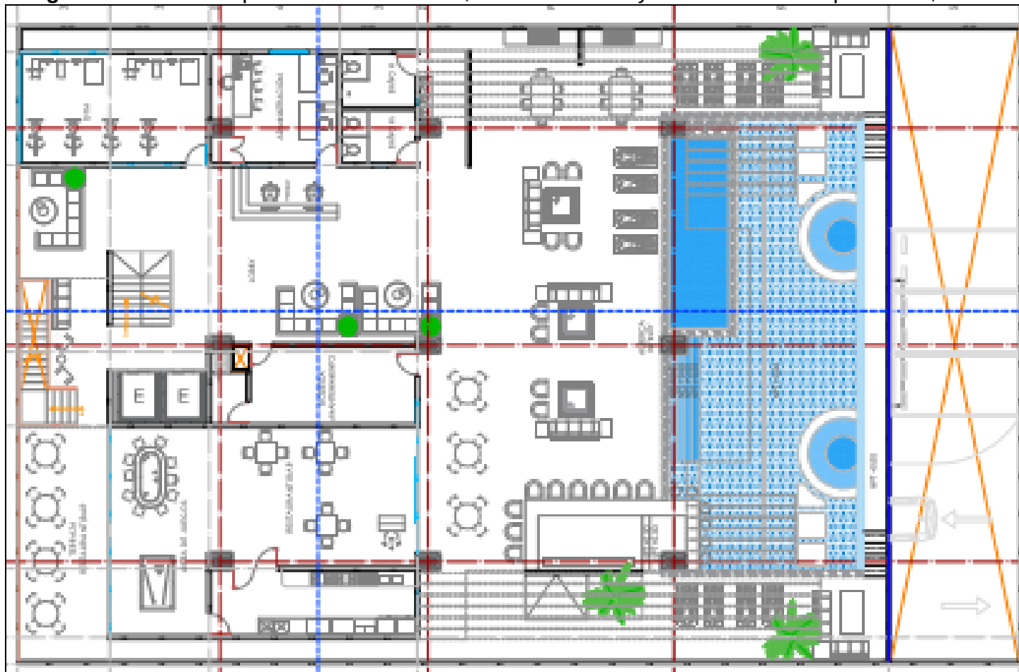
Imagen II.6.- Planta arquitectónica del nivel 2, áreas comunes y amenidades. Ver plano A-3, anexo 5.
