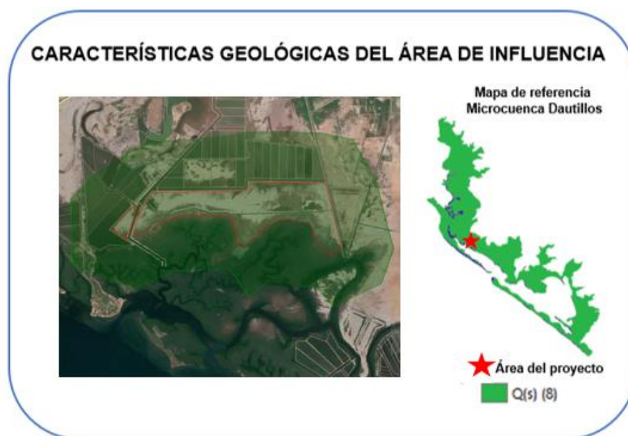
Figura IV.17. Características Geológicas del Área de Influencia
