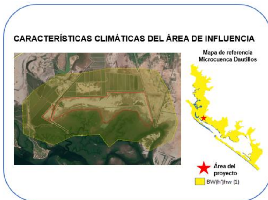
Figura IV.16 Características Climáticas del Área de Influencia
