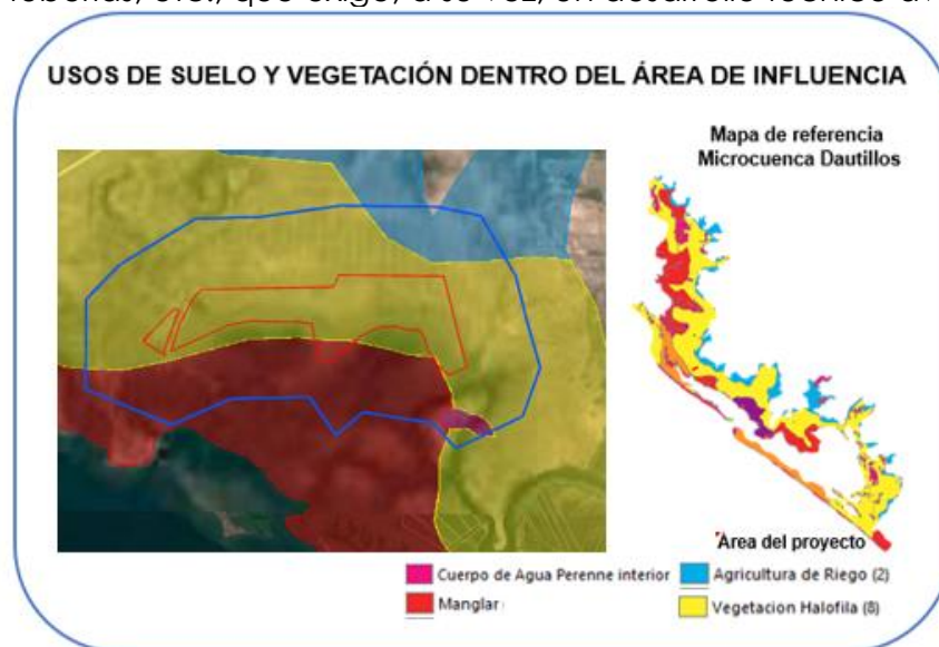
FiguraIV.20.- Uso de suelo y vegetación en el área de Influencia
