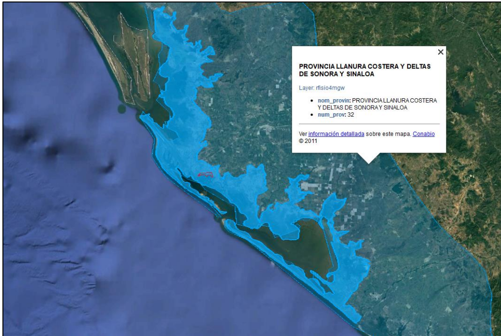
Figura IV.4.- Ubicación del Sistema Ambiental con respecto a la región fisiográfica.
