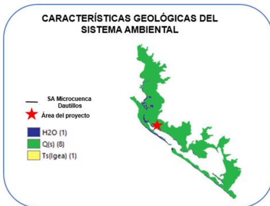
FiguraIV.7.-Características Geológicas del SA
