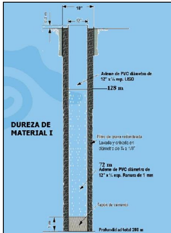
Figura II-8. Diseño del pozo de agua salada.
