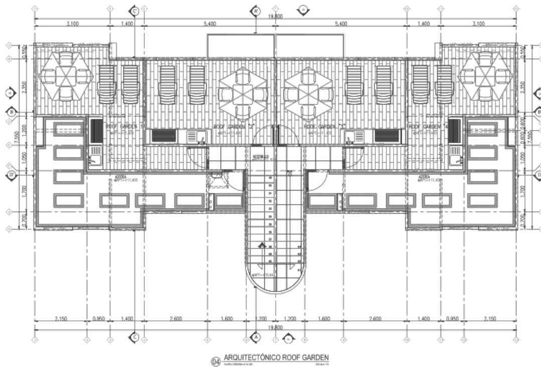
Figura 7.- Planta arquitectónica del roof garden.
