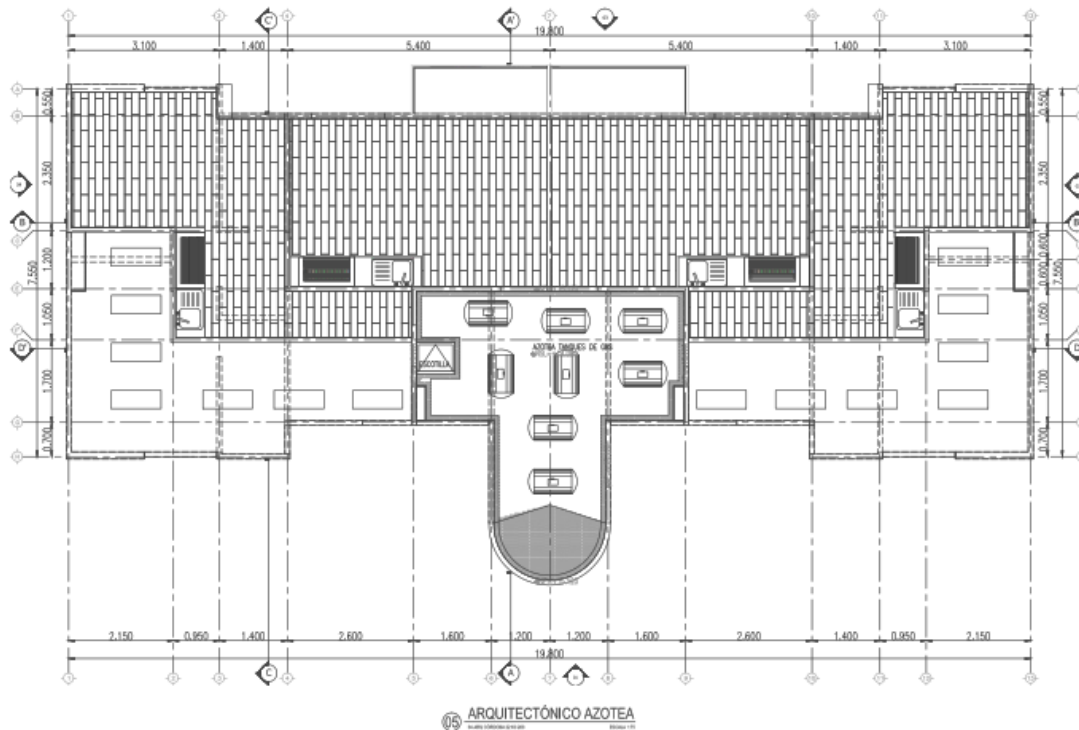
Figura 8.- Planta arquitectónica del nivel de azoteas.
