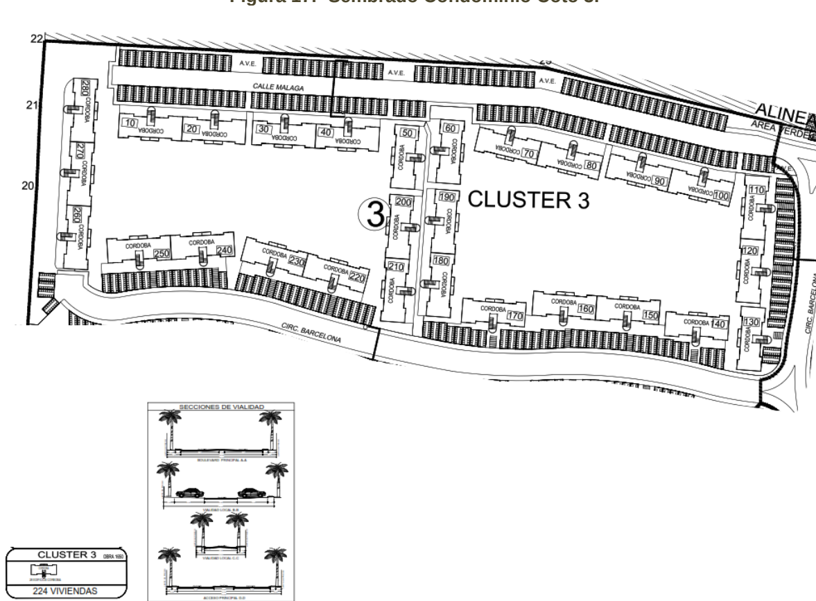
Figura 17.- Sembrado Condominio Coto 3.
