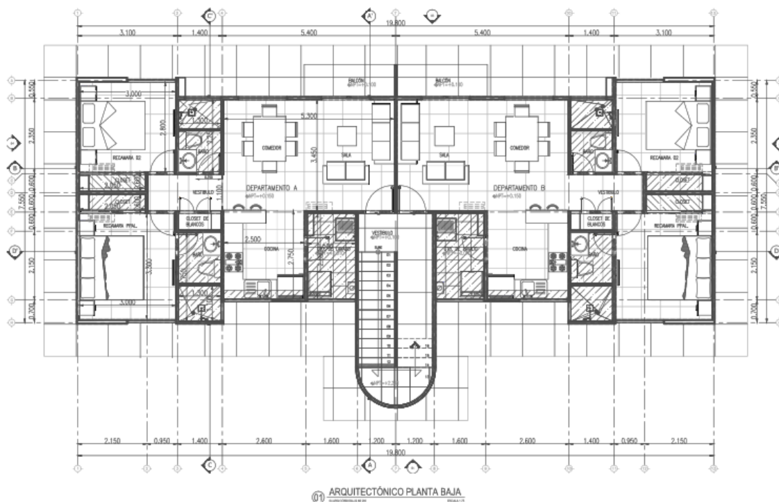
Figura 6.- Arquitectónico de las áreas del nivel tipo donde se observa los dos departamentos y escalera.
