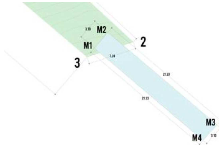
Figura 2.13. diseño del muelle pilotado de maderal del proyecto.
