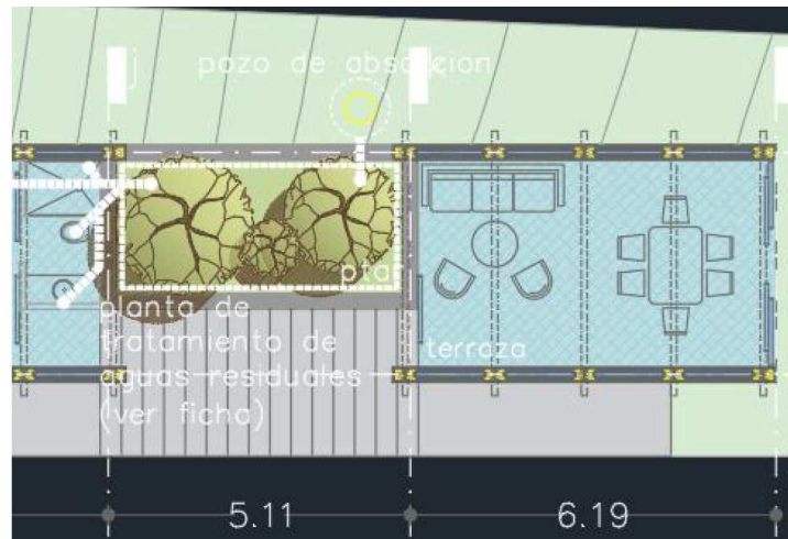
Figura 2.12. PTAR.
