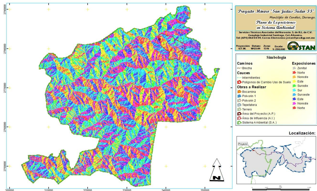
Figura IV-8. Exposición de la pendiente a nivel SA, AI y proyecto
