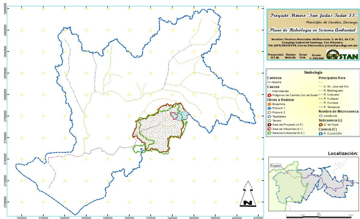
Figura IV-9. Ubicación dentro del marco hidrológico
