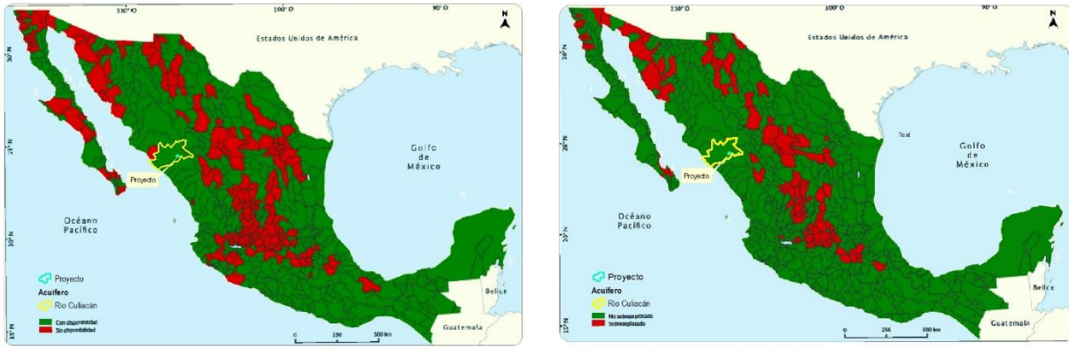
Figura IV-10. Disponibilidad de agua y sobreexplotación de acuíferos (AAM 2018)
