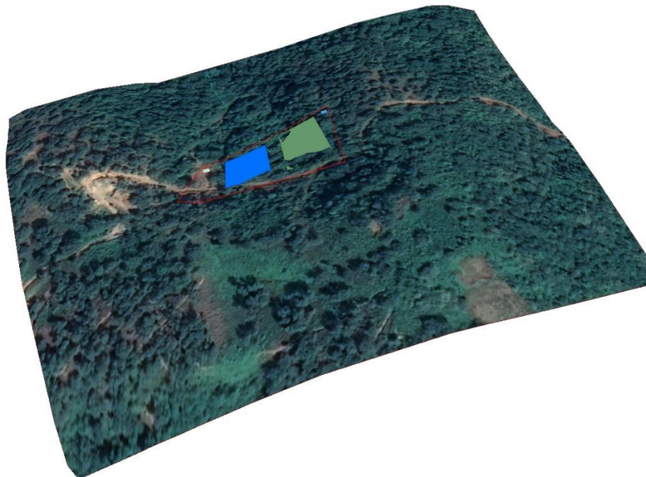
Figura IV-6. Determinación del relieve dentro del área del proyecto
