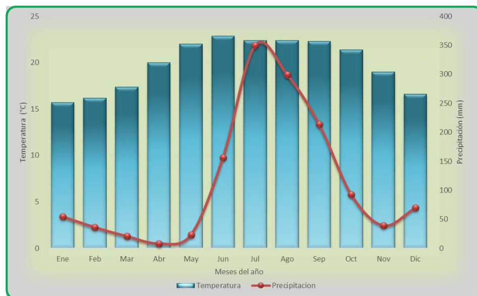
Figura IV-2. Isoterma de la estación climatológica de Canelas, municipio de Canelas, Dgo.
