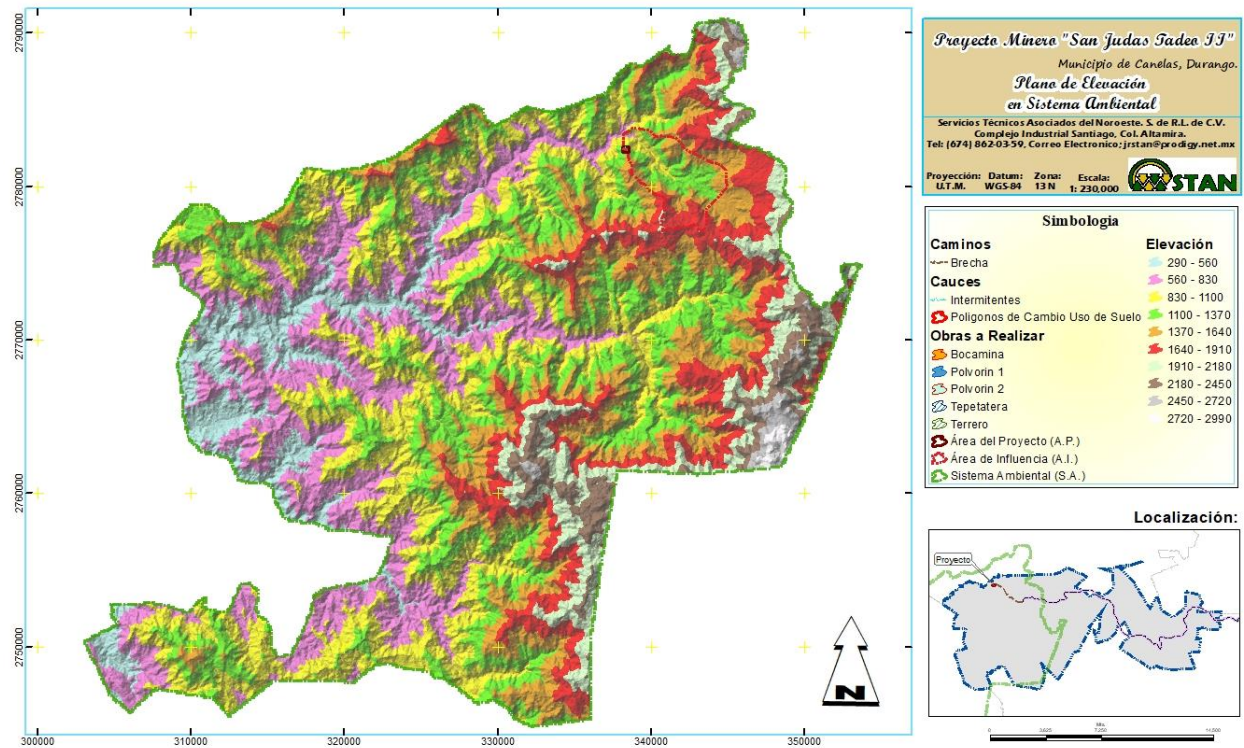
Figura IV-5. Elevación media del SA, AI y sitio y vista general del sitio en 3D, creada a partir del modelo TIN
