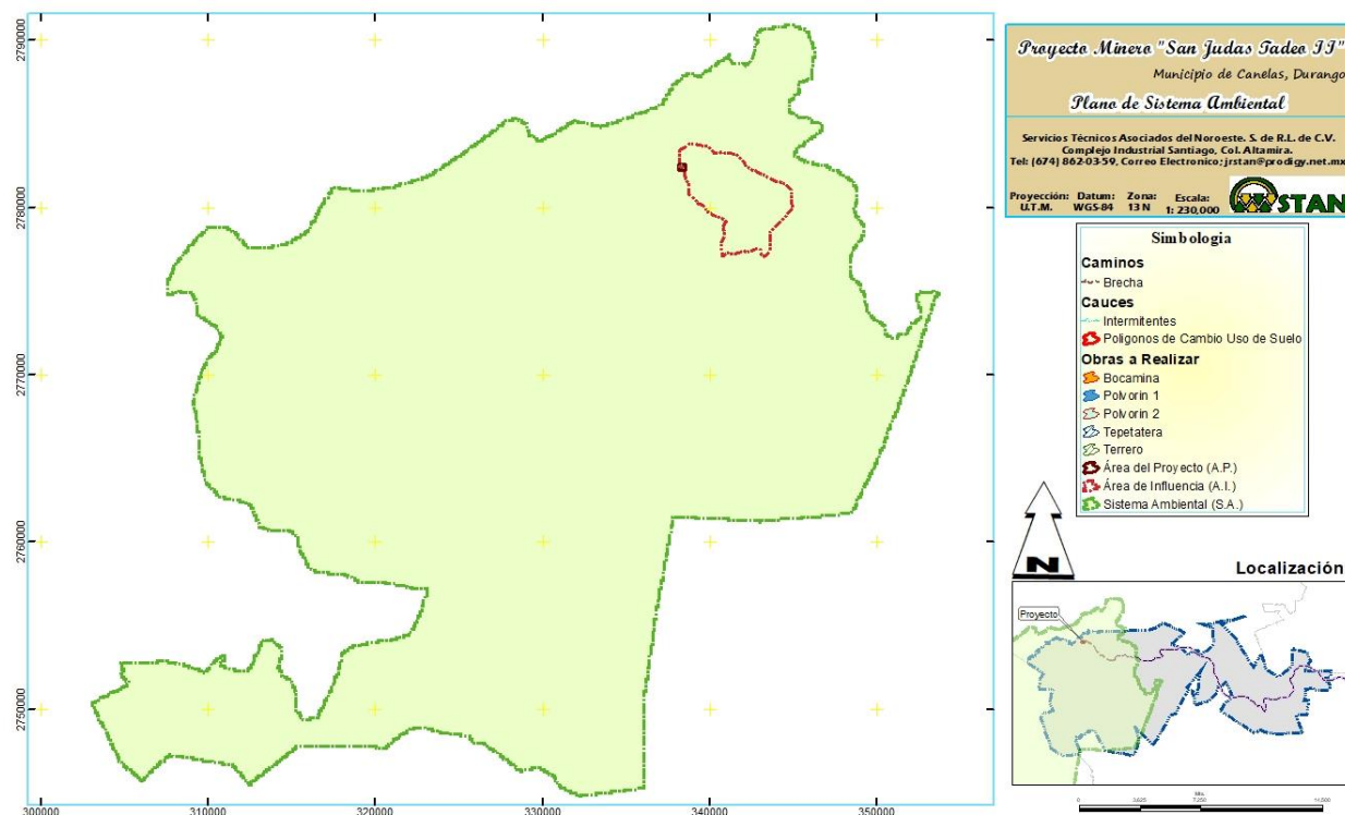
Figura IV-1. Ubicación del proyecto a nivel del sistema ambiental
