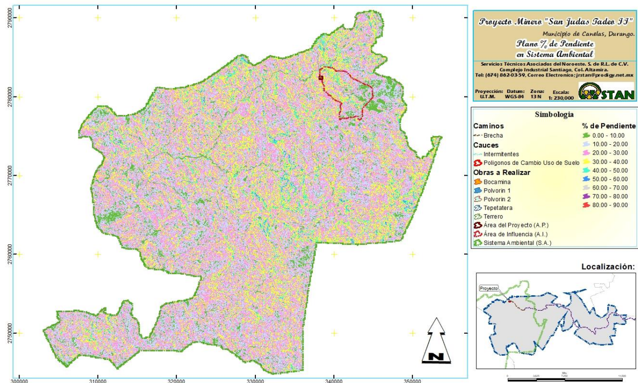
Figura IV-7. Rango de pendiente dentro del SA, AI y proyecto
