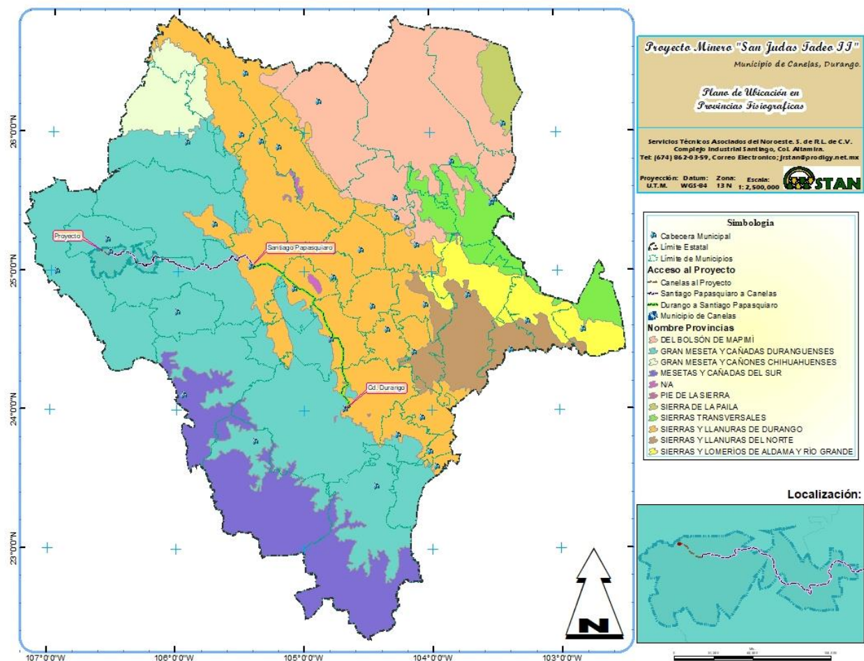
Figura IV-4. Ubicación del proyecto dentro de la fisiografía estatal
