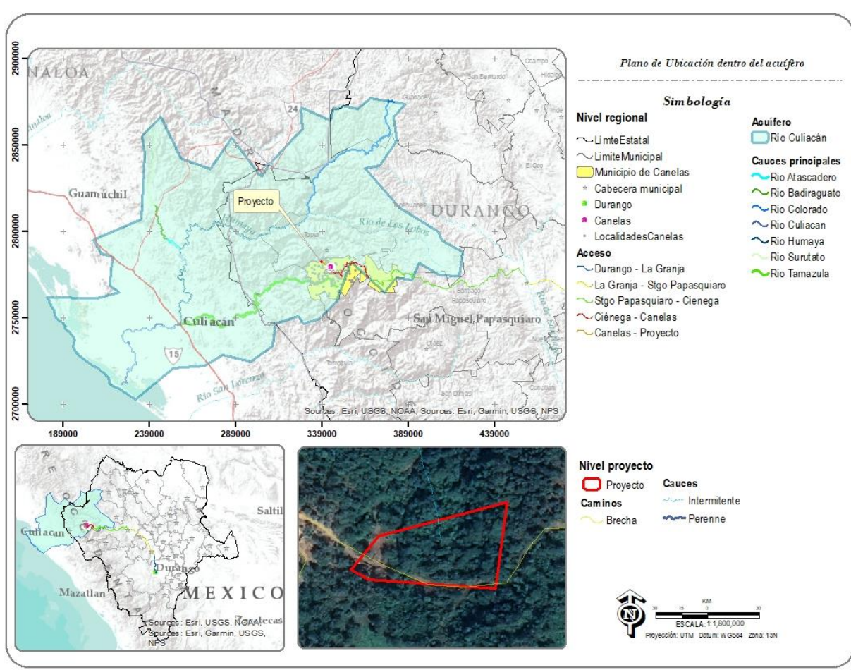
Figura IV-11. Ubicación del proyecto dentro del acuífero
