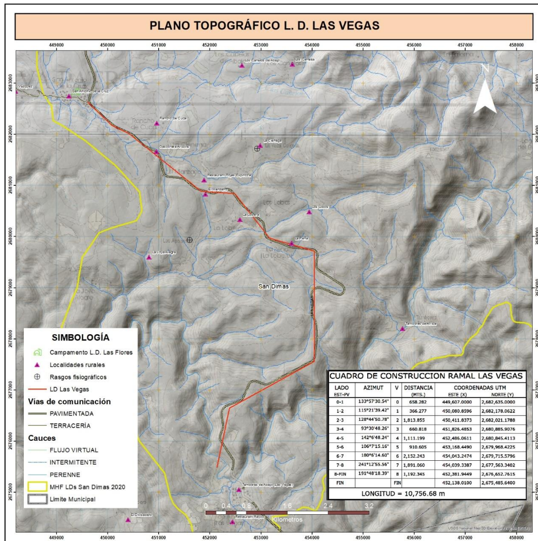
Figura II-5 Plano topográfico L. D. Las Vegas
