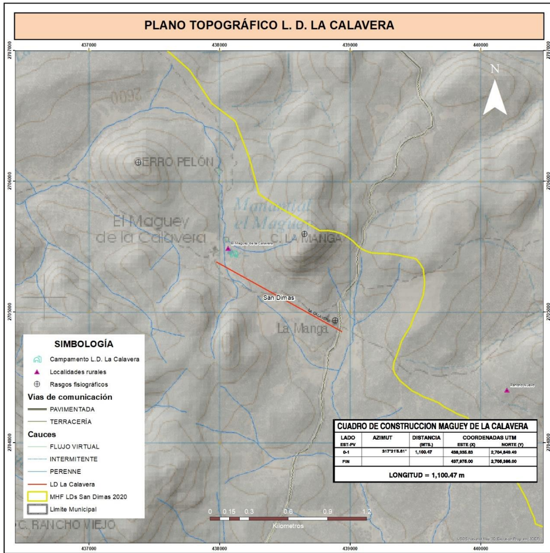
Figura II-3 Plano topográfico L. D. La Calavera
