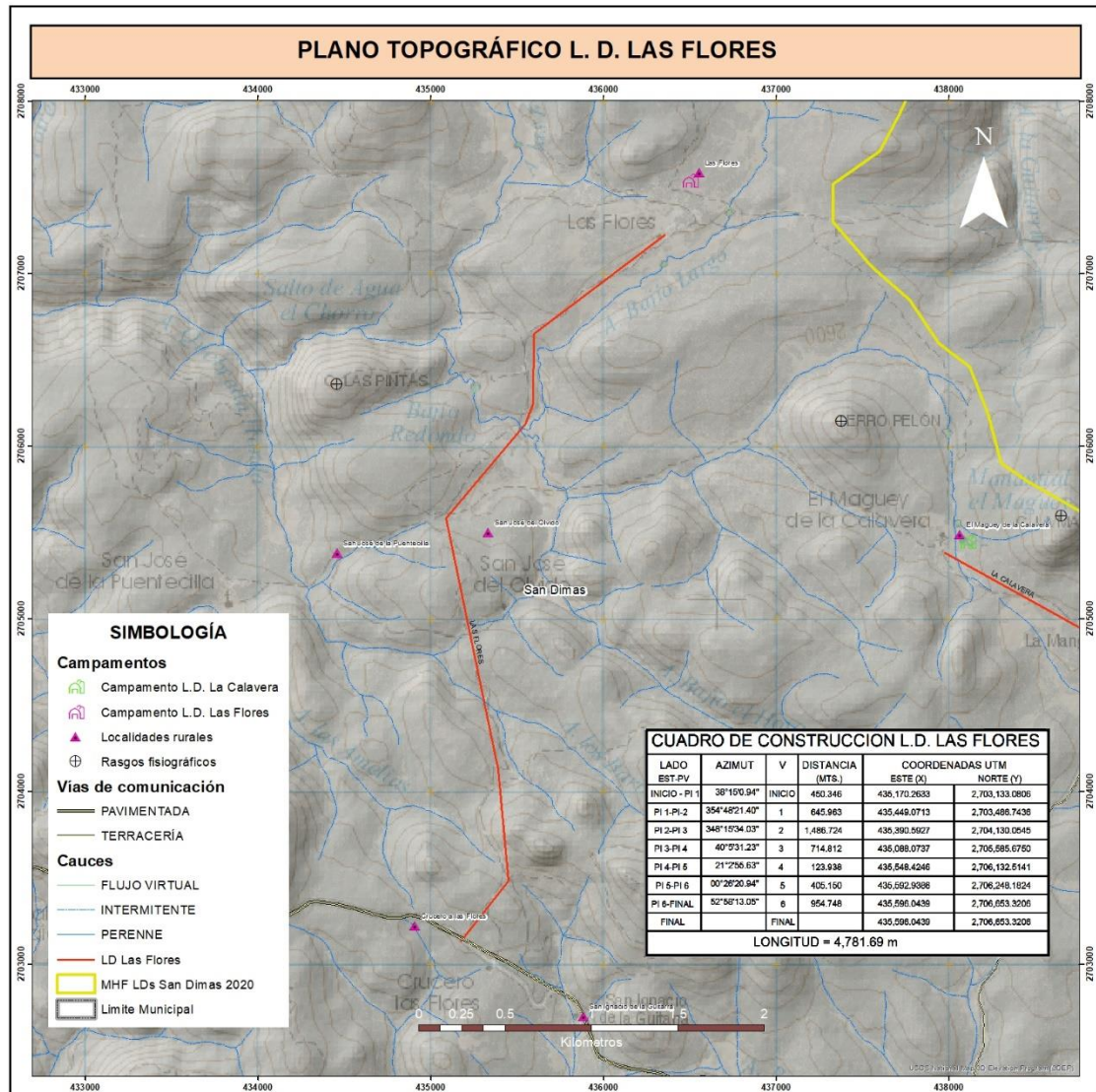
Figura VIII-11 Topografía L. D. Las Flores
