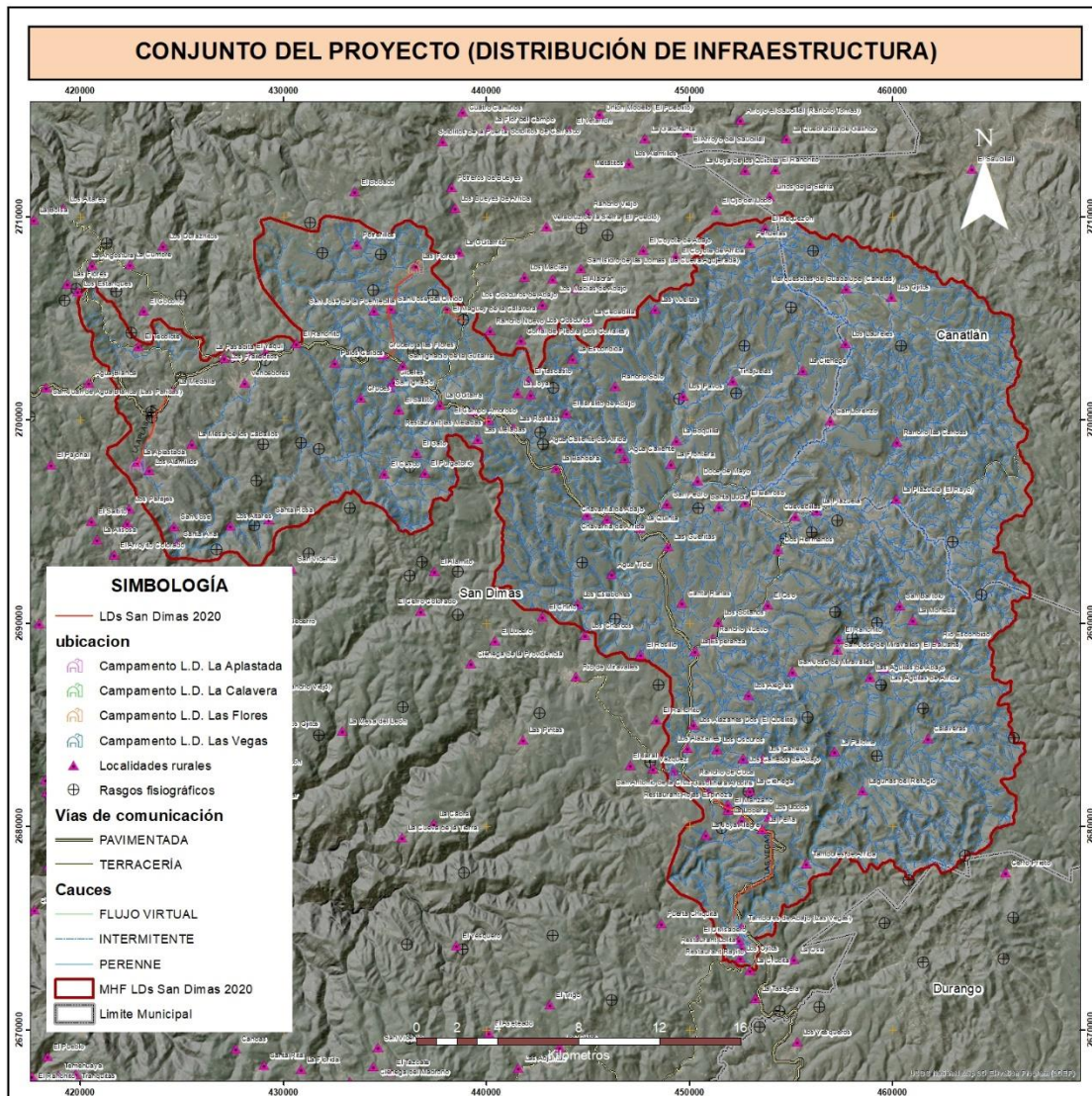
Figura II-6 Conjunto del proyecto
