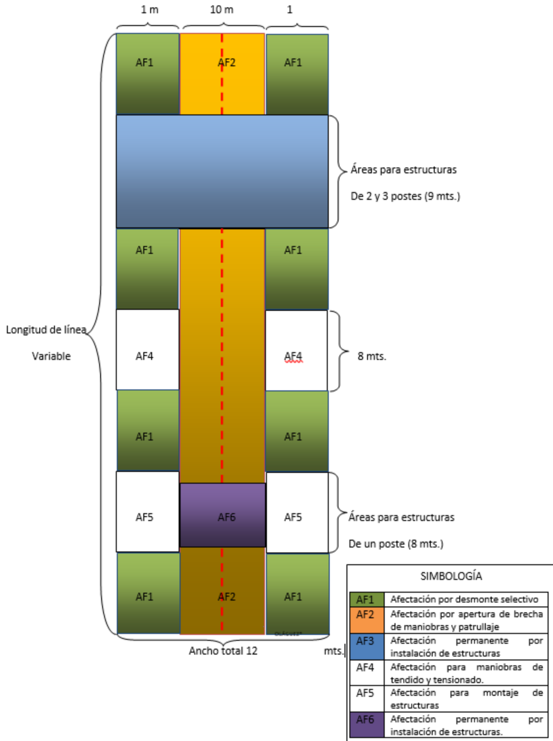
Figura II-1 Descripción del nuevo uso de suelo
