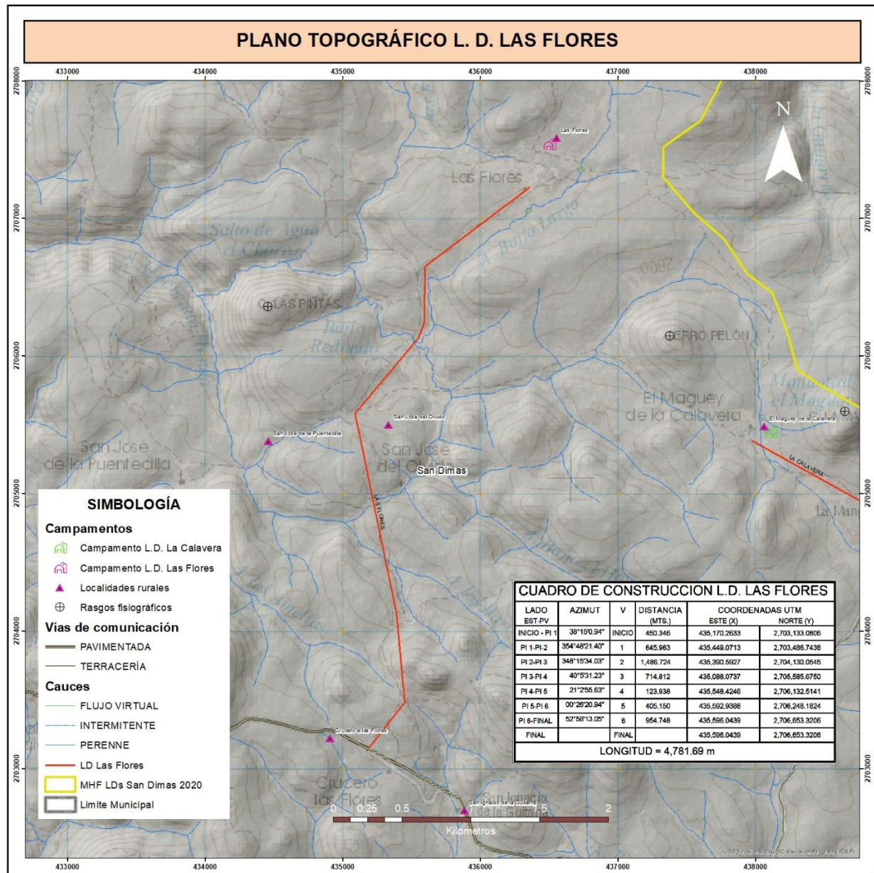
Figura II-4 Plano topográfico L. D. Las Flores
