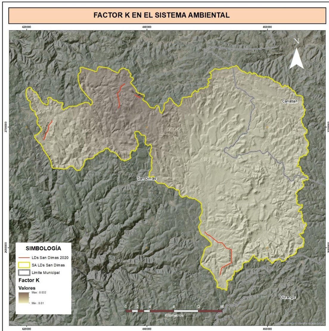
Figura IV-17 Estimación del factor K para el SA
