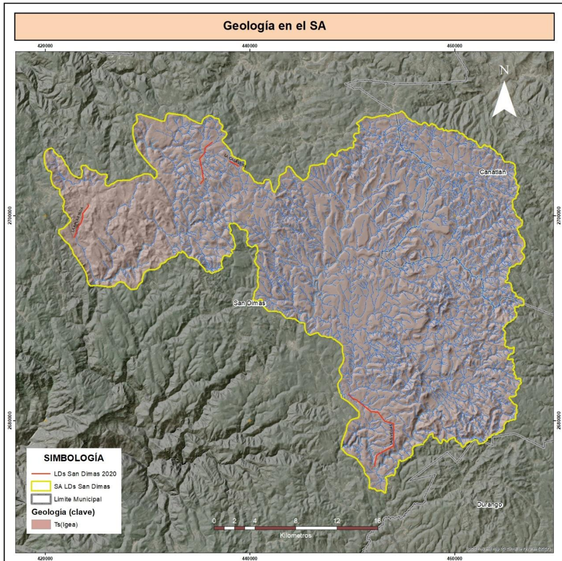
Figura VIII-6 Geología
