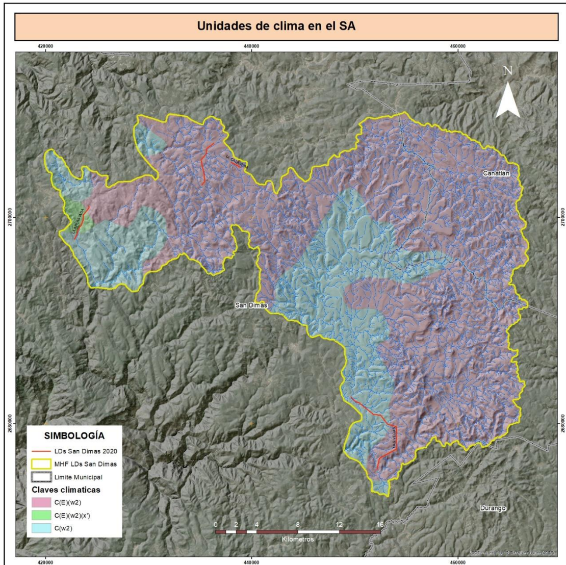
Figura VIII-3 Climas
