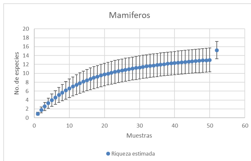
Gráfica IV-6 Curva de acumulación de especies para la mastofauna
