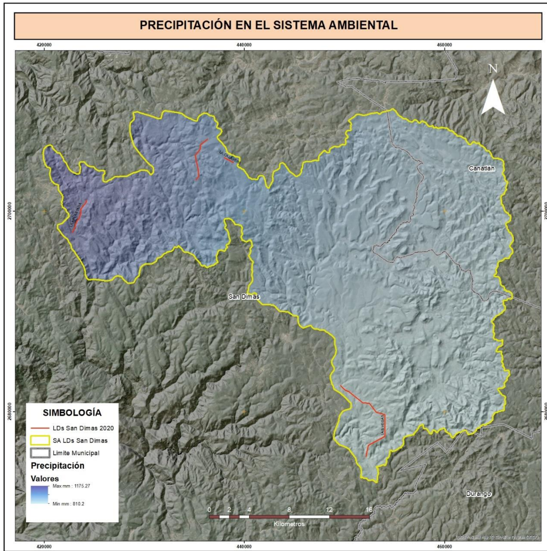
Figura IV-15 Raster de precipitación promedio anual para el SA
