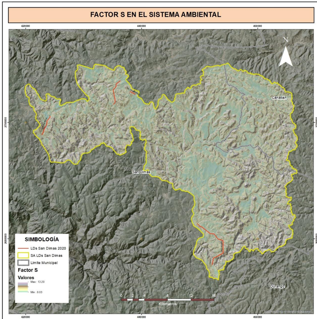
Figura IV-21 Estimación del factor S para el SA
