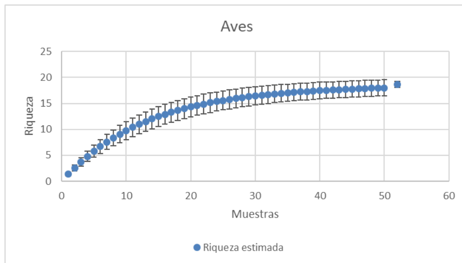
Gráfica IV-5 Curva de acumulación de especies para la avifauna
