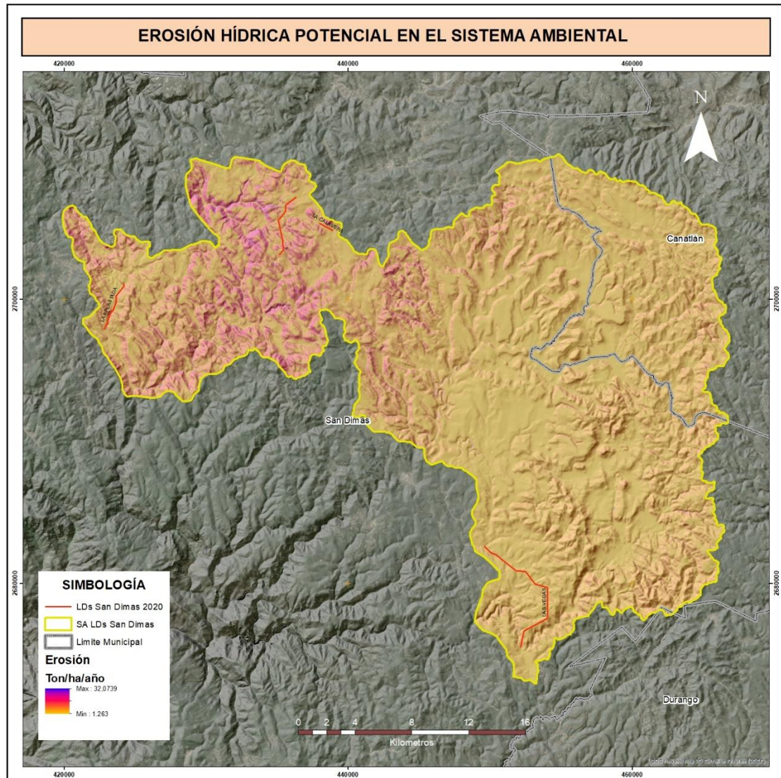
Figura VIII-8 Erosión potencial
