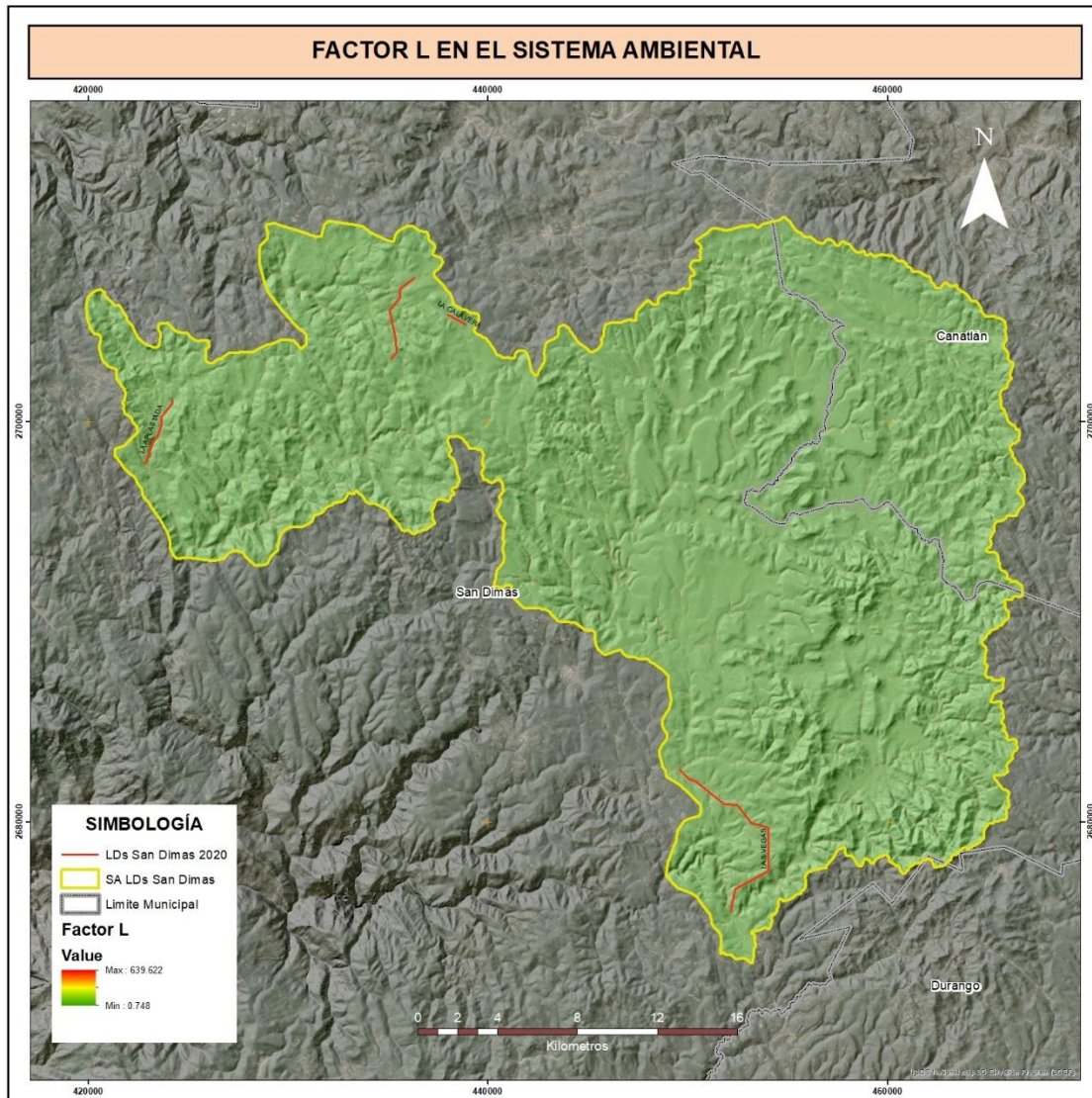
Figura IV-20 Estimación del factor L para el SA
