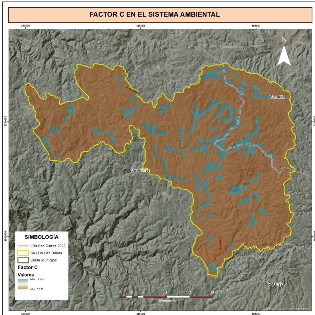
Figura IV-24 Estimación del factor C del SA
