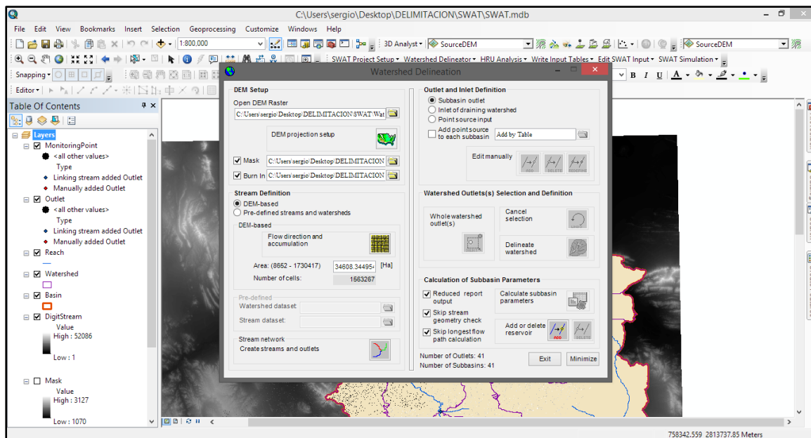
Figura IV-3 Modulo de ArcSwat para generar la delimitación del SA
