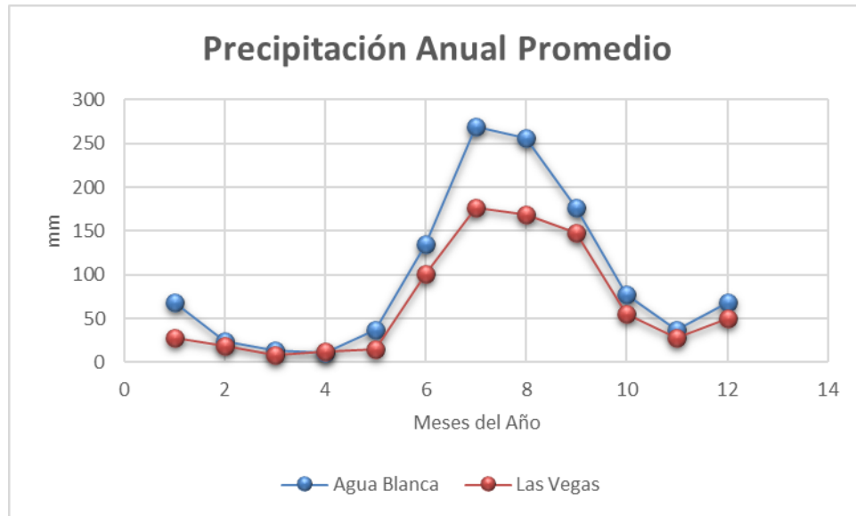
Gráfica IV-2 Precipitaciones anuales
