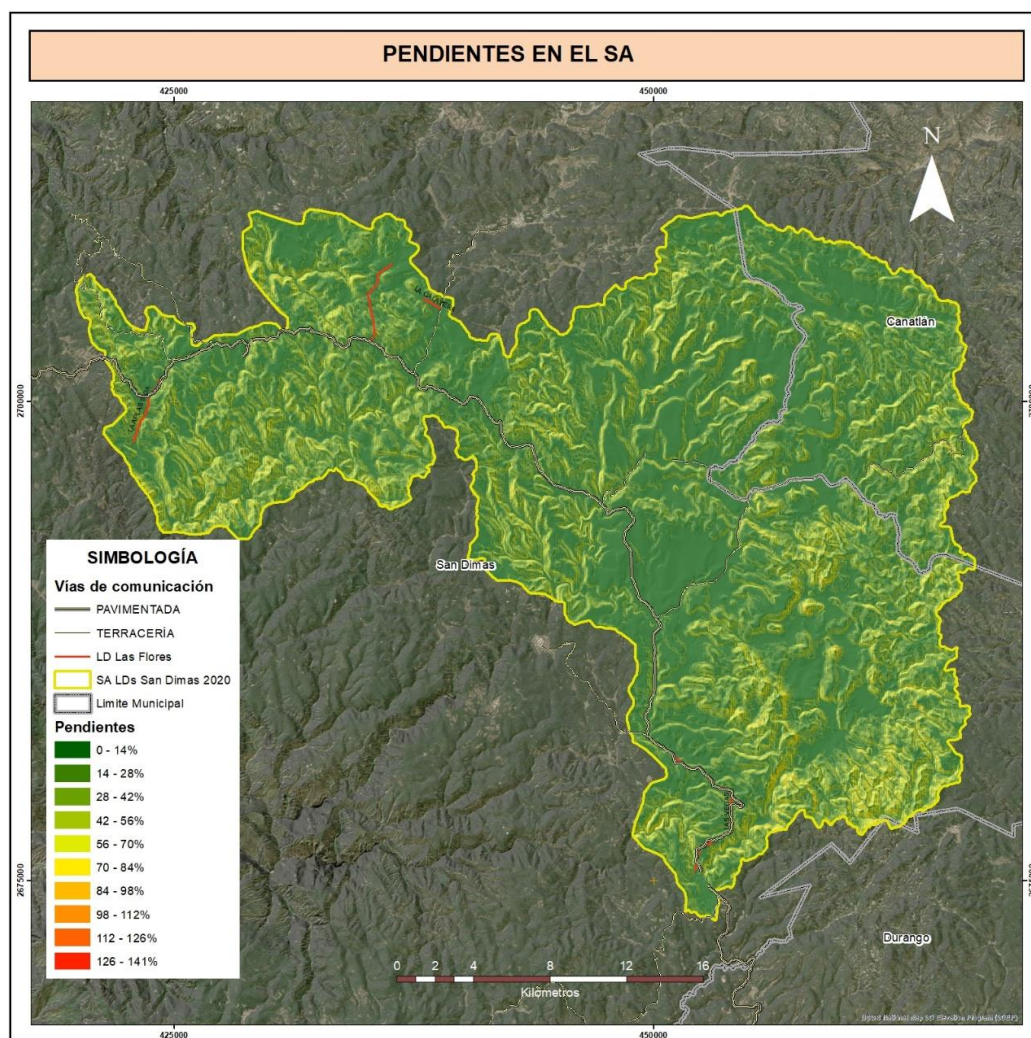
Figura IV-6 Pendientes del sistema ambiental
