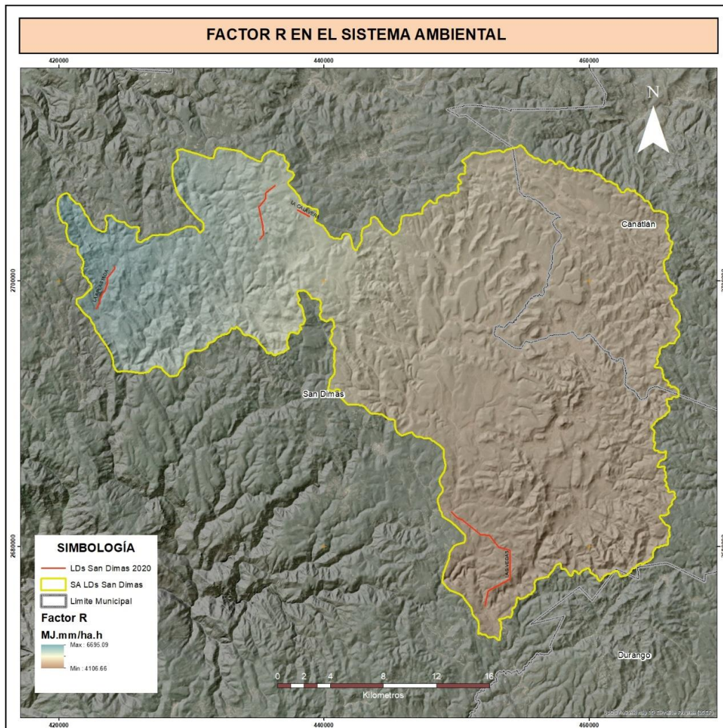
Figura IV-16 Estimación del factor R para el SA
