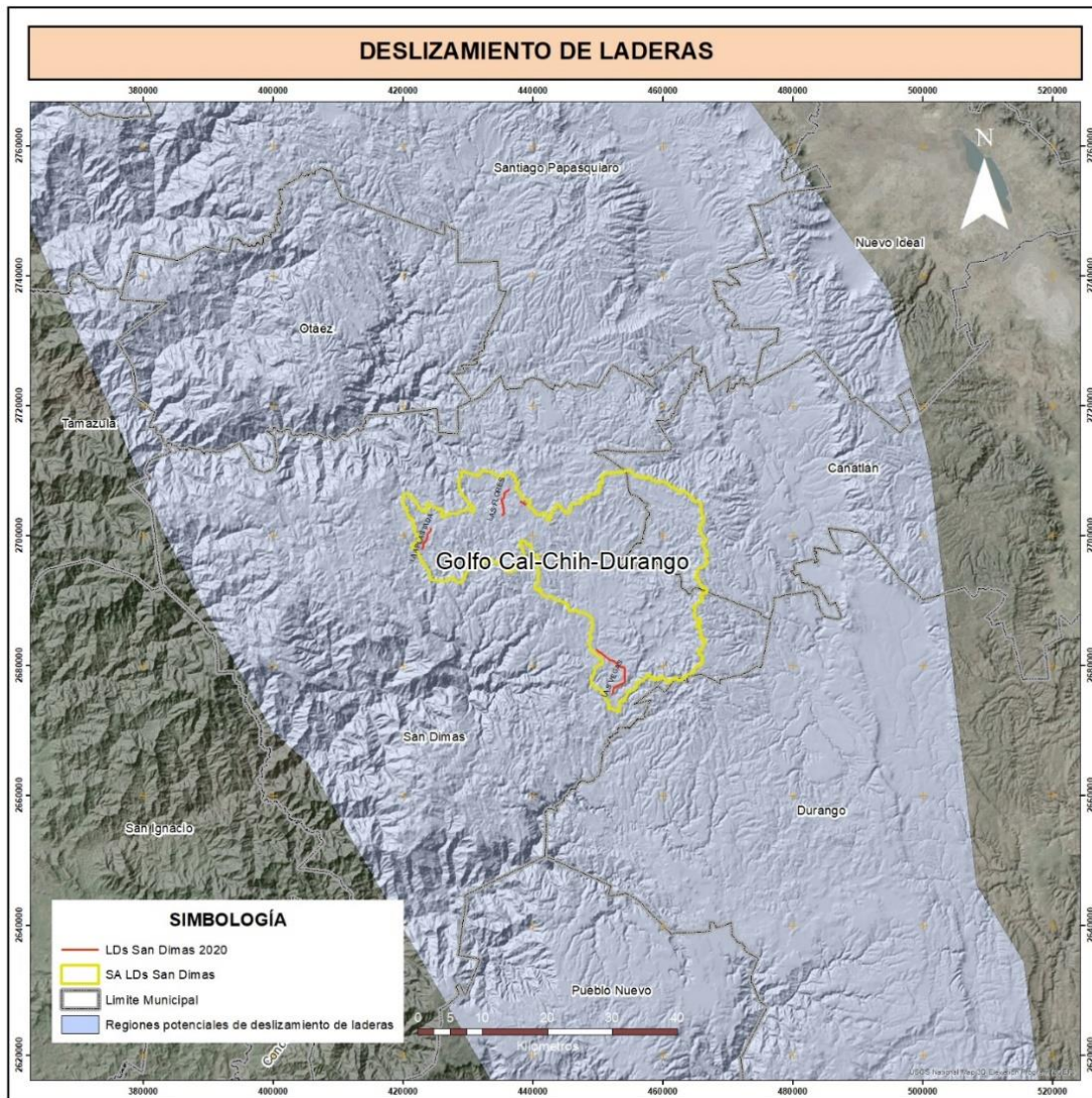
Figura IV-9 Regiones potenciales de deslizamiento de laderas
