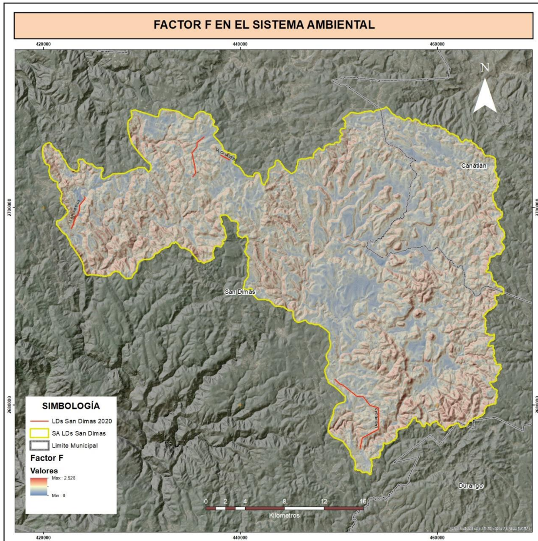
Figura IV-18 Estimación del factor F para el SA
