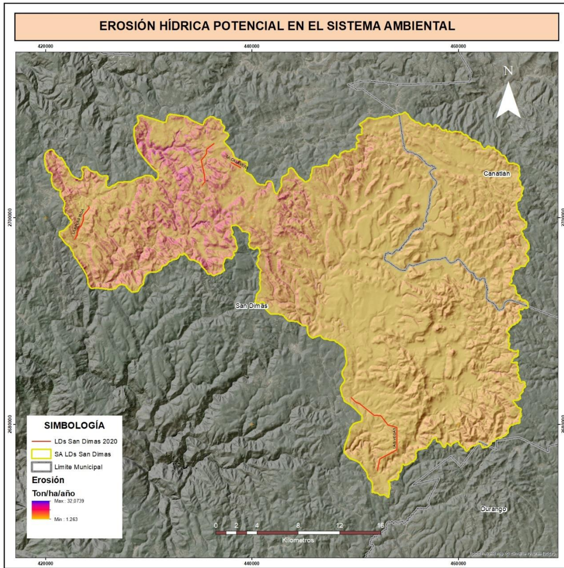
Figura IV-23 Erosión potencial en el SA
