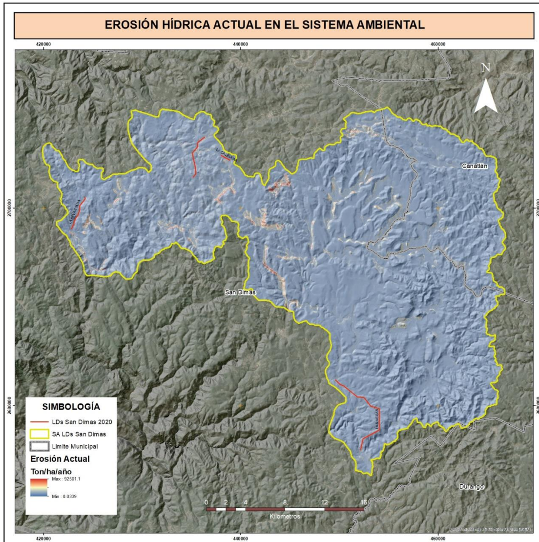
Figura IV-25 Erosión actual en el SA
