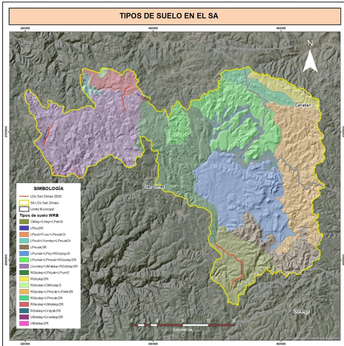
Figura IV-11 Tipos de suelos presentes en el SA
