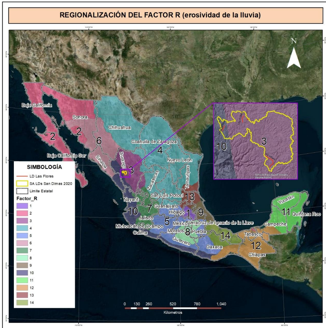
Figura IV-13 Regiones del factor R (Becerra, 1997)
