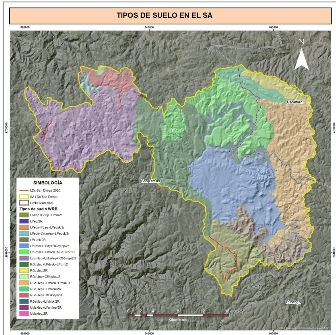
Figura VIII-5 Unidades de suelo
