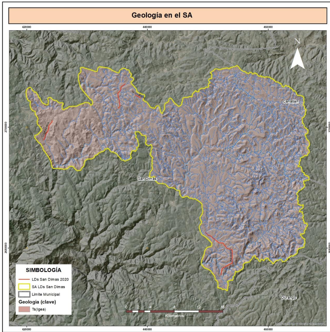
Figura IV-5 Geología del sistema ambiental
