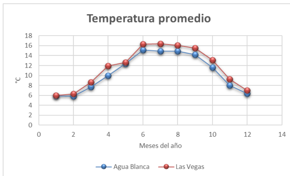
Gráfica IV-1 Temperaturas promedio anual
