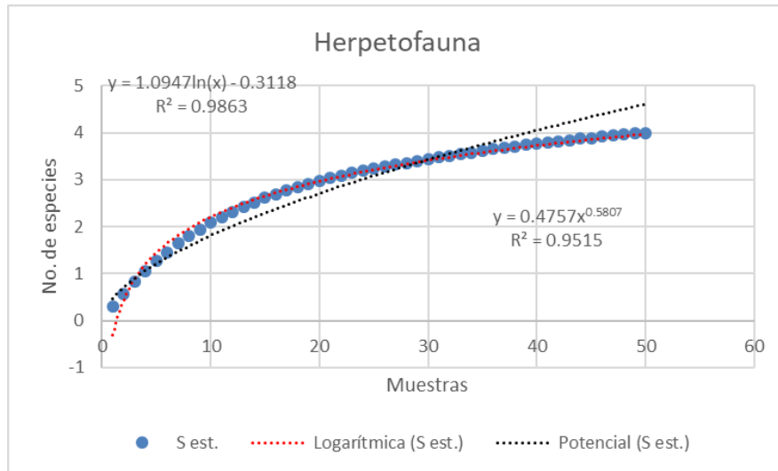
Gráfica IV-7 Curva de acumulación de especies para la herpetofauna
