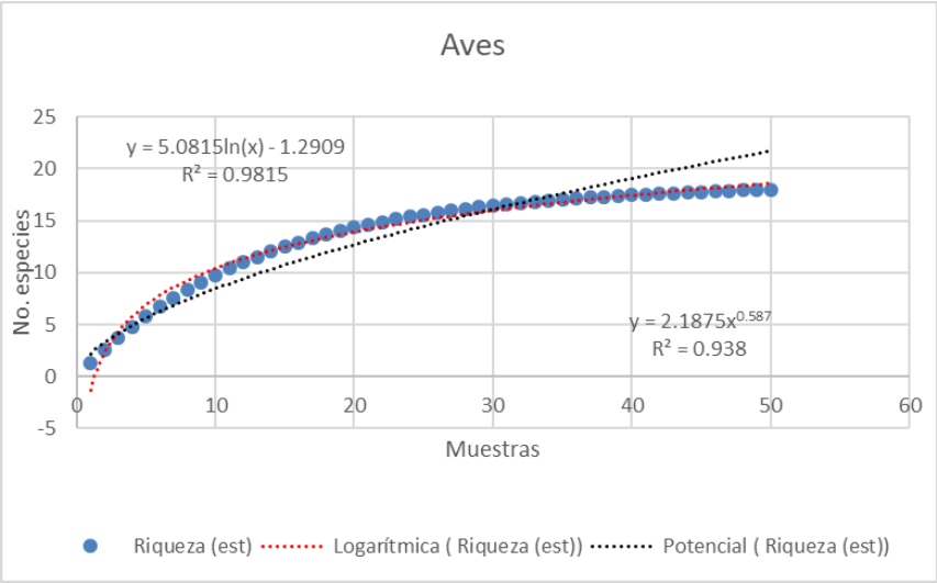
Gráfica IV-8 Estimación de los modelos paramétricos (logarítmica y potencial) conforme a la proporción de especies registradas (S obs) aves
