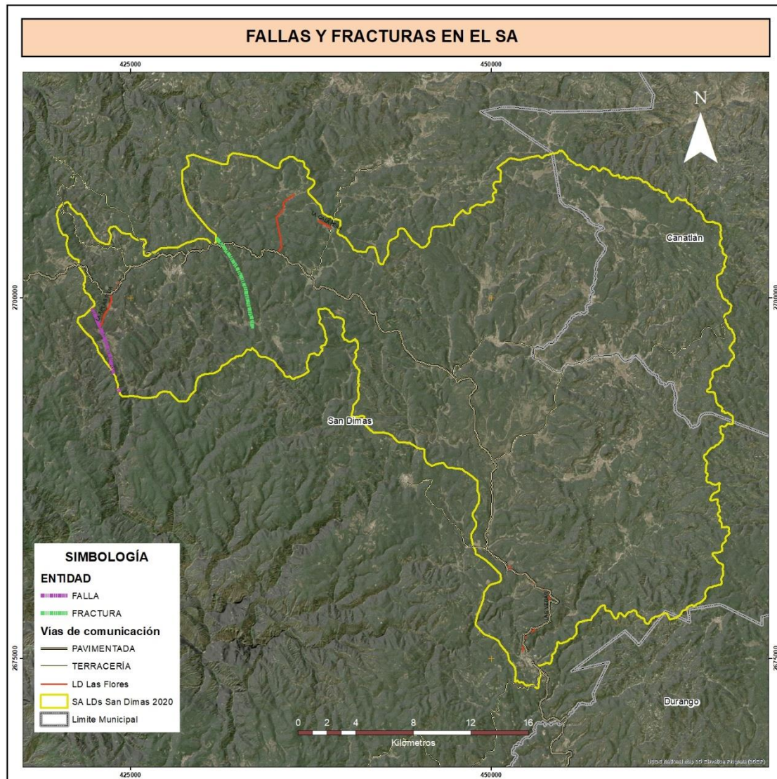
Figura IV-7 Fallas y fracturas existentes en el sistema ambiental
