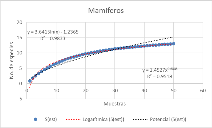
Gráfica IV-9 Estimación de los modelos paramétricos (logarítmica y potencial) conforme a la proporción de especies registradas (S obs) mamíferos
