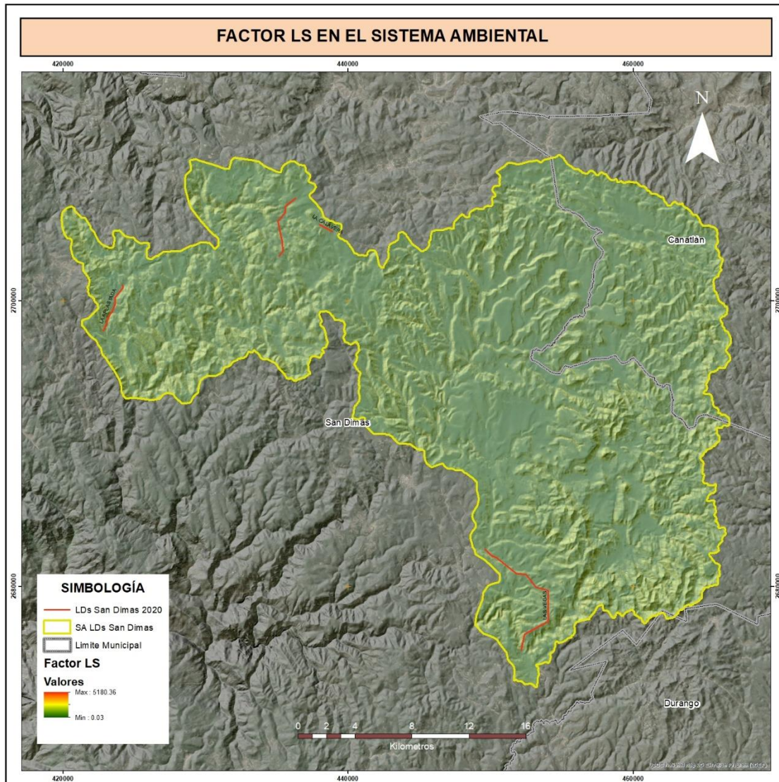
Figura IV-22 Estimación del factor LS para el SA
