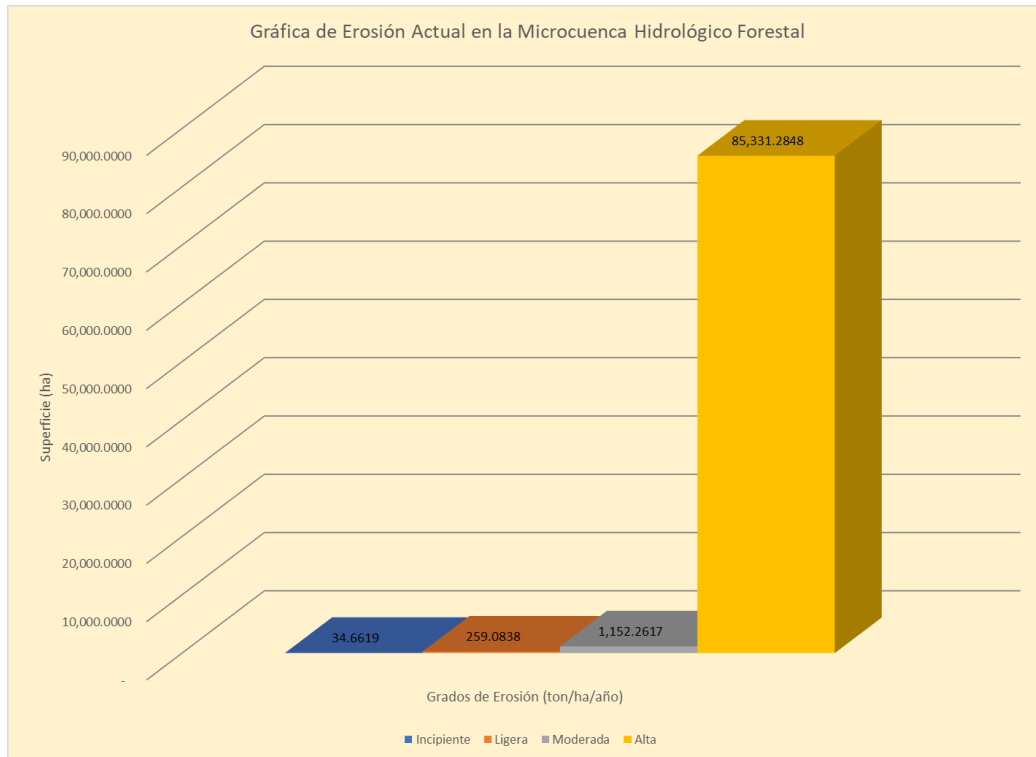
Gráfica IV-4 Erosión actual en el SA (ton*ha*año)
