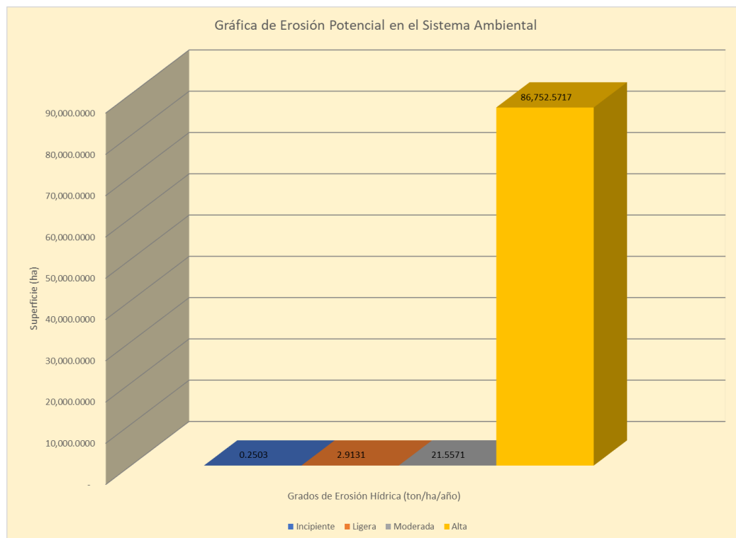
Gráfica IV-3 Erosión potencial en el SA
