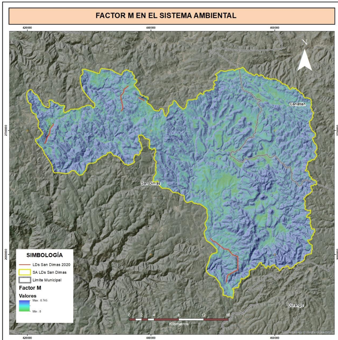
Figura IV-19 Estimación del factor M para el SA
