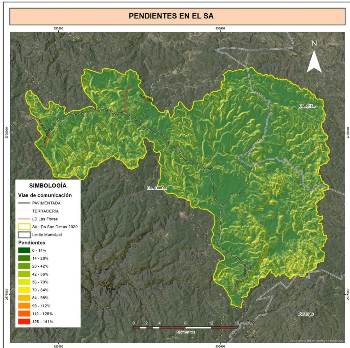
Figura VIII-7 Pendientes
