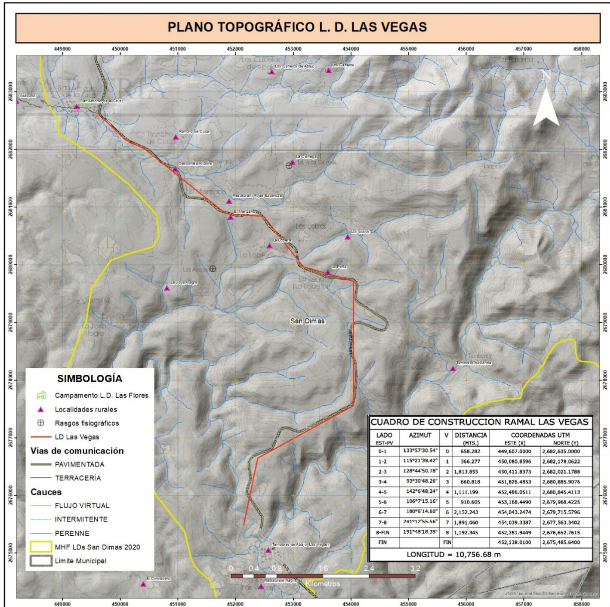
Figura VIII-12 Topografía L. D. Las Vegas
