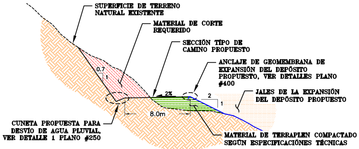
Figura II-6. Sección tipo del camino propuesto
