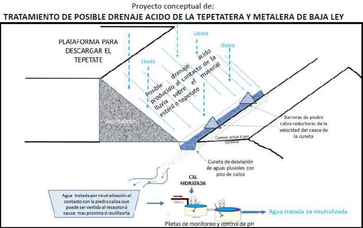
Figura II- 2. Tratamiento de posible drenaje ácido.
