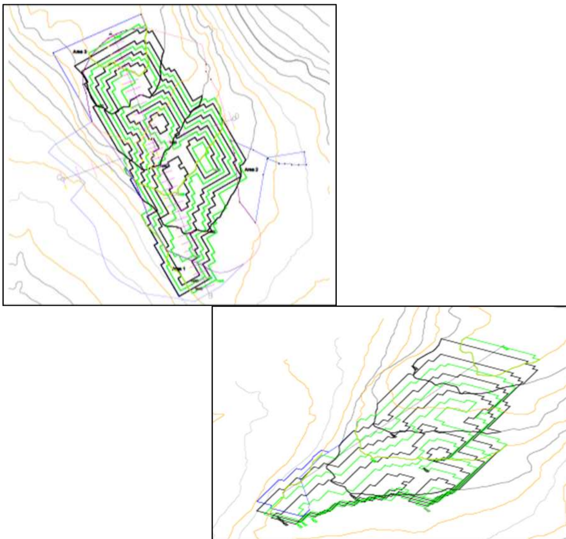
Figura II- 12. Vista esquemática final de las áreas de soporte.
