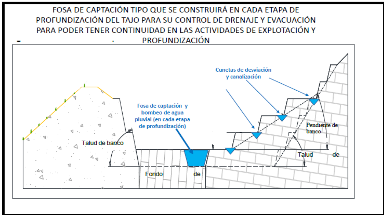
Figura II- 3. Fosa de captación para control y evaluación de drenaje ácido.
