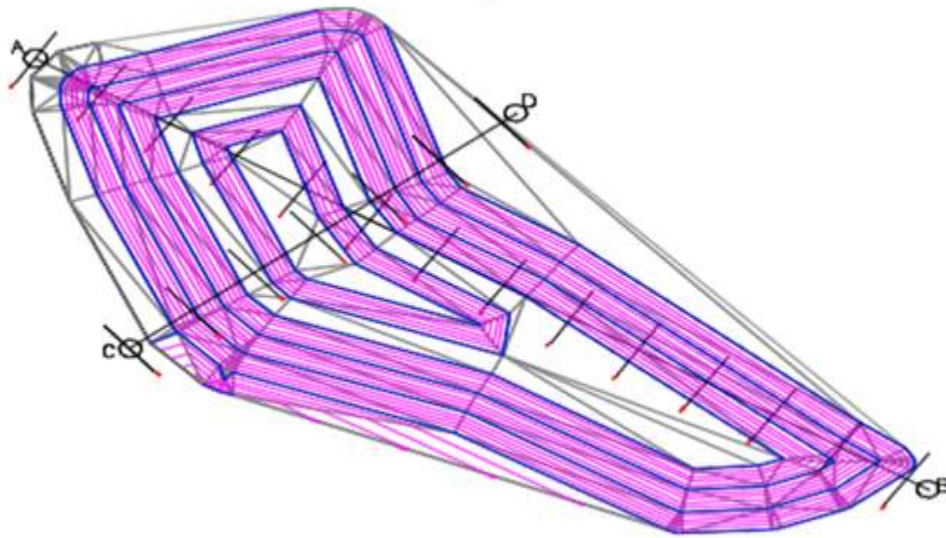
Figura II-10. Vista esquemática final del depósito de mineral de baja ley.
