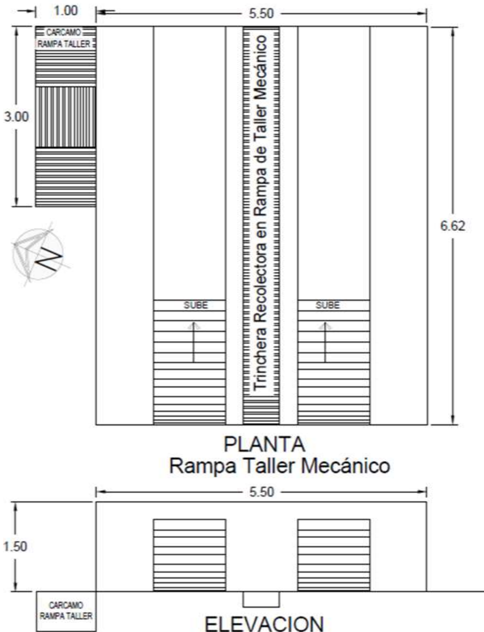
Figura II-15. Arreglo general de rampa taller mecánico y cárcamos para colecta de residuos Patio de Maniobras Taller.
