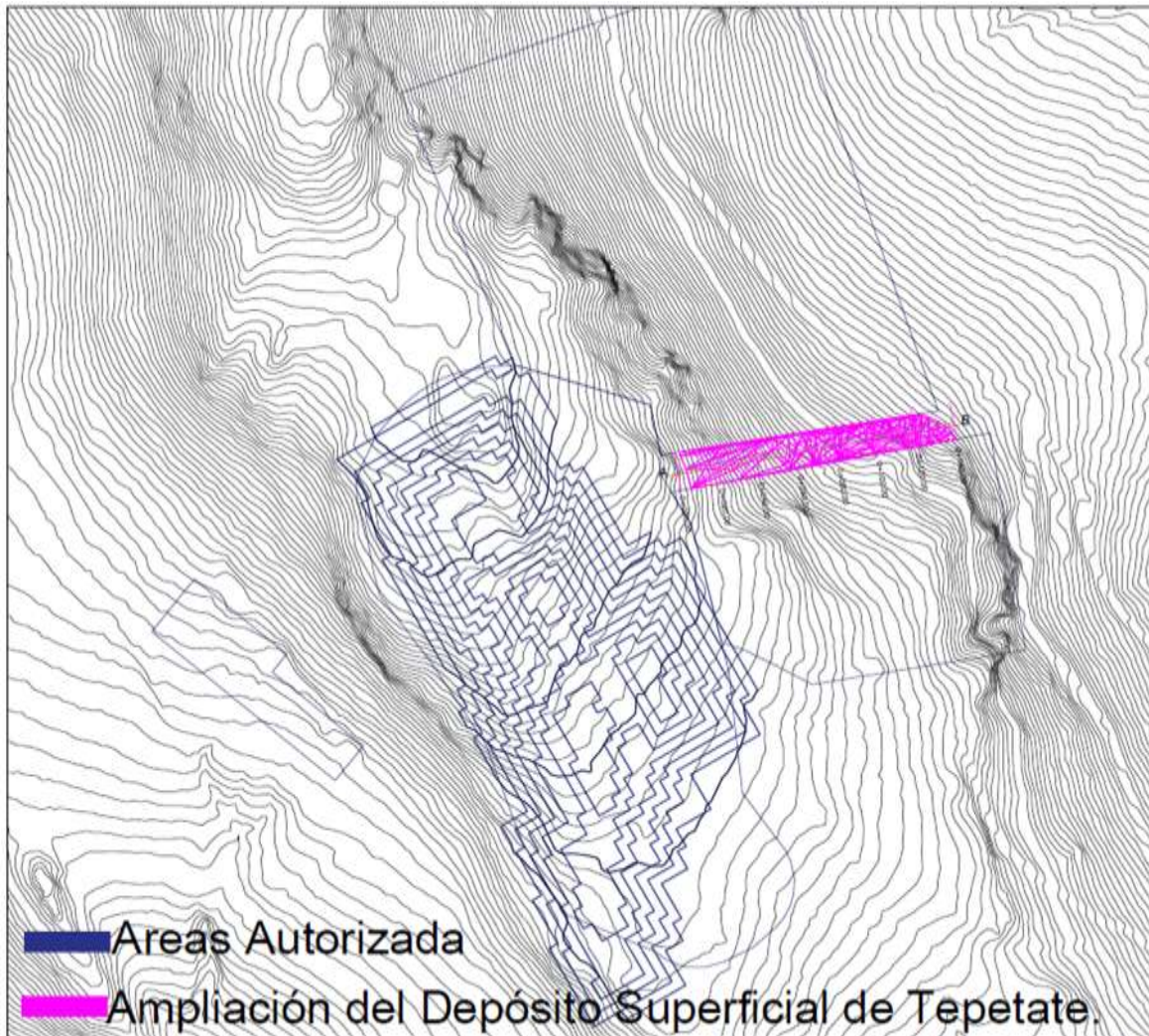
Figura II-8. Vista esquemática final del depósito superficial de tepetate.
