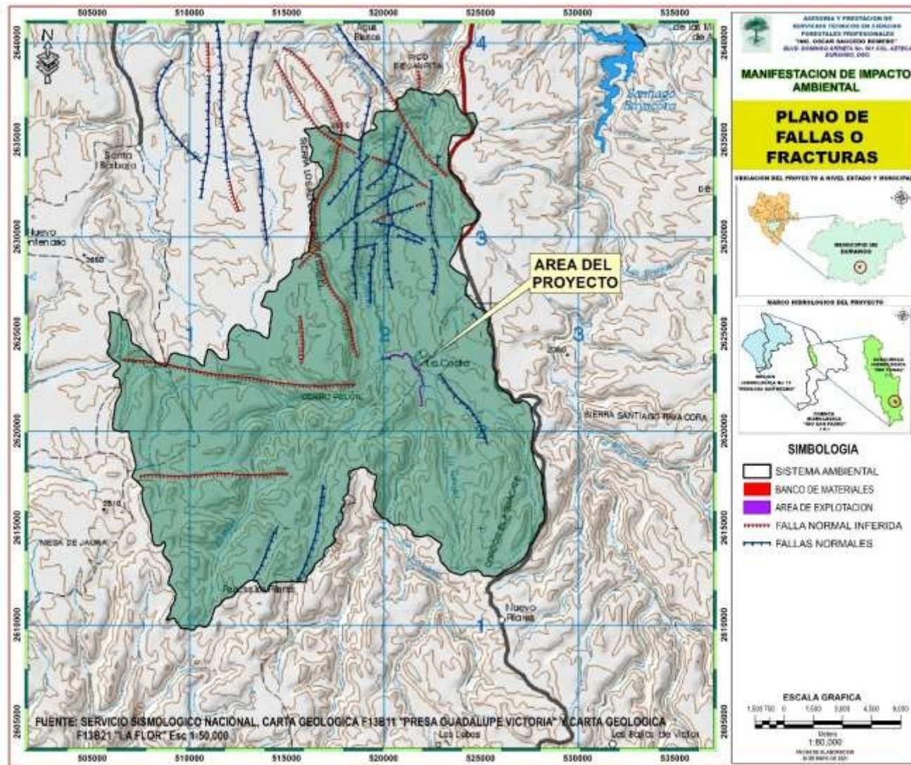
Figura 4.17. Fallas geológicas dentro del SA, INEGI
