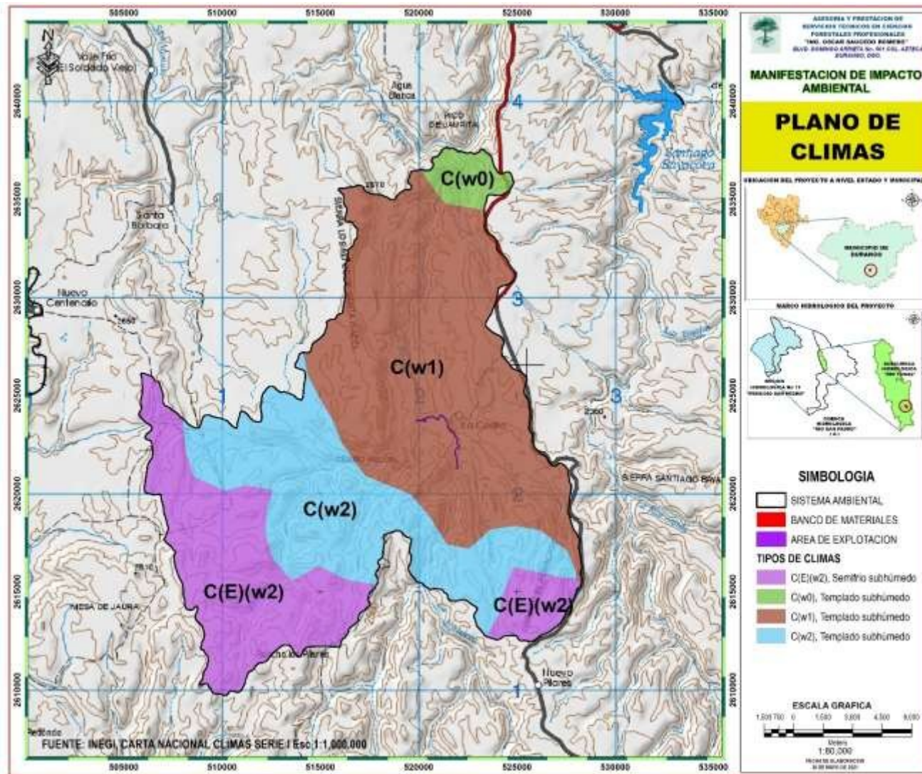
Figura 4.3. Tipos de clima dentro del SA según Clasificación de Köppen (INEGI)
