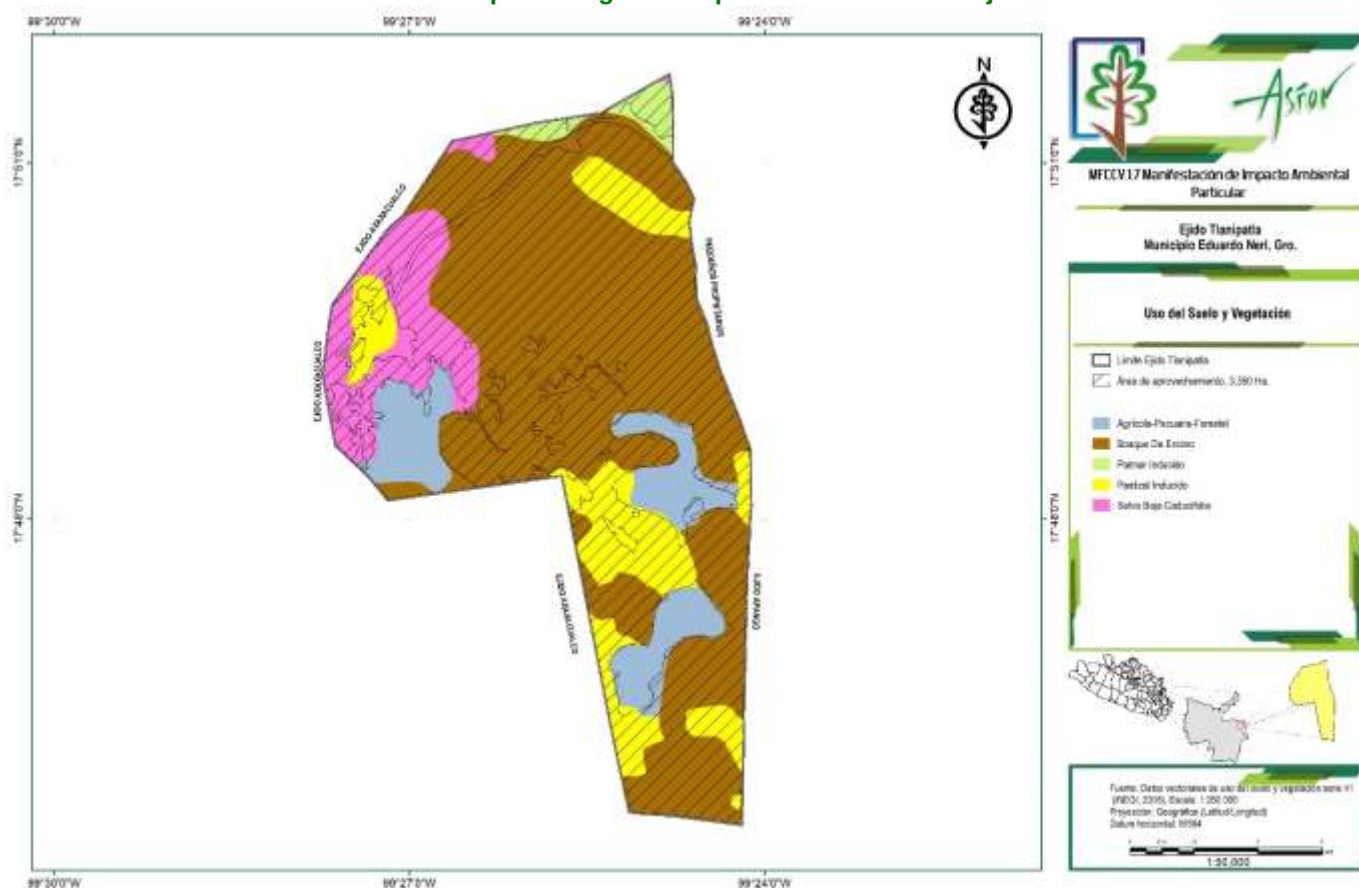
Plano 8.- Tipo de vegetación presente dentro del Ejido.
