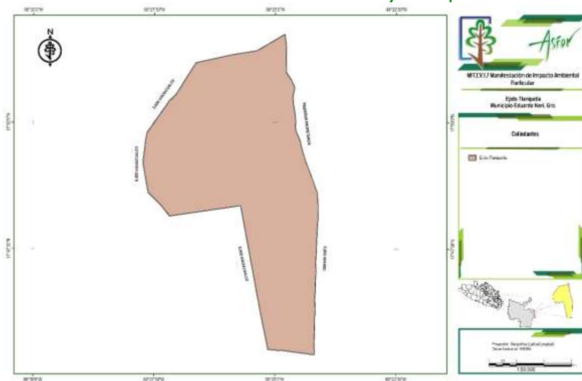
Plano 2.- Colindancias del ejido Tlanipatla.
