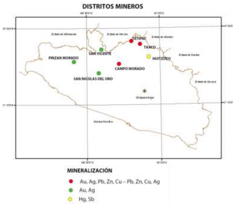
Figura 6.- Distritos Mineros en el Estado de Guerrero
