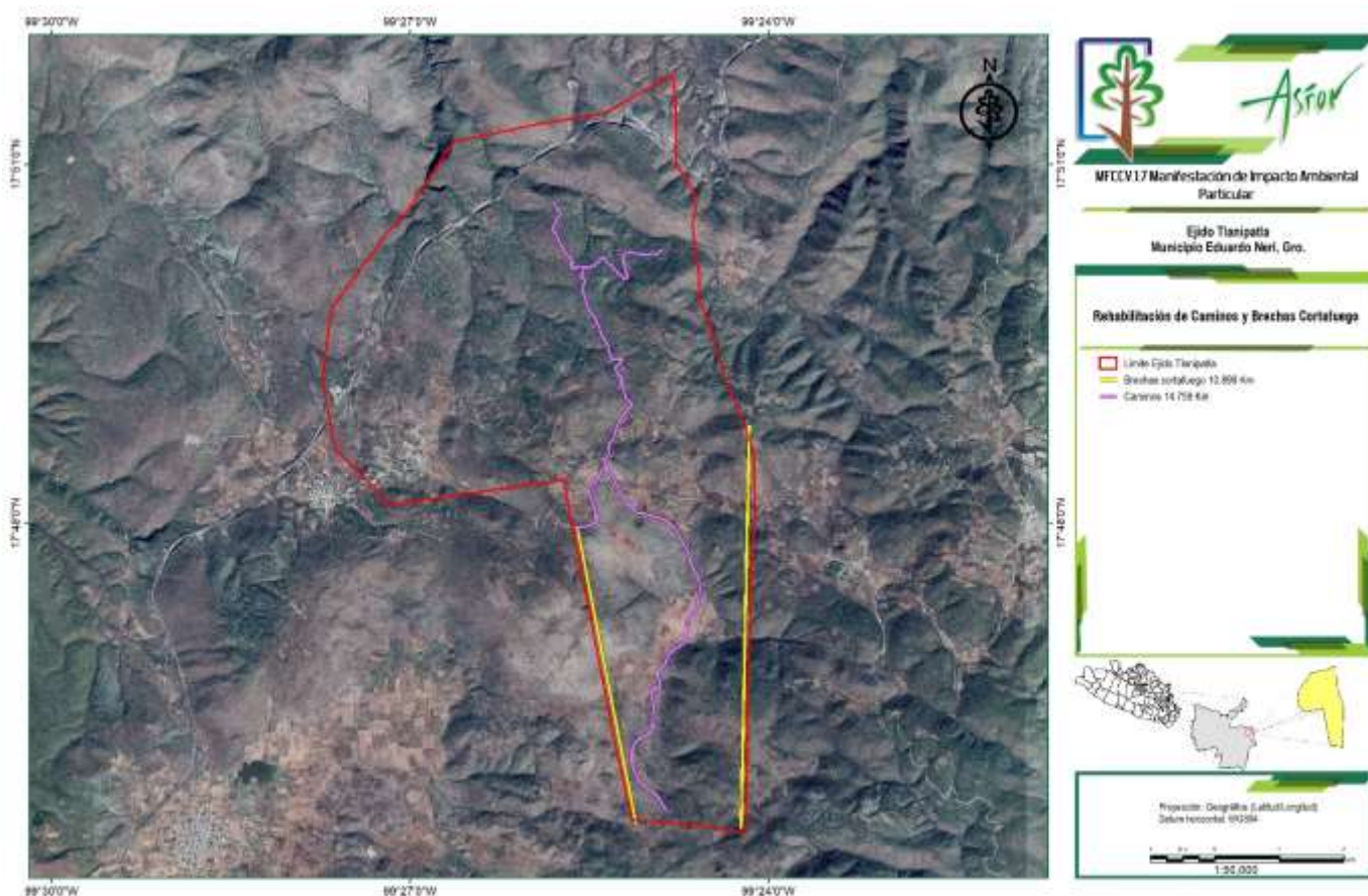
Plano 4.- Plano de caminos a rehabilitar.
