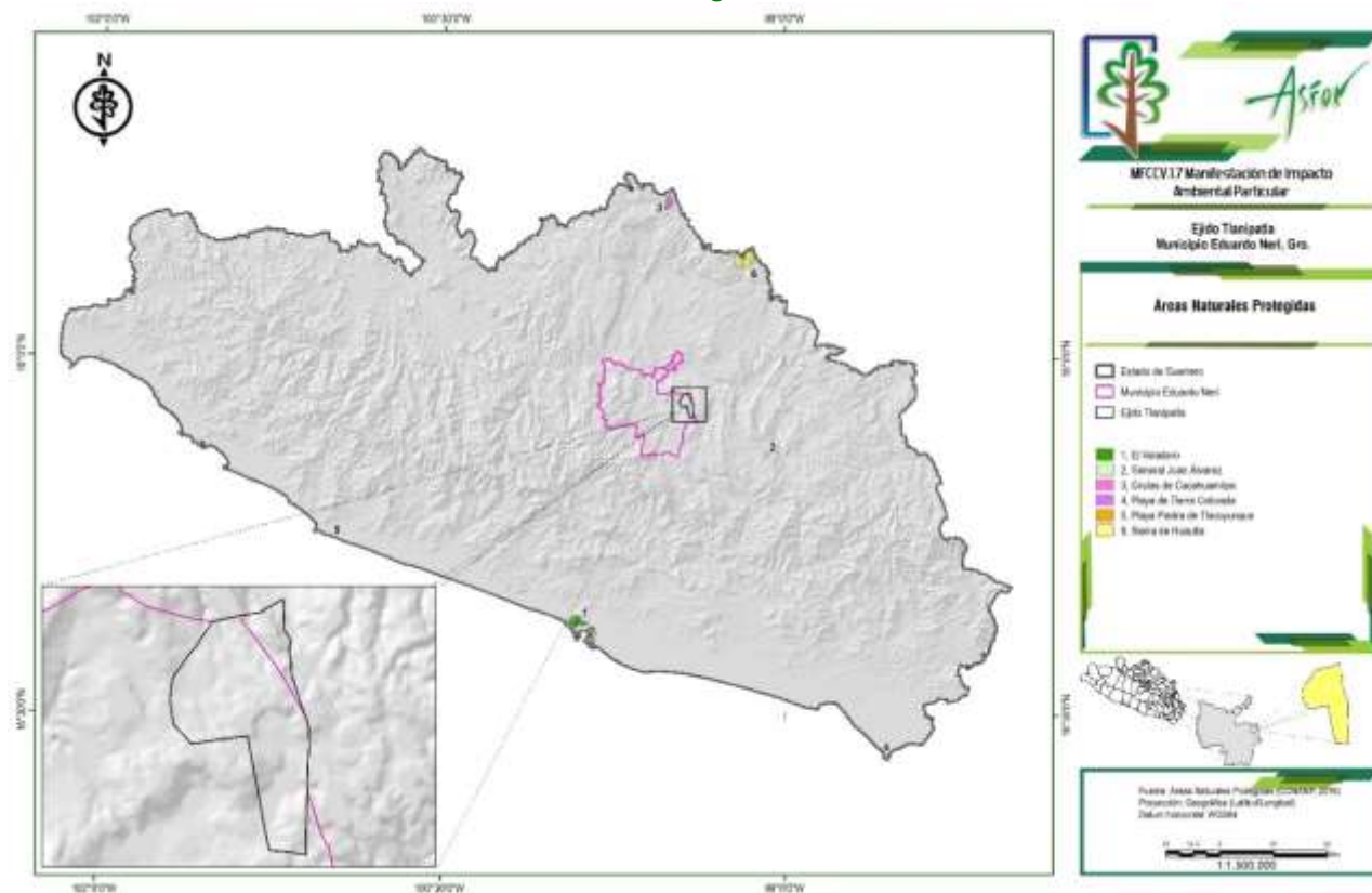
Plano 17.- Áreas naturales Protegidas en el estado de Guerrero.
