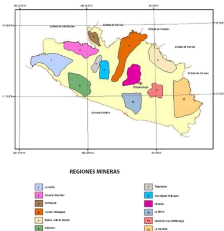
Figura 5.- Regiones Mineras en el Estado de Guerrero
