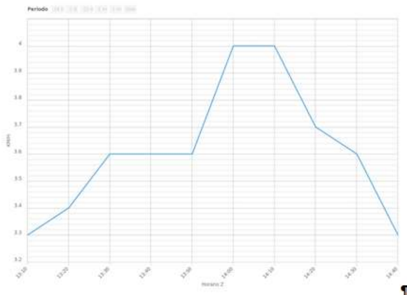
Gráfico 2.- Velocidad del viento.
