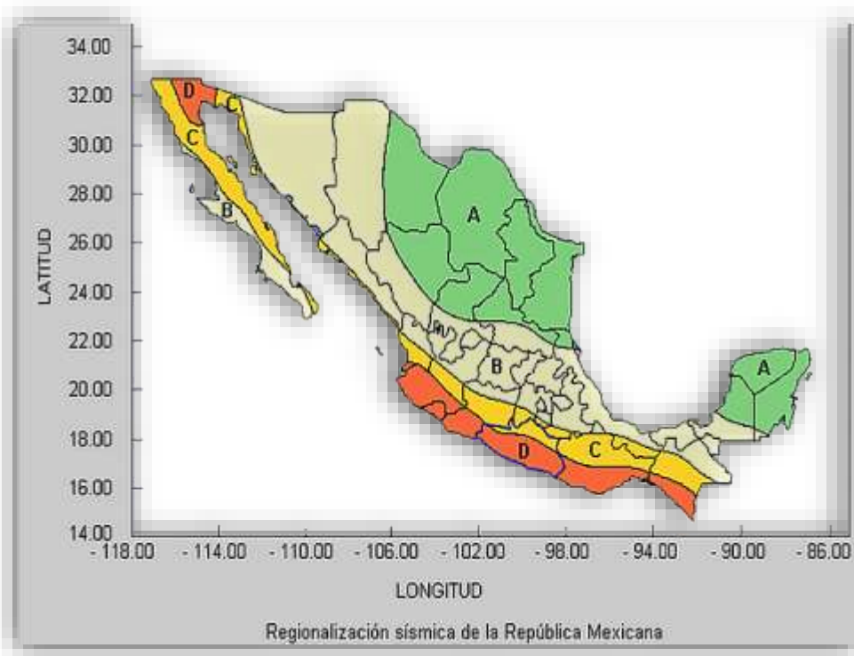
Figura 4.- Regionalización sísmica de la República Mexicana.
