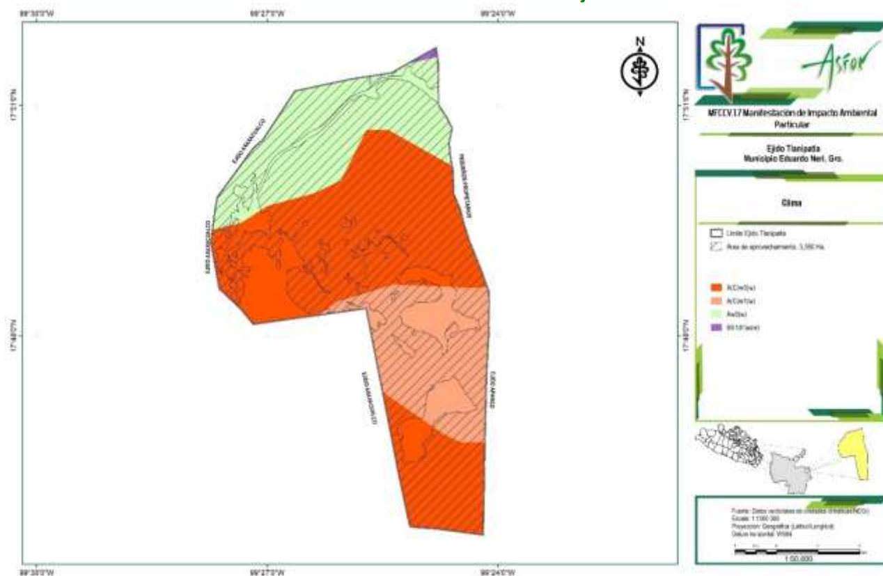
Plano 27.- Plano de climas en el ejido.
