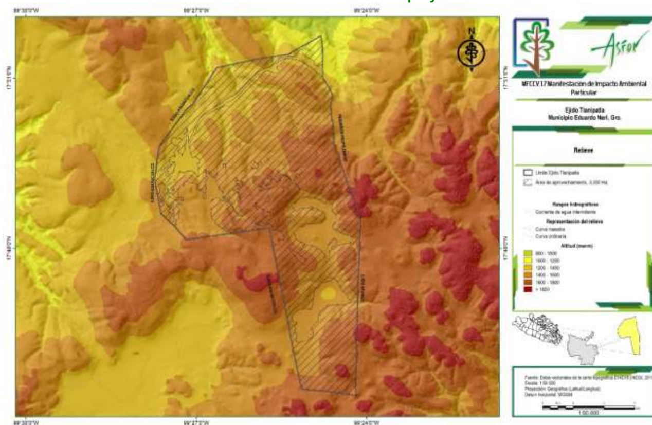
Plano 30.- Relieve en el sitio del proyecto.
