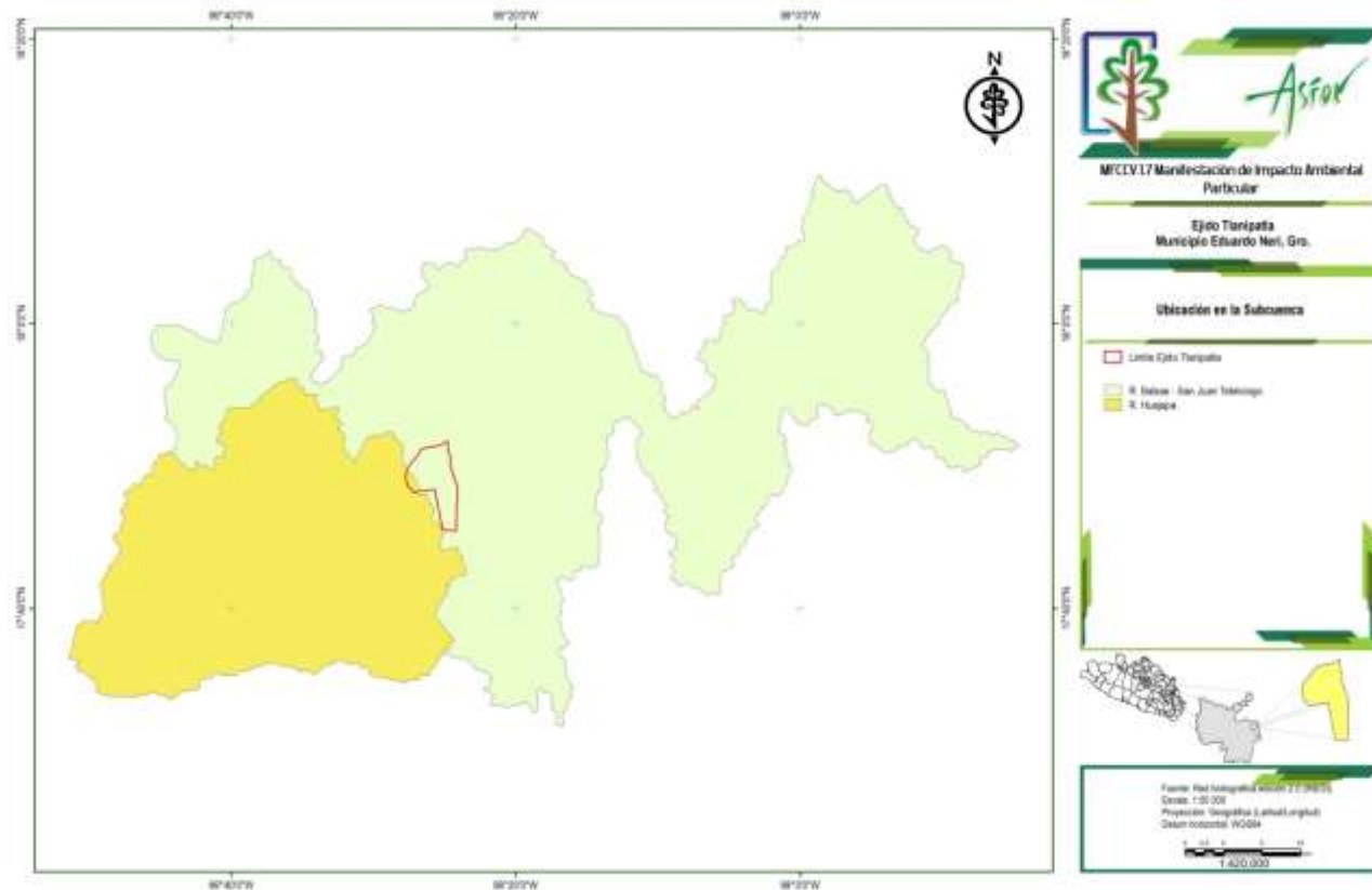
Plano 21.- Ubicación de la superficie de aprovechamiento en las Subcuencas R. Balsas- San Juan Tetelcingo y R. Huajapa.
