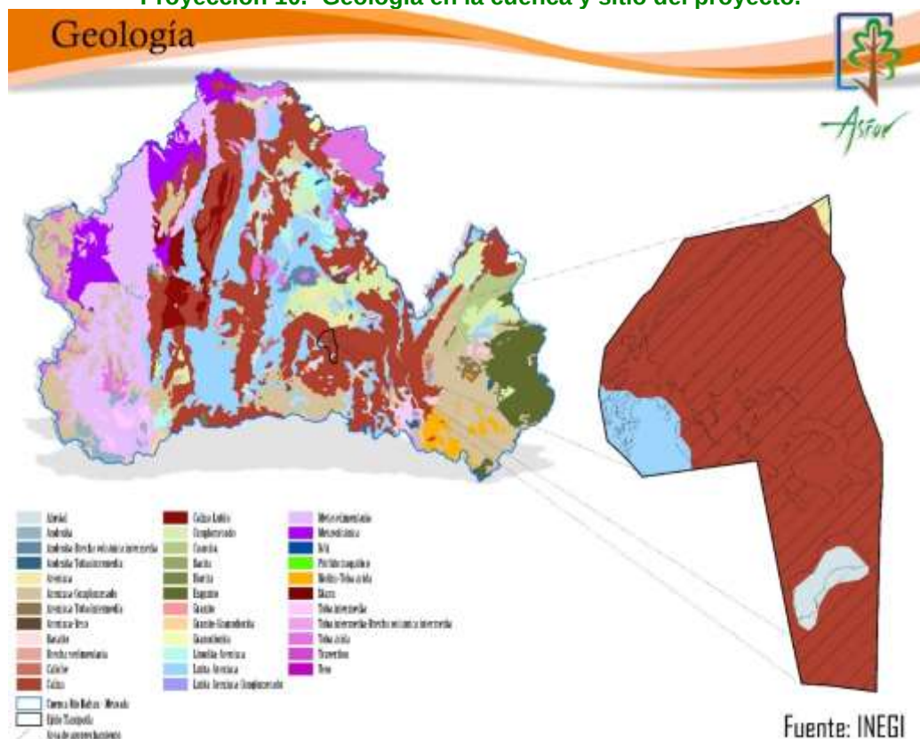
Proyección 10.- Geología en la cuenca y sitio del proyecto.
