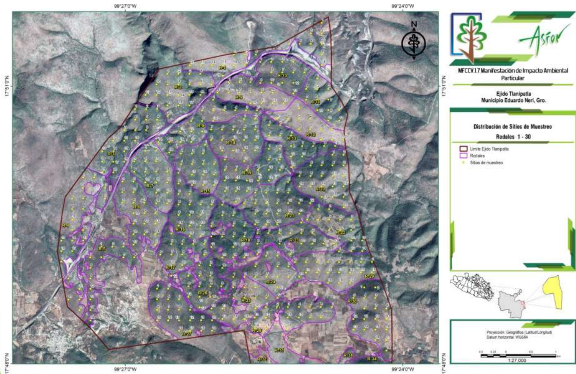
Plano 13.- Distribución de los sitios de muestreo en los rodales 1 al 30 en el diseño del proyecto.
