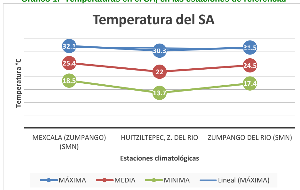
Gráfico 1.- Temperaturas en el SA, en las estaciones de referencia.
