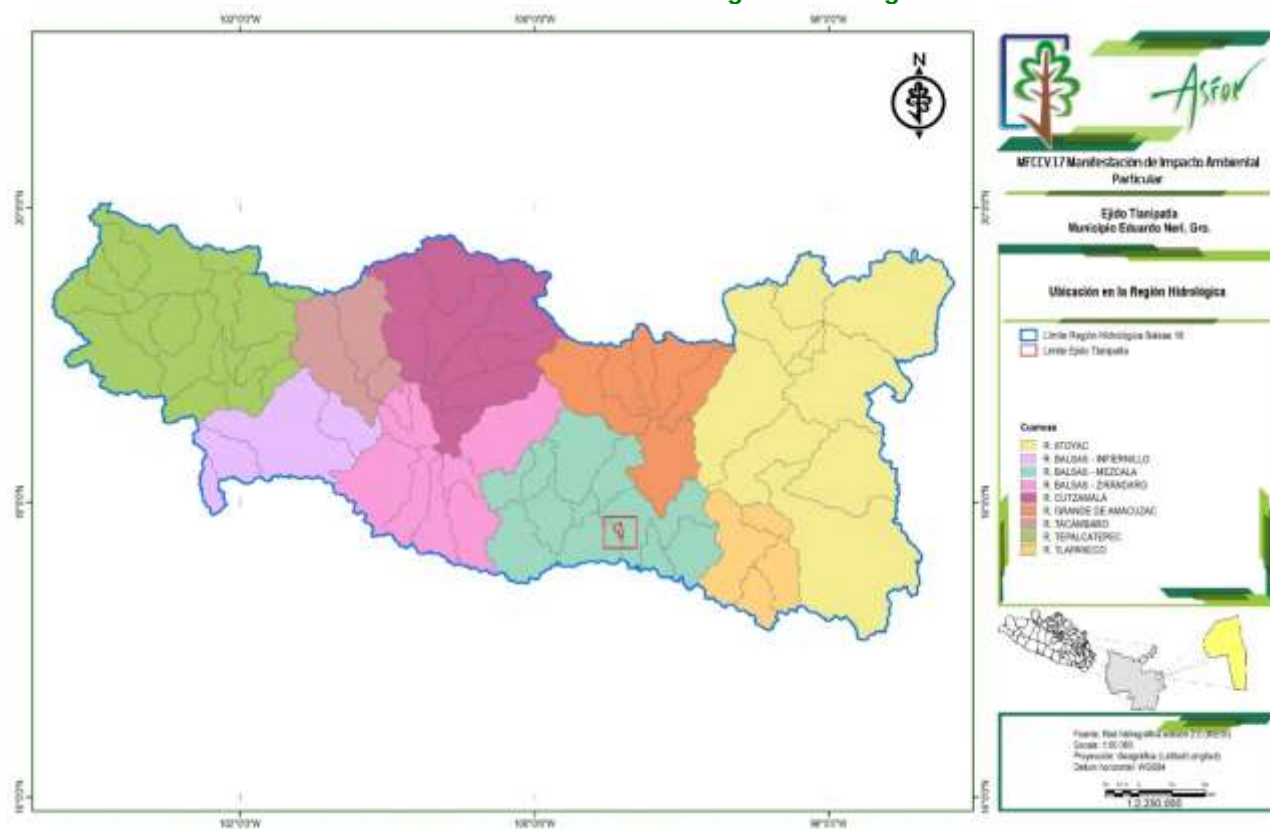
Plano 24.- Ubicación dentro de la Región Hidrológica No. 18.
