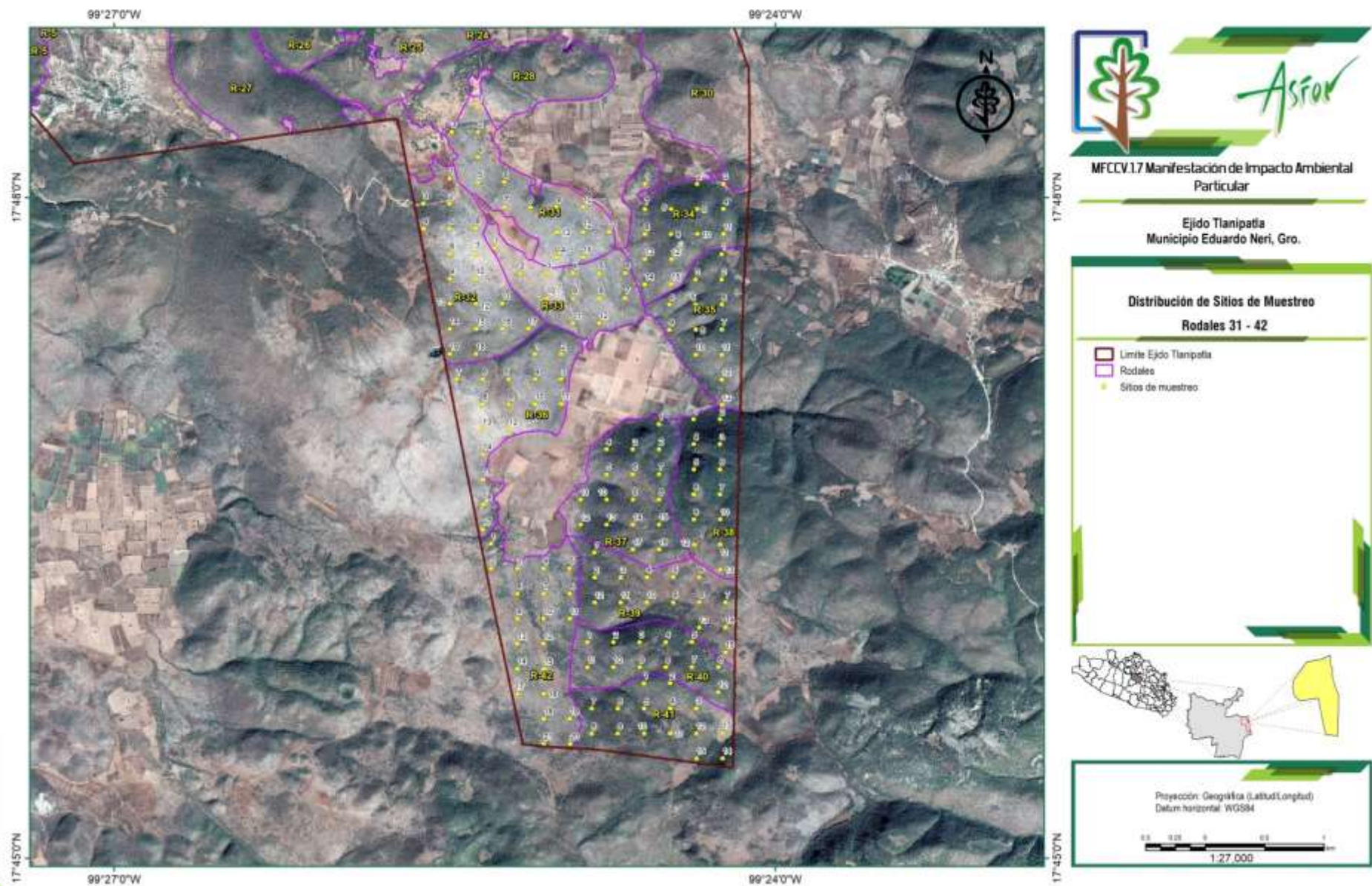
Plano 14.- Distribución de los sitios de muestreo en los rodales 31 al 42 en el diseño del proyecto.
