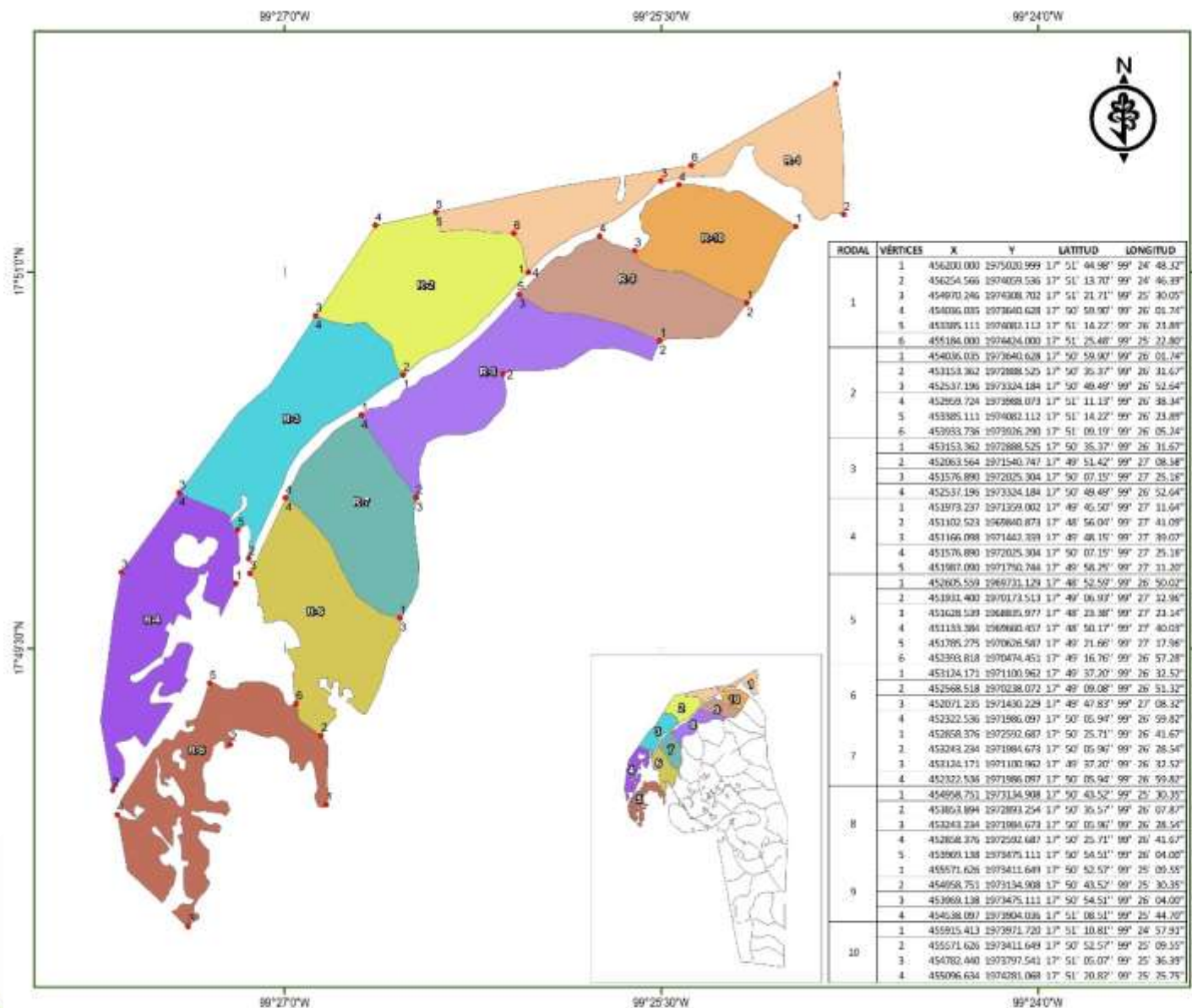
Plano 9.- Ubicación y localización de los rodales del 1 al 10.
