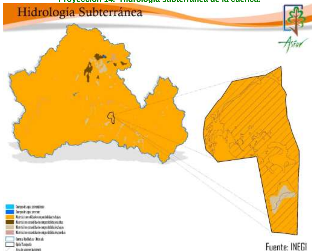
Proyección 14.- Hidrología subterránea de la cuenca.
