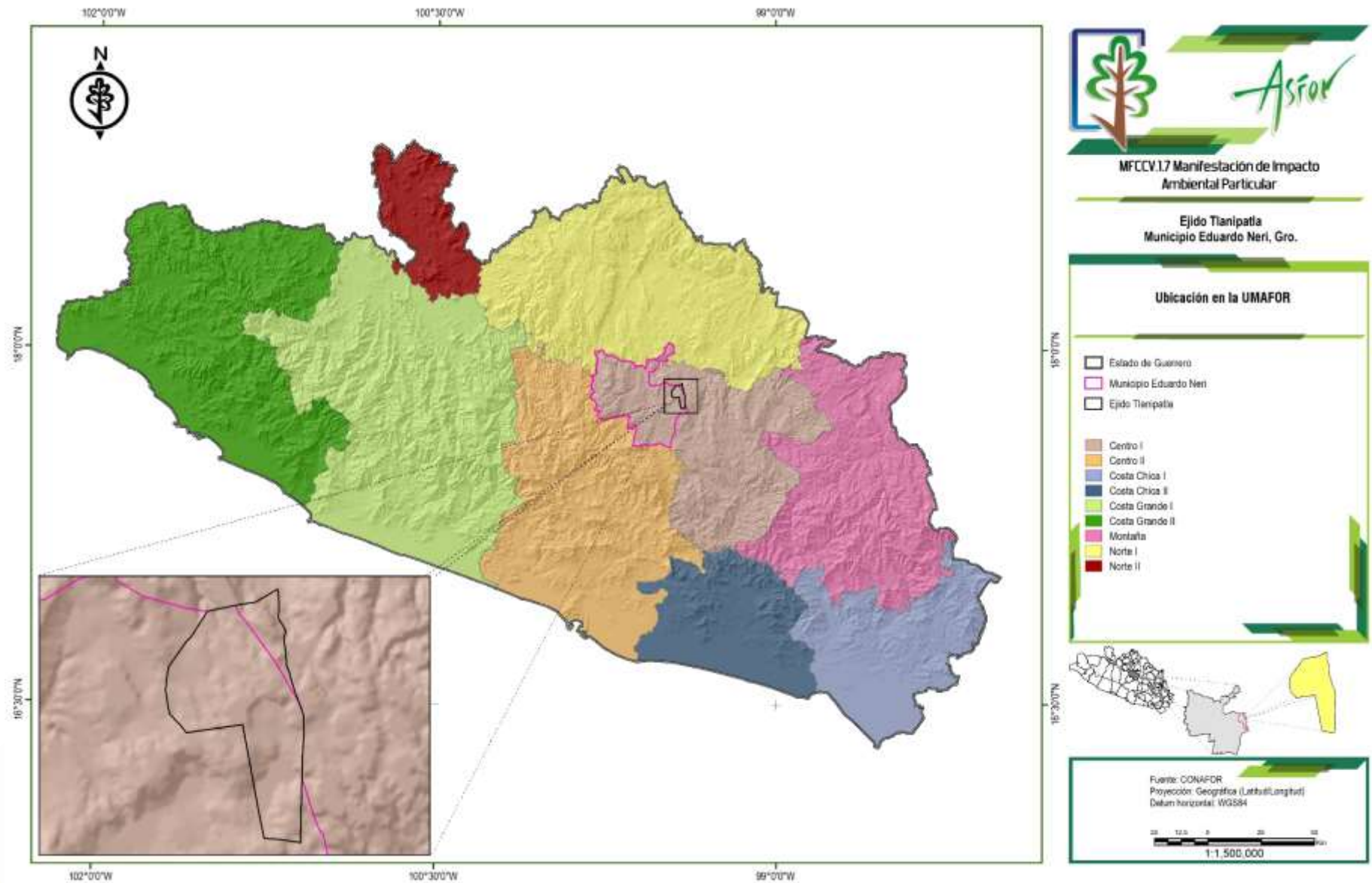
Plano 16.- Ubicación del ejido dentro de la UMAFOR.
