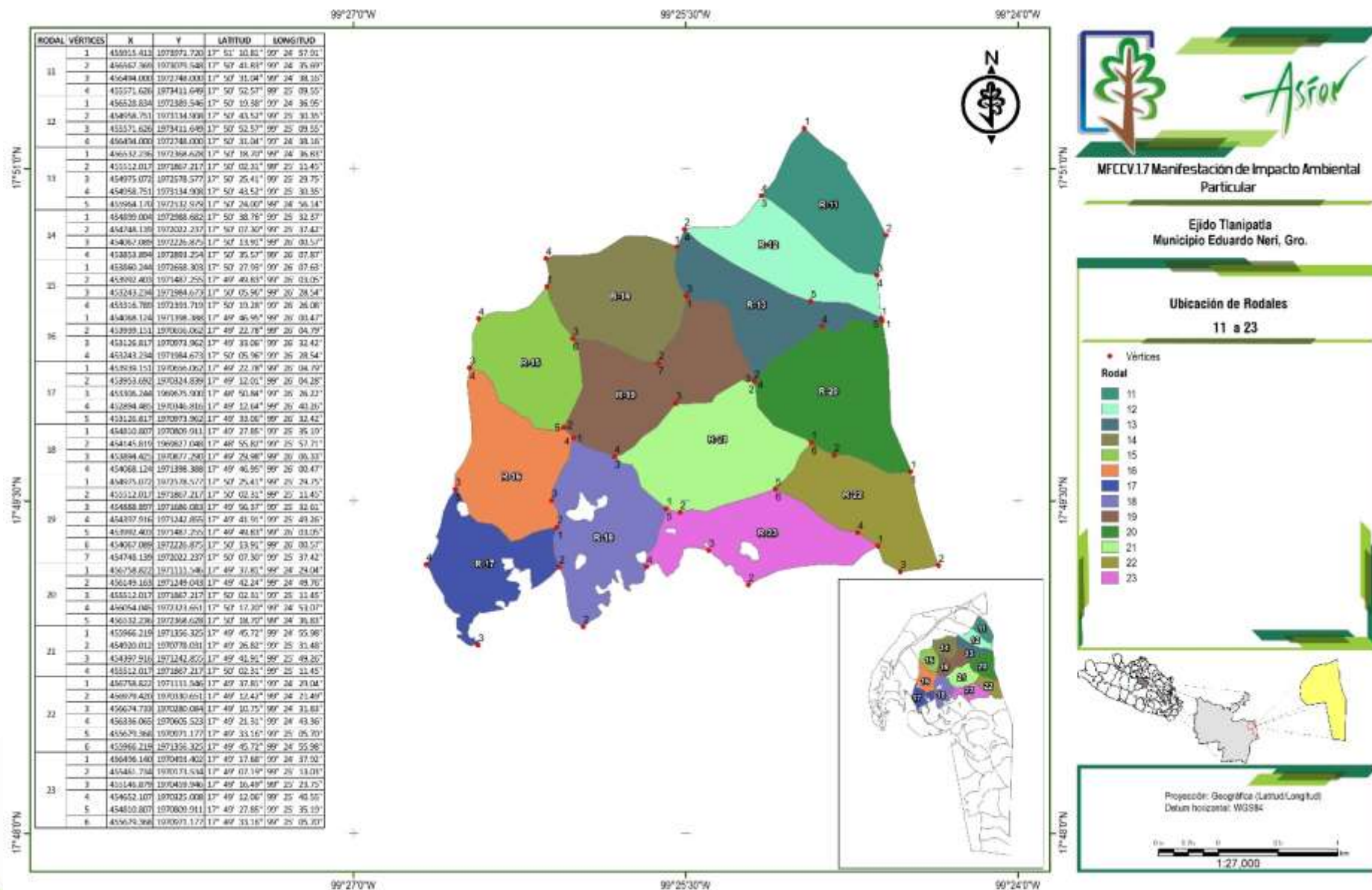
Plano 10.- Ubicación y localización de los rodales del 11 al 23.
