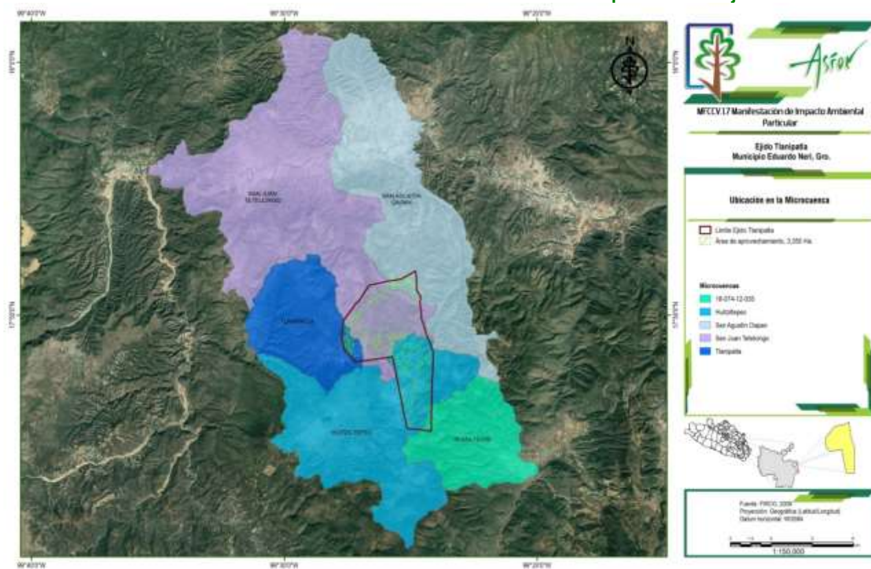
Plano 22.- Identificación de las microcuencas sobre las que incide el ejido.
