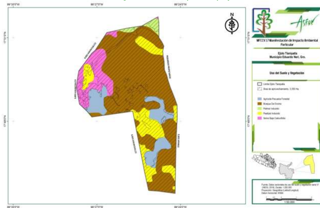
Plano 32.- Vegetación dentro del predi del proyecto.
