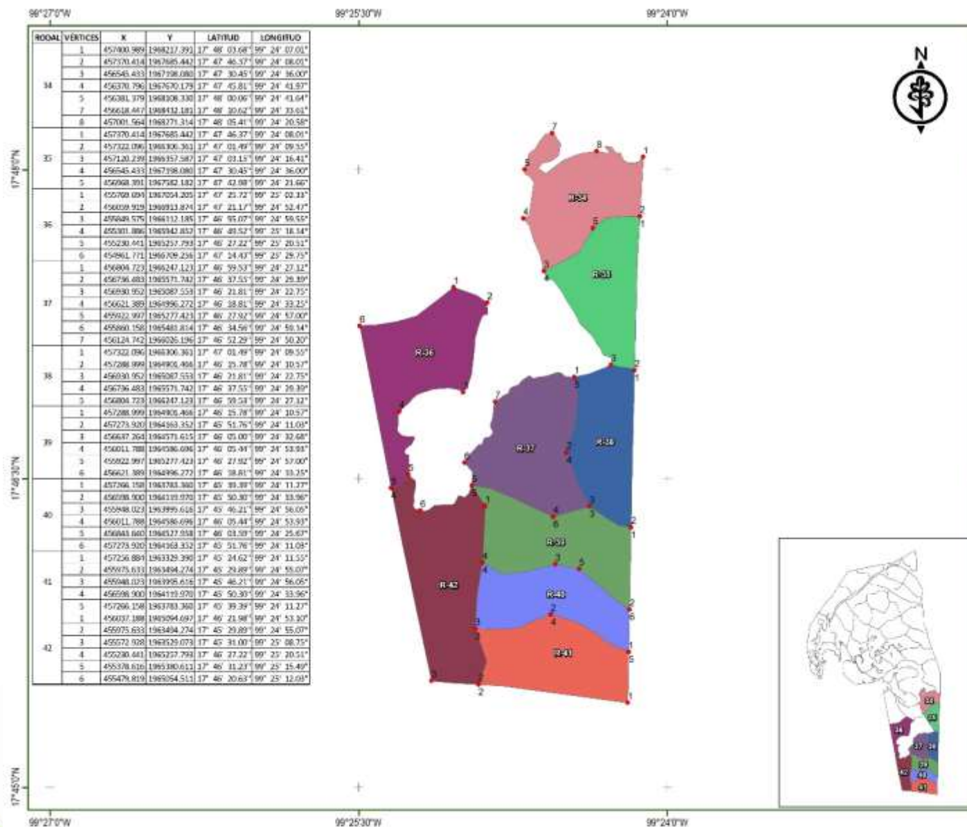
Plano 12.- Ubicación y localización de los rodales del 34 al 42.
