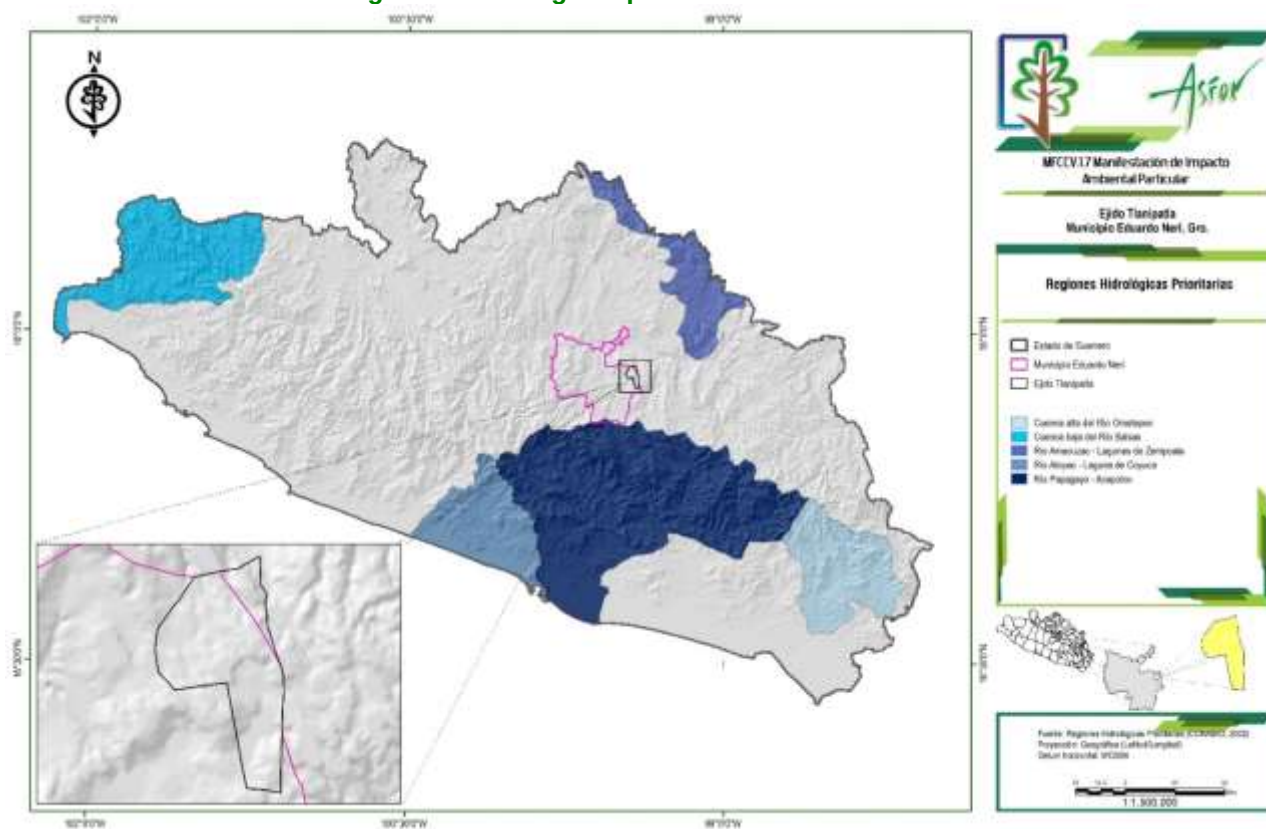
Plano 18.- Regiones hidrológicas prioritarias en el estado de Guerrero.
