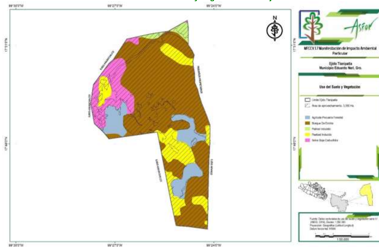
Plano 26.- Uso de suelo y vegetación en el ejido.
