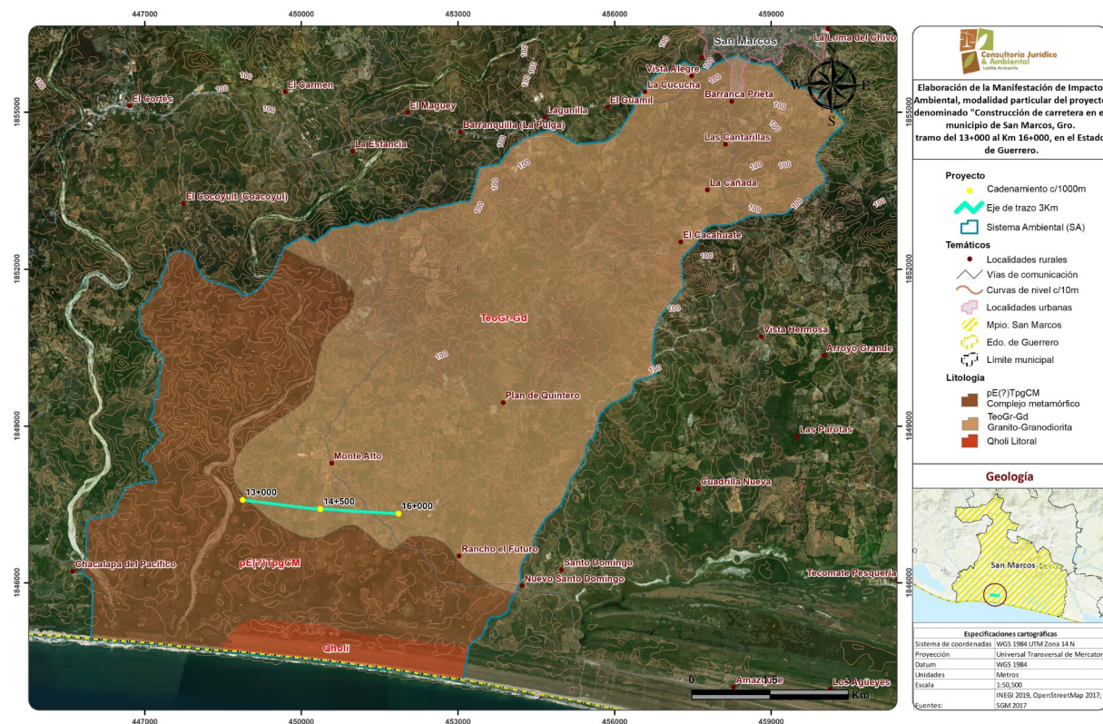
Figura IV.4. Geología dentro del SA.
