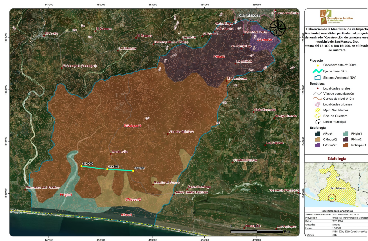
Figura IV.6. Mapa. Edafología presente en el SA.
