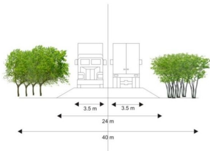
Figura II.1 Sección tipo para la construcción del camino.
