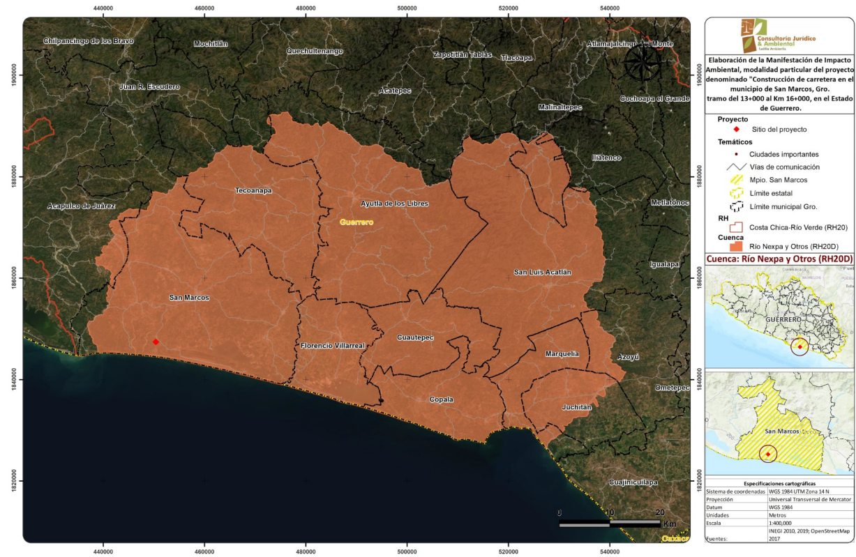
Figura IV.8. Cuenca hidrológica del SA
