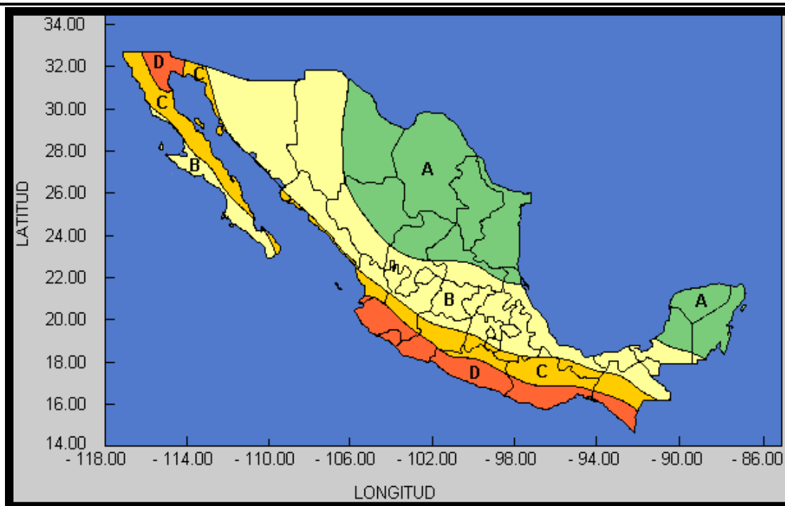
Figura IV.5. Regionalización sísmica de la República Mexicana.
