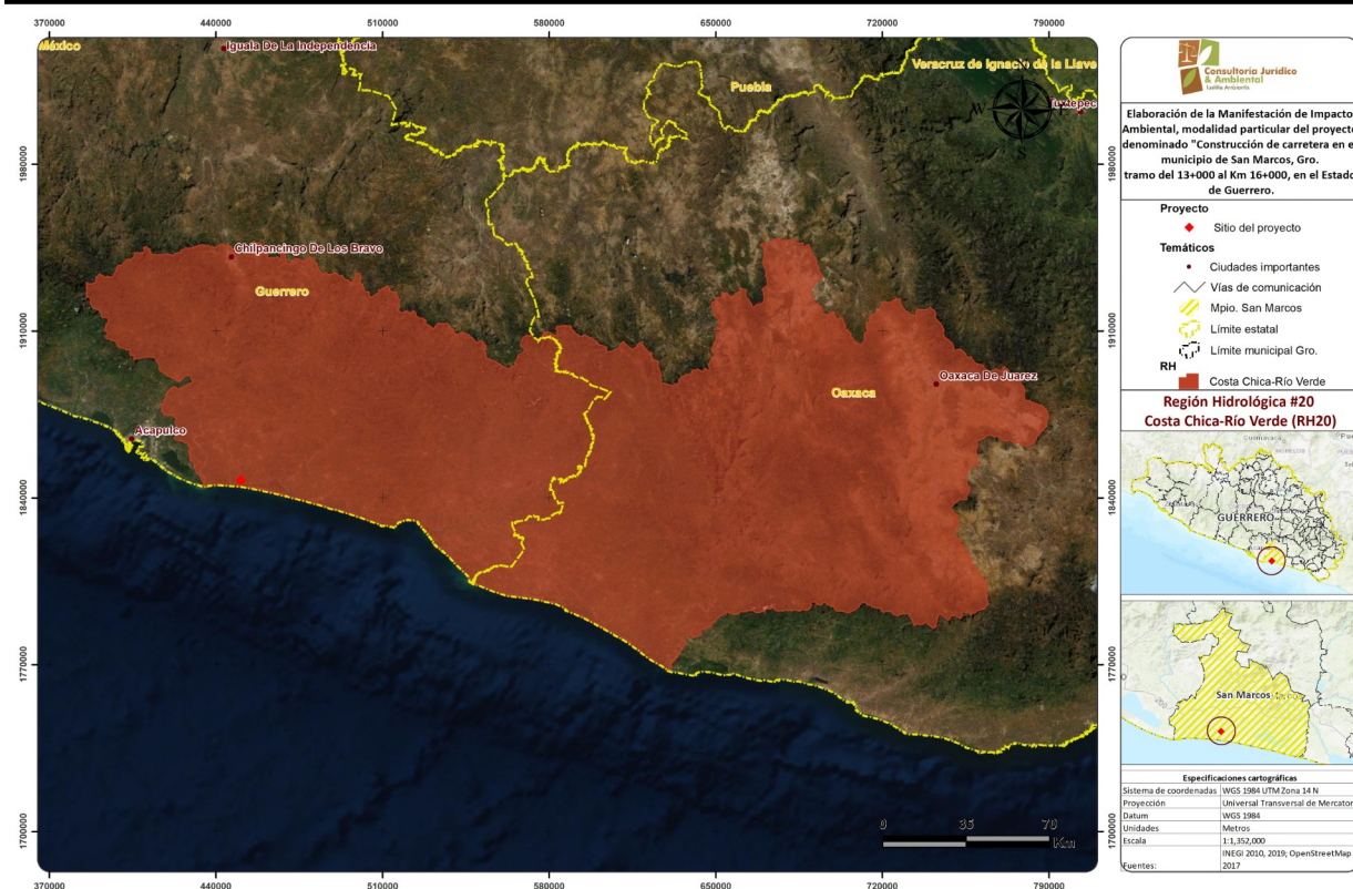
Figura IV.7. Región hidrológica del SA
