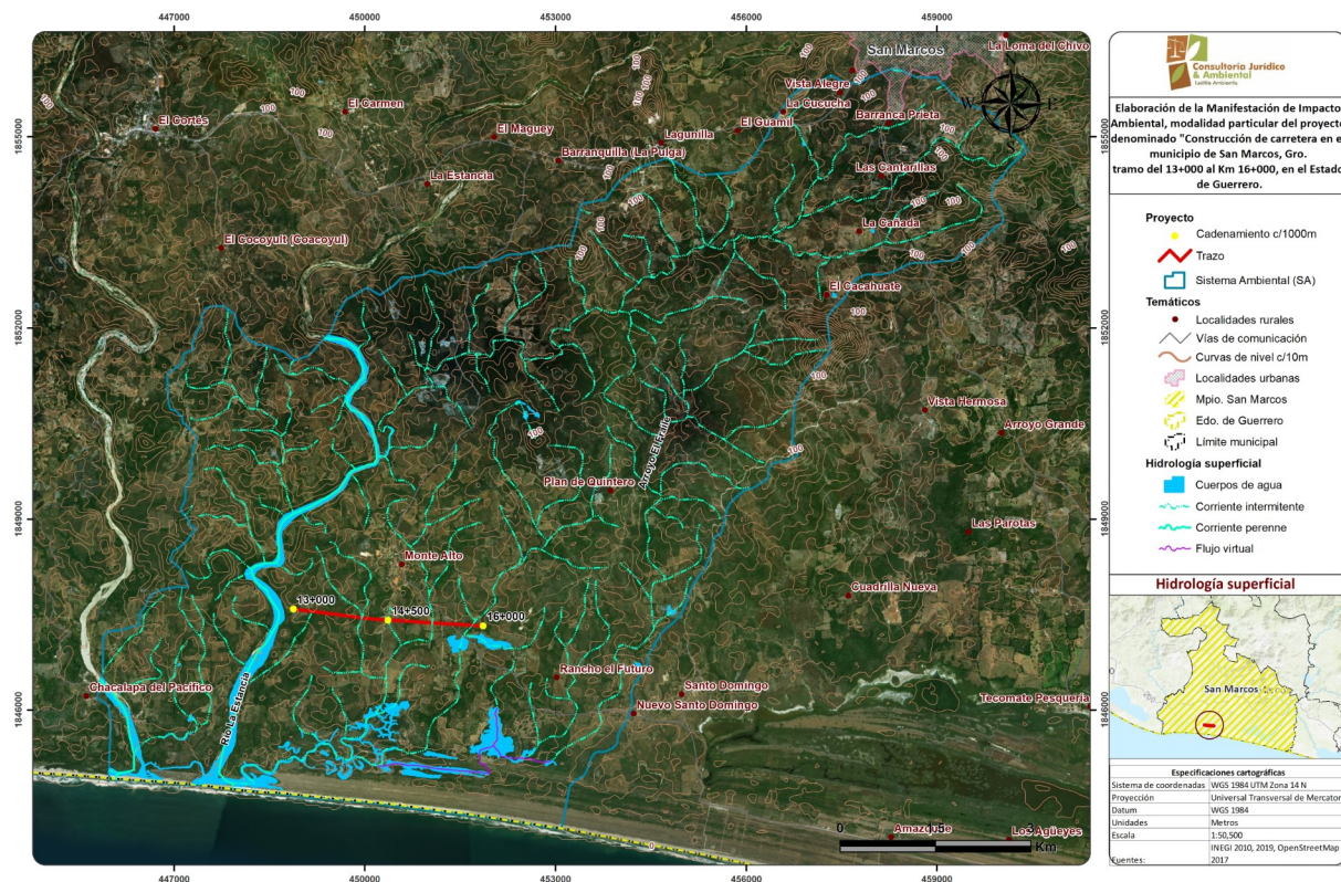
Figura IV.9. Hidrología superficial en el SA
