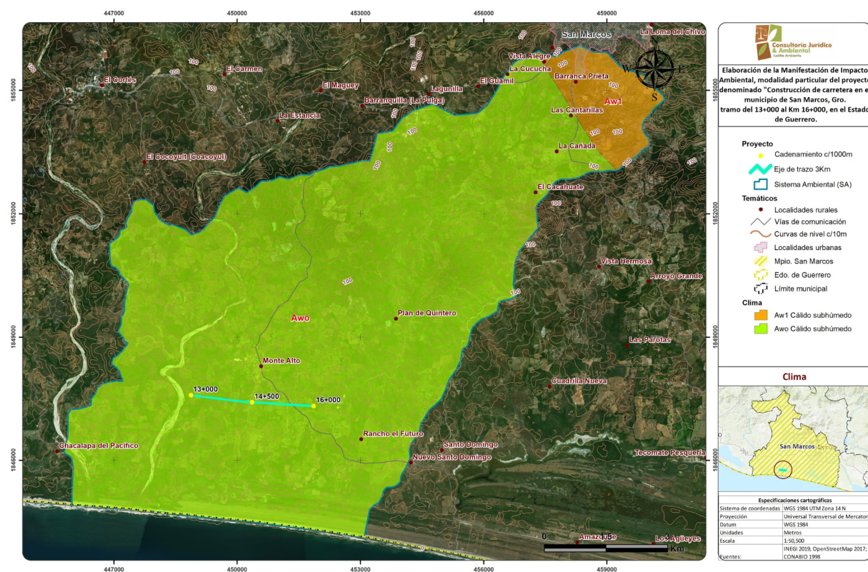
Figura IV.2. Clima dentro del SA.
