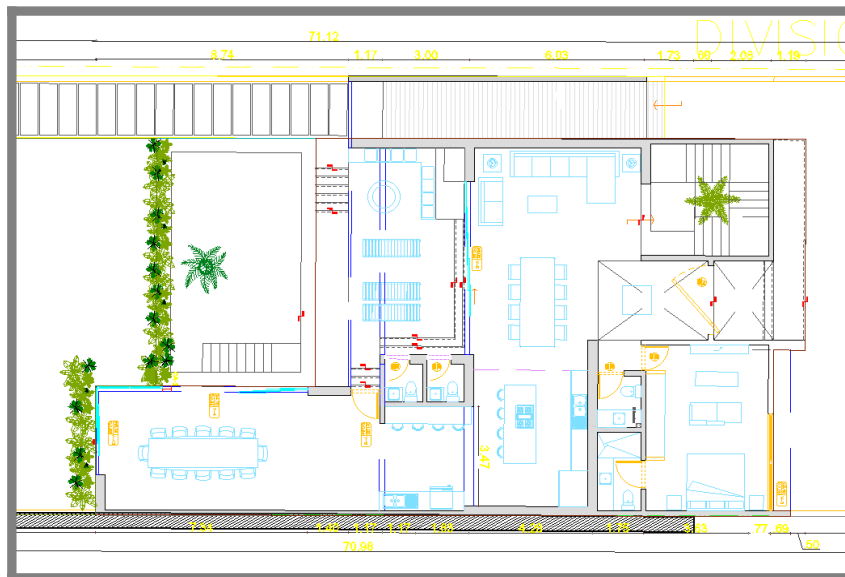
Figura II.3 Detalle del proyecto. Casa Principal, planta baja.
