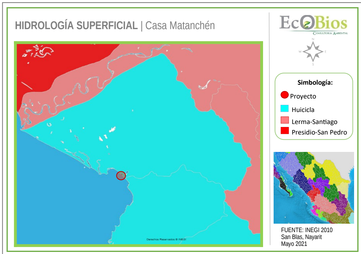
Figura IV.11 Hidrología superficial
