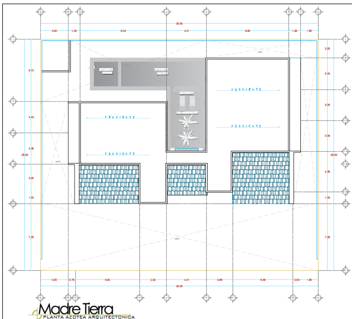
Ilustración II-4. Planta arquitectónica de la azotea.
