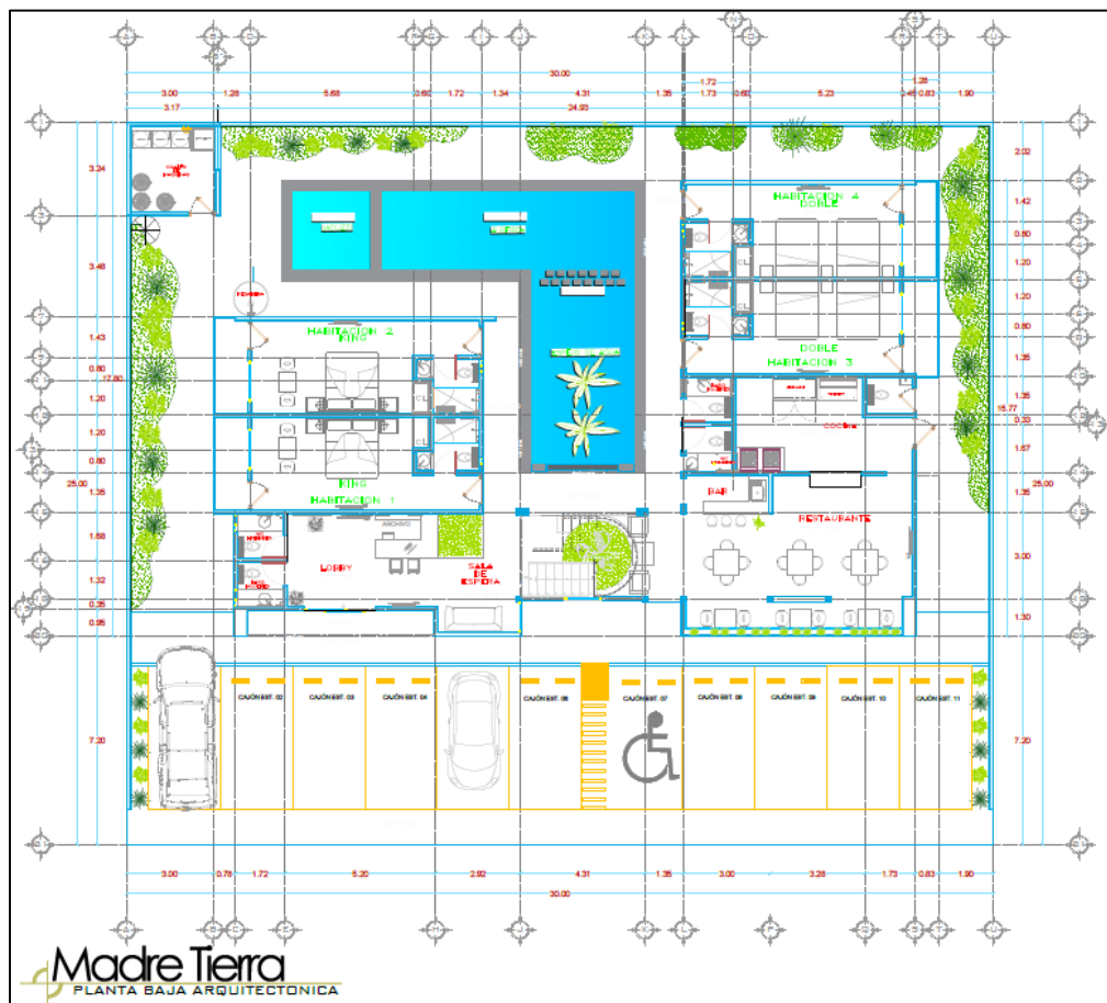
Ilustración II-8. Planta arquitectónica de la planta baja.
