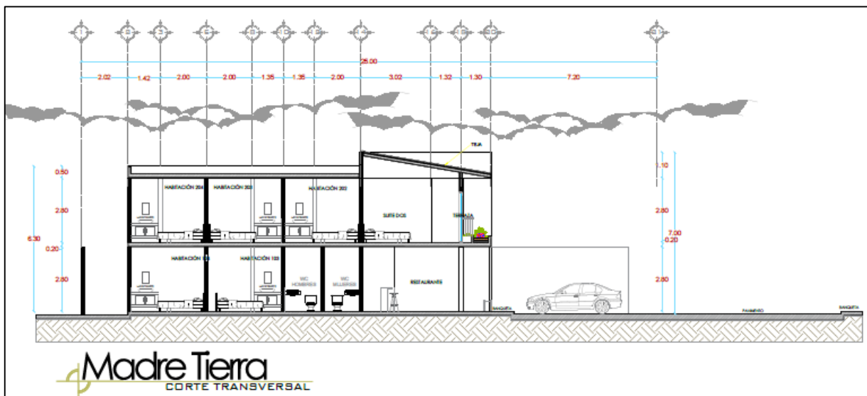
Ilustración II-6. Planta arquitectónica del corte trasversal.
