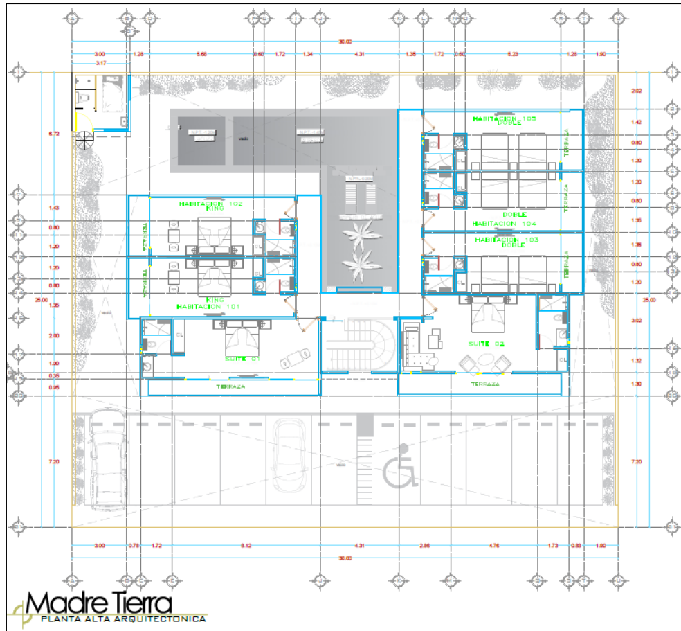
Ilustración II-9. Planta arquitectónica de la planta alta.
