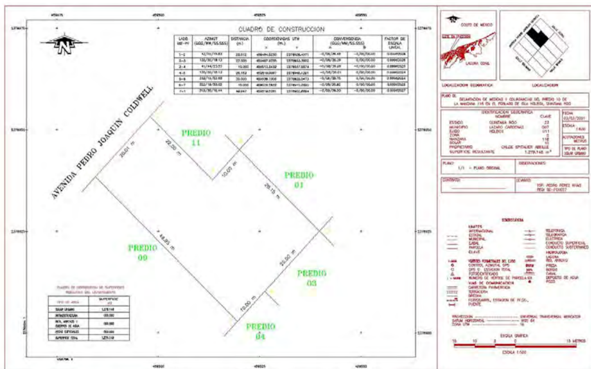
Figura II-2 Levantamiento topográfico Proyecto MESÓN MELABEILLE
