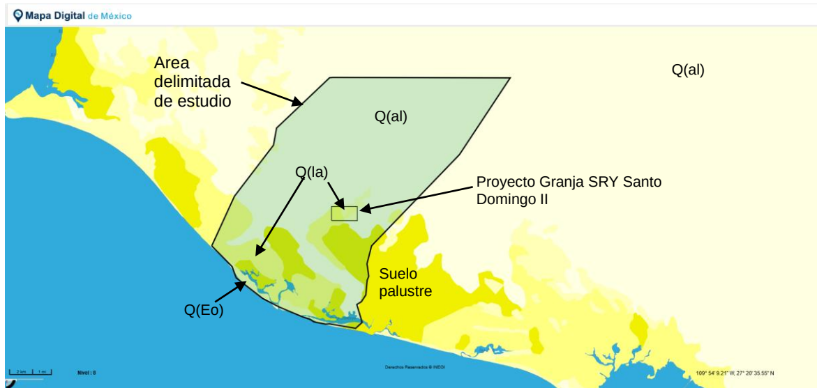
Carta Geológica, delimitación del área de estudio y ubicación del proyecto Granja Acuícola SRY Santo Domingo II.
