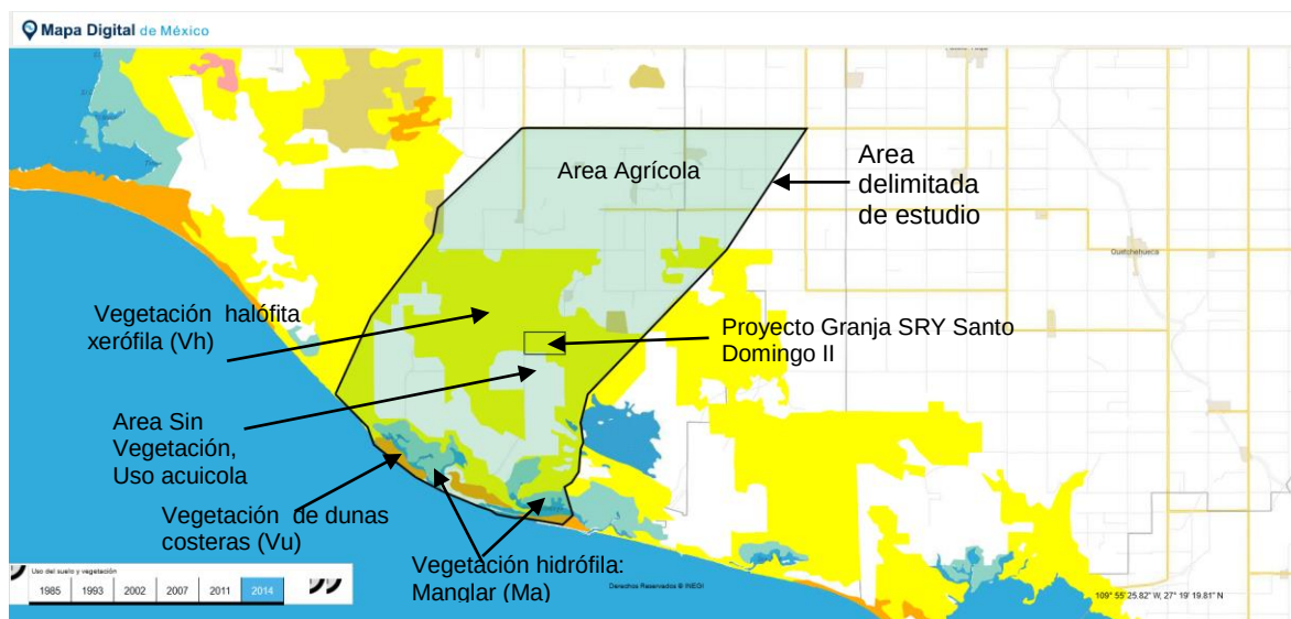
Carta de Uso del suelo y Vegetación, ubicación de la Granja Acuícola SRY Santo Domingo II . INEGI, SERIE VI, 2014.
