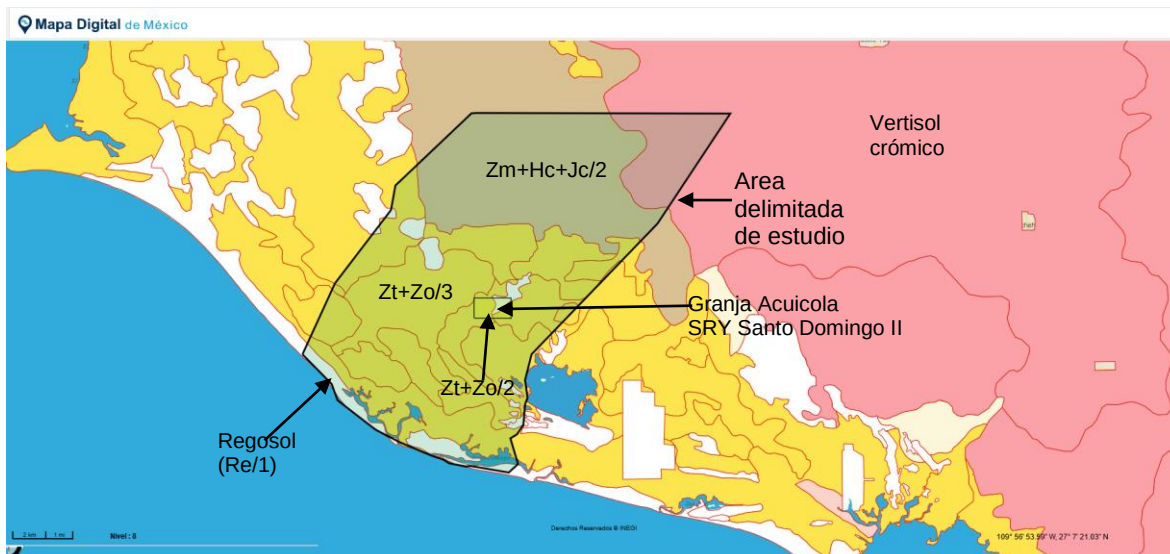
Carta Edafológica y ubicación del proyecto Granja Acuícola SRY Santo Domingo II , para cultivo semiintensivo de camarón blanco.
