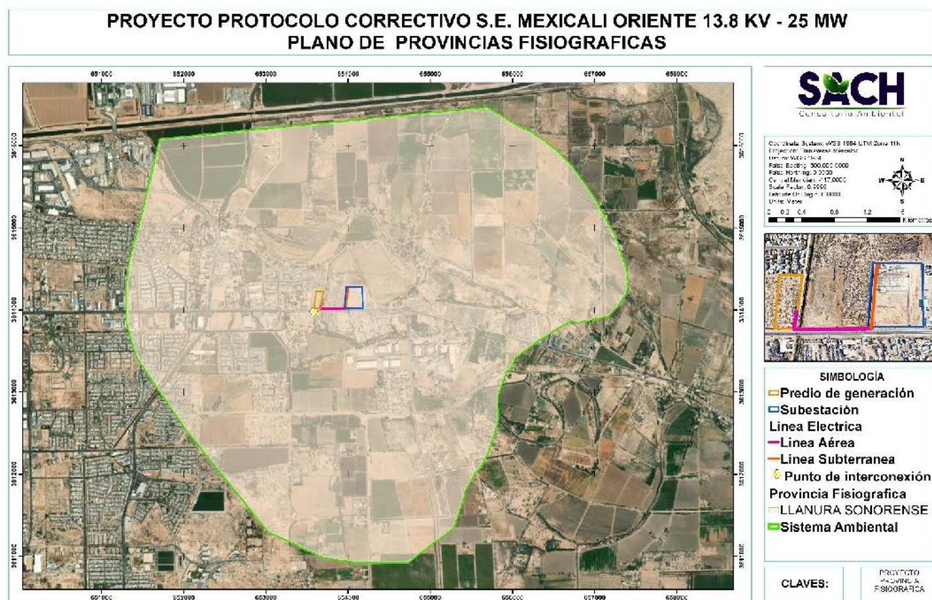
Ilustración 6 Plano de provincias fisiográficas
