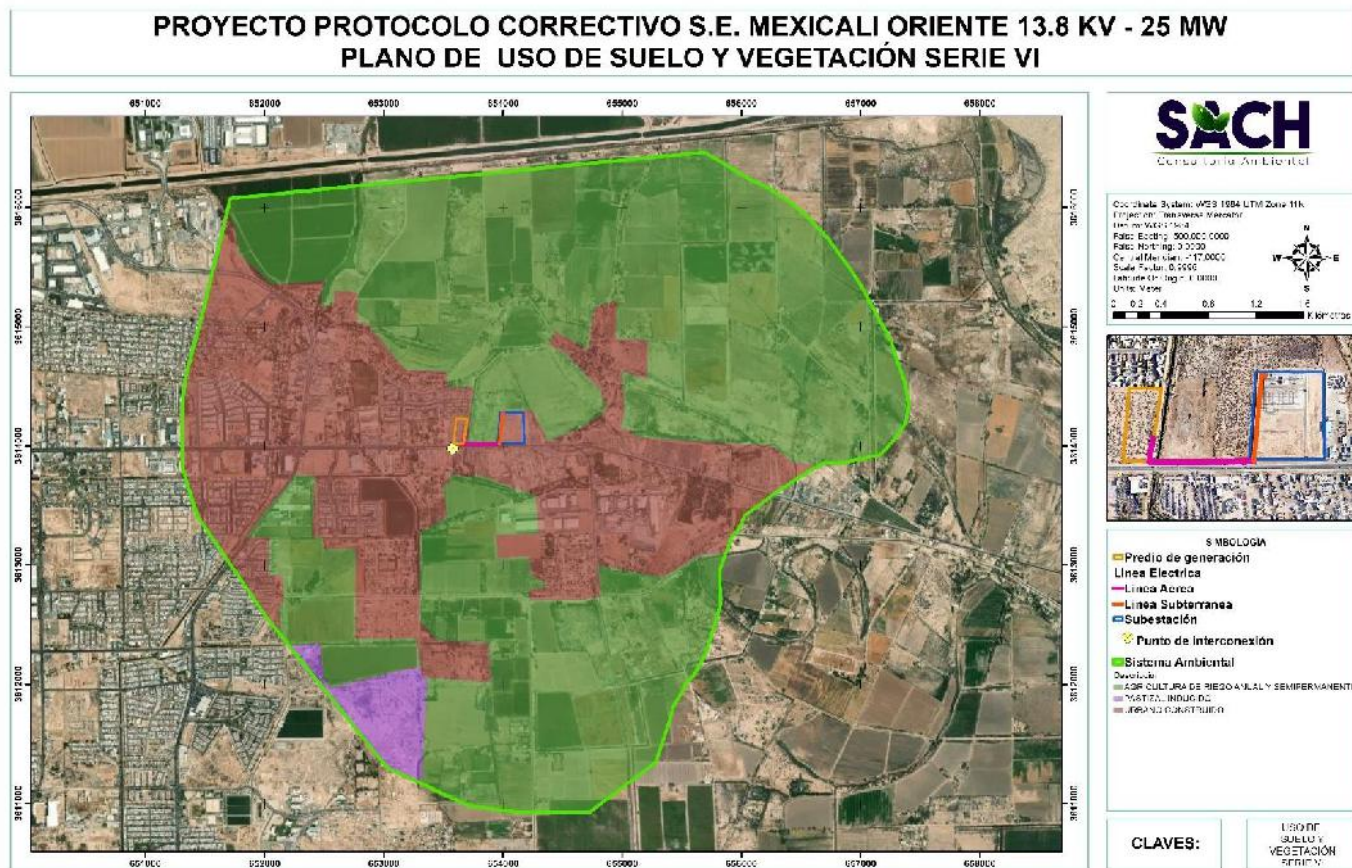
Ilustración 15 Plano de uso de suelo y vegetación serie VI
