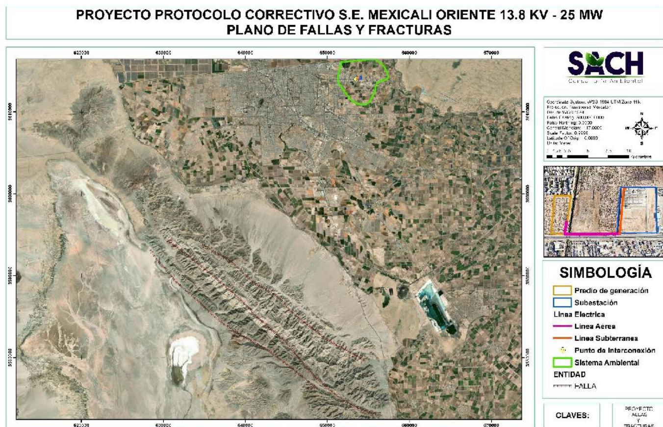
Ilustración 8 Plano de fallas y fracturas
