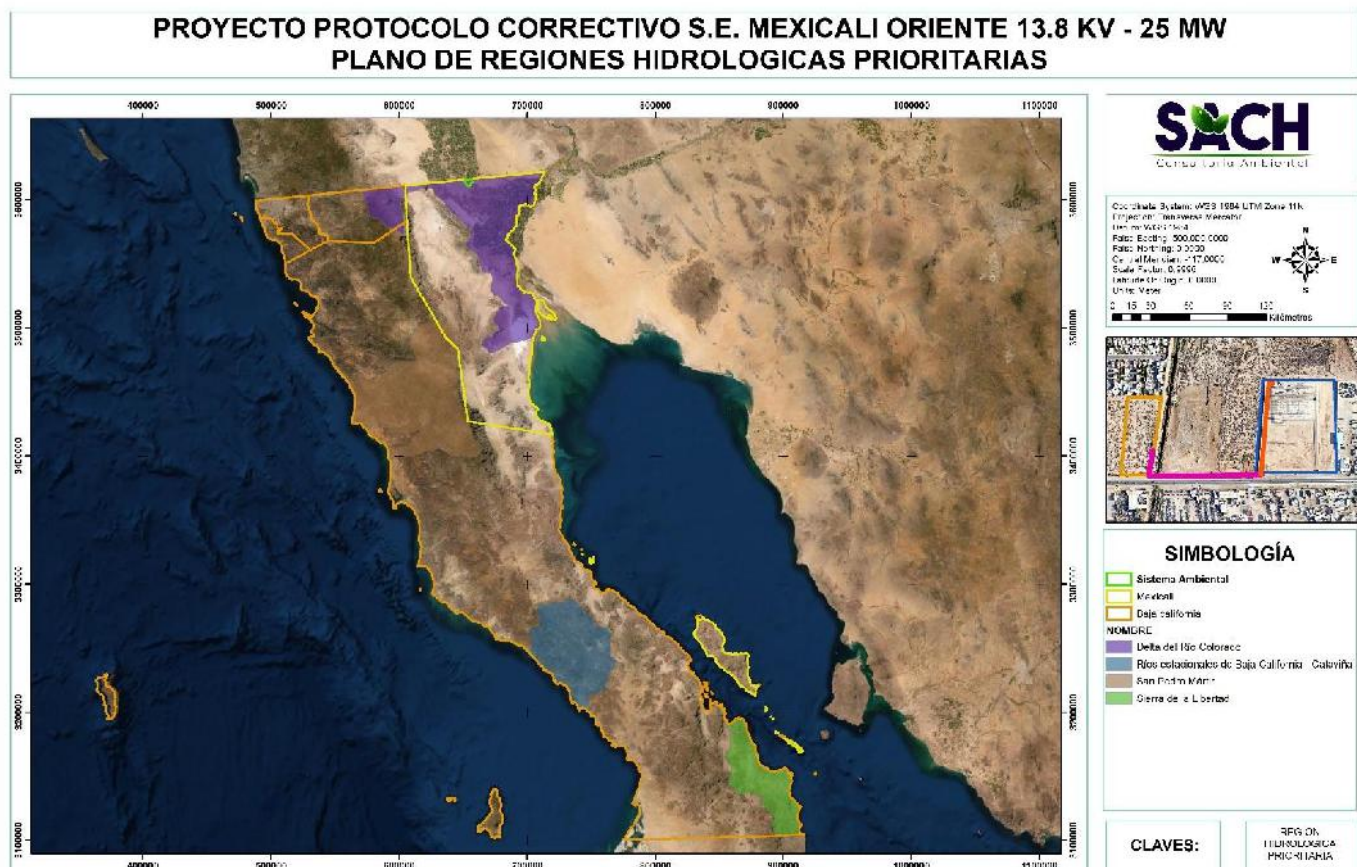
Ilustración 5 Plano de regiones hidrológicas prioritarias
