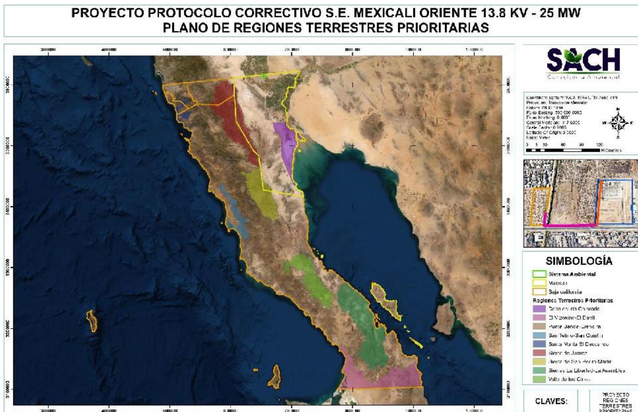
Ilustración 3 Plano de Regiones Terrestres Prioritarias
