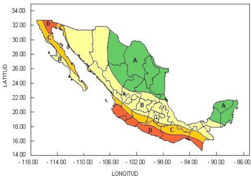
Ilustración 17.- Regionalización sísmica de la República mexicana.
