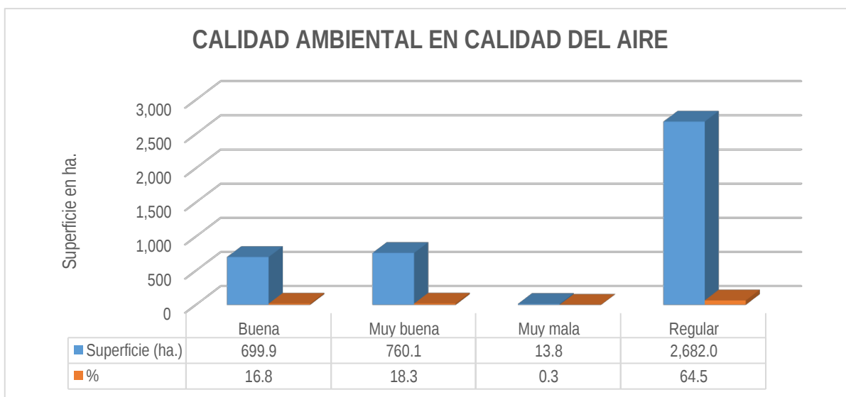
Ilustración 25.- Calidad ambiental en calidad del aire
