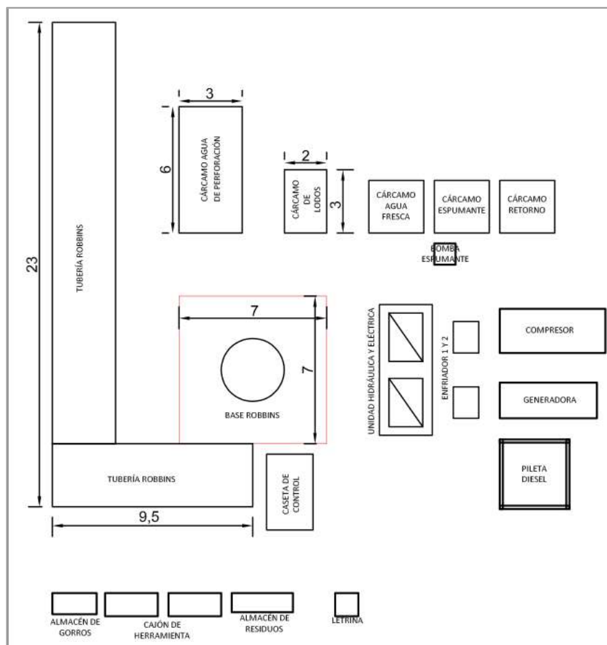
Figura II-3. Arreglo general de un Robbins
