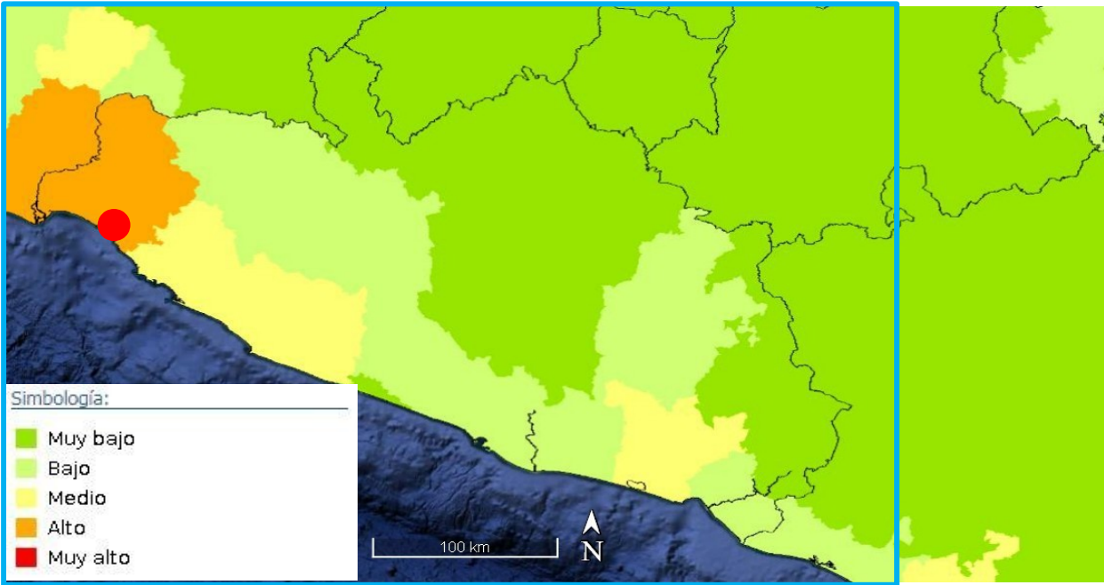
Grado de peligro por presencia de ciclones tropicales
