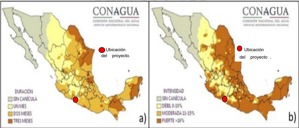
Fig. 2. a) Duración de la canícula en meses, b) Intensidad de la canícula en %. Para el cálculo de los mapas se utilizó información disponible de 985 estaciones en el periodo mayo-septiembre de 2014 en el Sistema de Información Hidroclimatológica (SIH) de la Gerencia de Aguas Superficiales e Ingeniería de Ríos-Conagua, cualquier cálculo posterior podrá resultar diferente.
