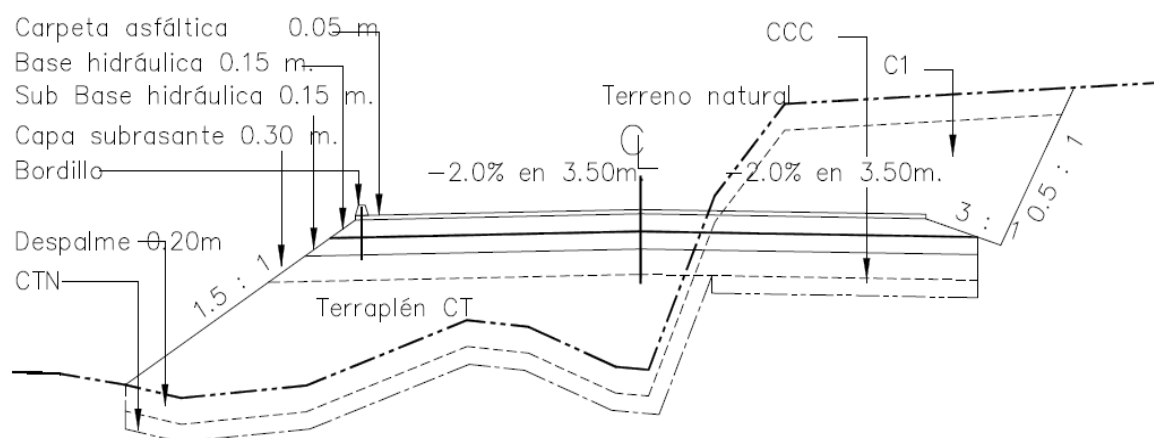
Imagen 10. Secciones tipo del camino a pavimentar.
