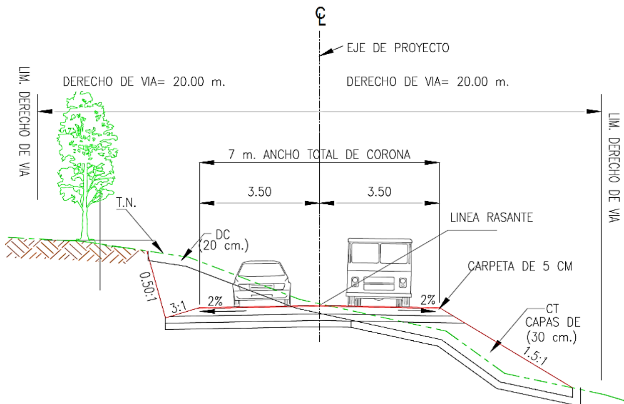
Imagen 1. Sección tipo del proyecto de pavimentación del camino.
