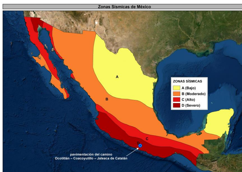
Imagen 37: Zonas Sísmicas de México, INEGI, 2005.
