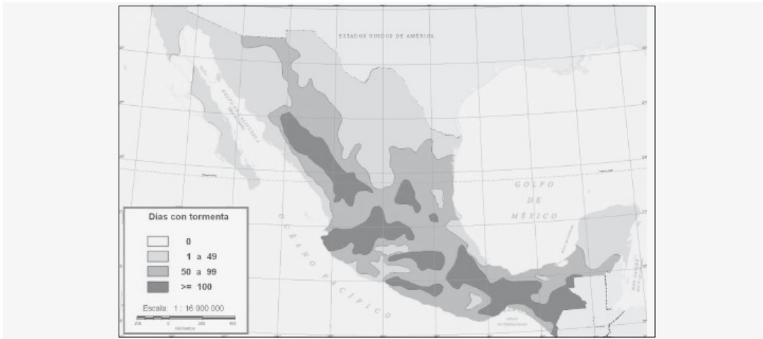
Imagen 11 Máximo anual de días con tormenta eléctrica en México. FUENTE: CENAPREV. SEGOB. 2010
