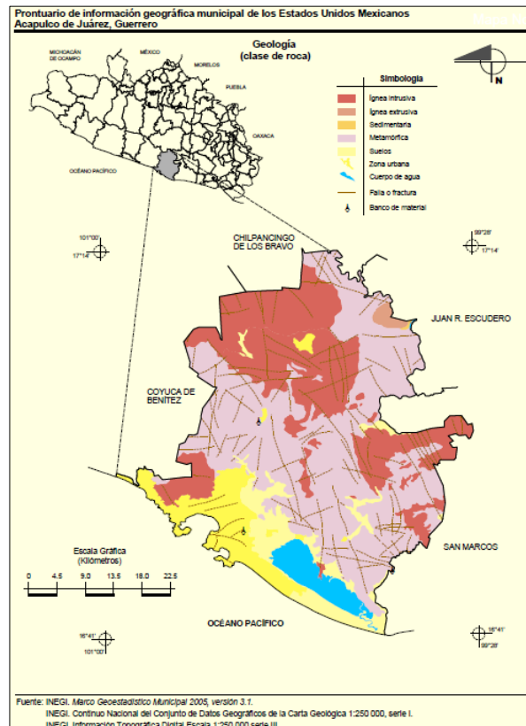
Imagen 9 Carta geológica INEGI
