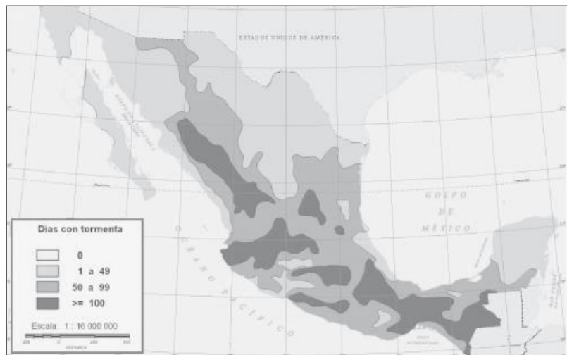
Imagen 8 Máximo anual de días con tormenta eléctrica en México. 2010
