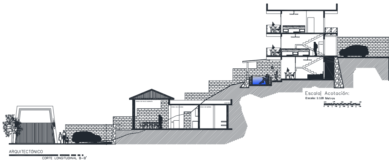
Imagen 02. Refiere un perfil general del proyecto que se pretende llevar a cabo al interior del lote. (Para mayor detalle en su distribución, dimensiones y escala, ver planos impresos y digitalizados anexos).
