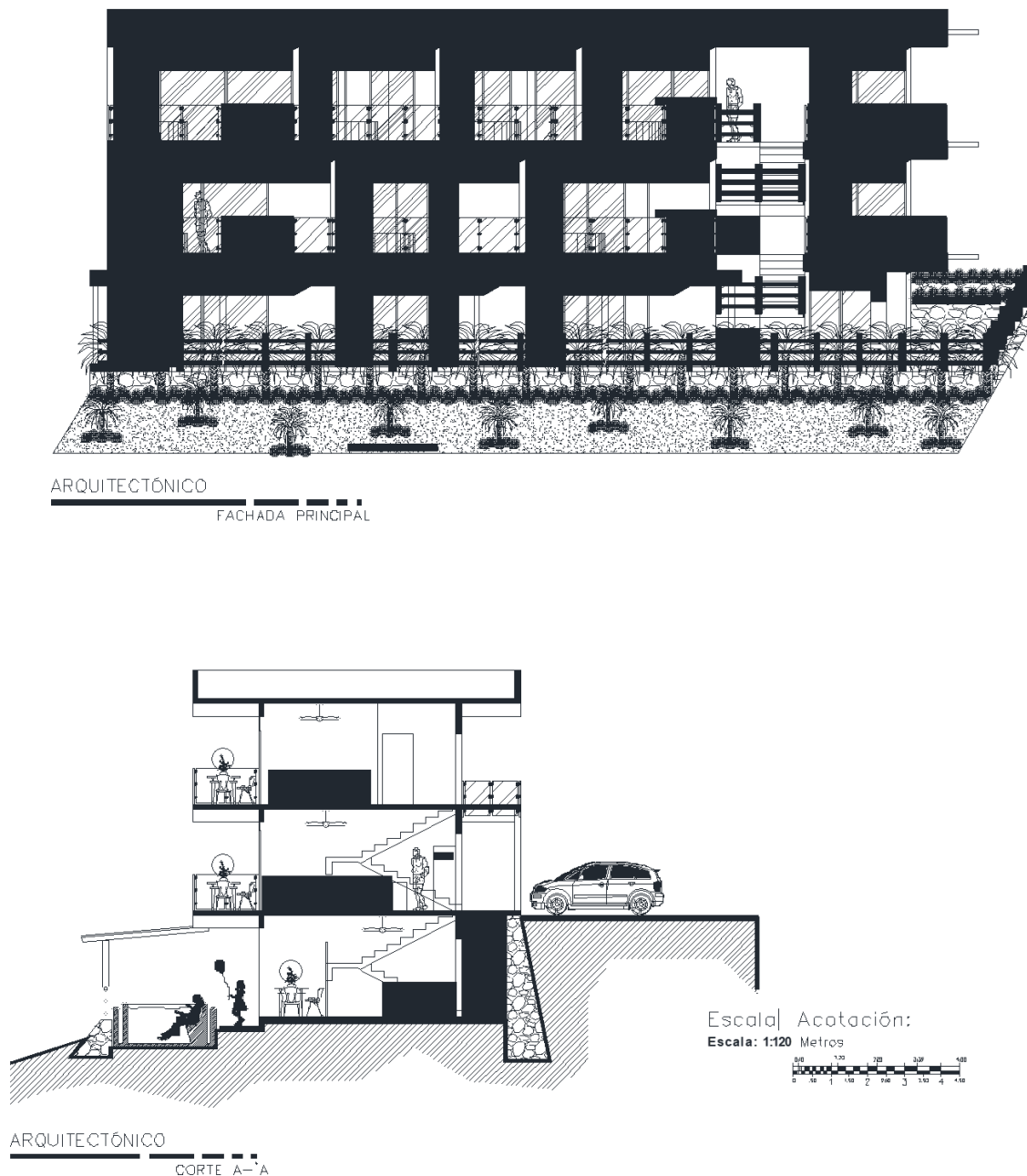
Imagen 03. Refiere la fachada principal y el corte arquitectónico que permiten constatar una visión general del tipo de proyecto que se llevara a cabo al interior del lote. (Para mayor detalle en su distribución, dimensiones y escala, ver planos impresos y digitalizados anexos)
